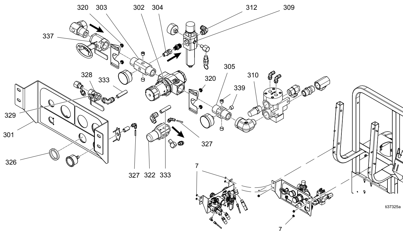
FIG. 1 Comandi pneumatici
