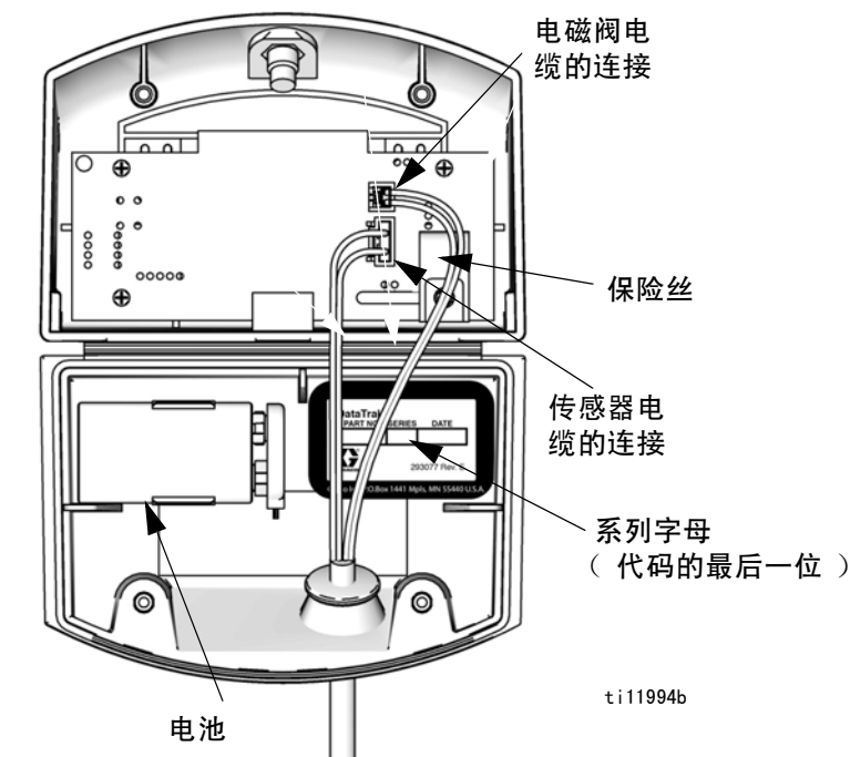
图 4。DataTrak 电池和保险丝的位置
