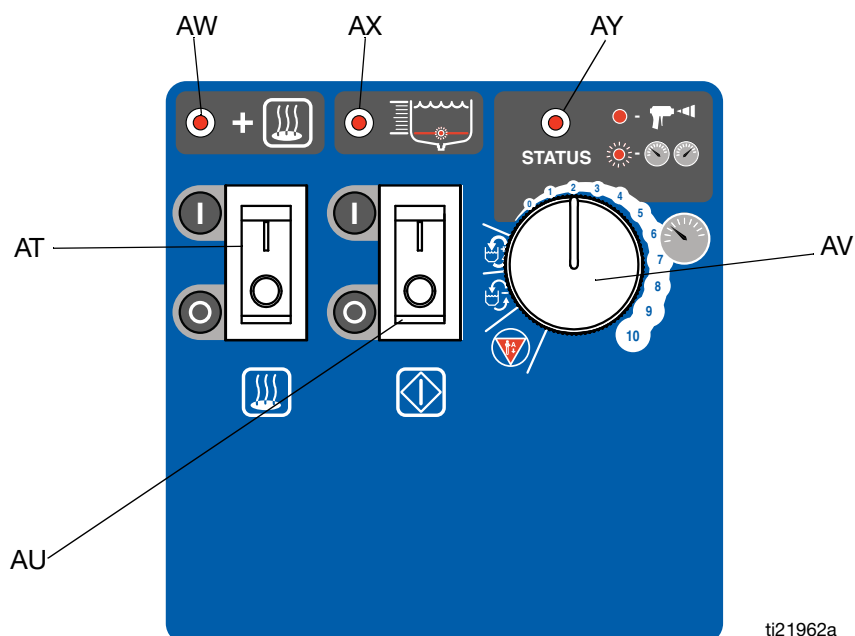
FIG. 3 Systemregla och -indikatorer
