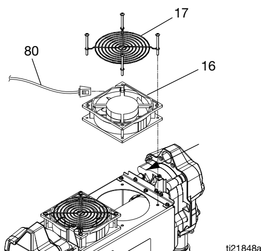
FIG. 20 Fläktar
