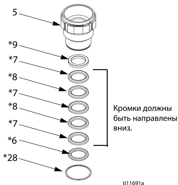
Рис. 3. Замена уплотнений горловины
