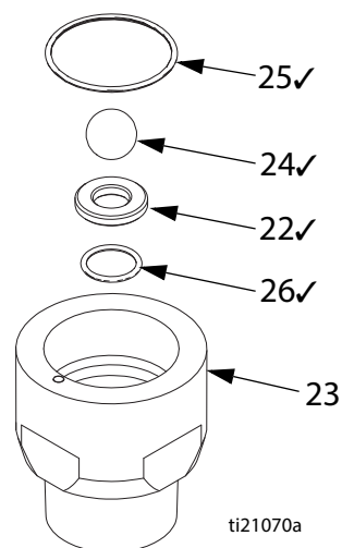
Рис. 7. Замените впускной шар и седло.
