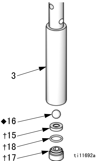
图 5. 更换活塞球和基座。
