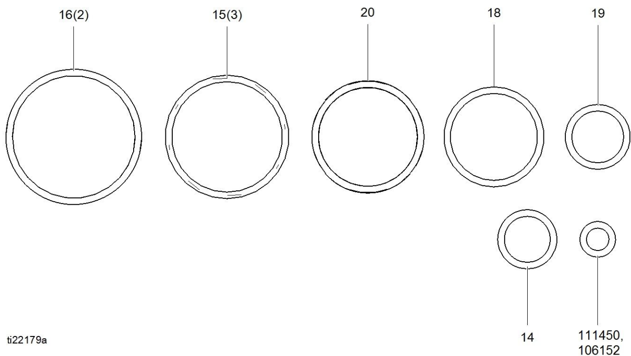
Figure 4 Rozmiary uszczelki okrągłych z zestawu 24T848 i 24Y671
