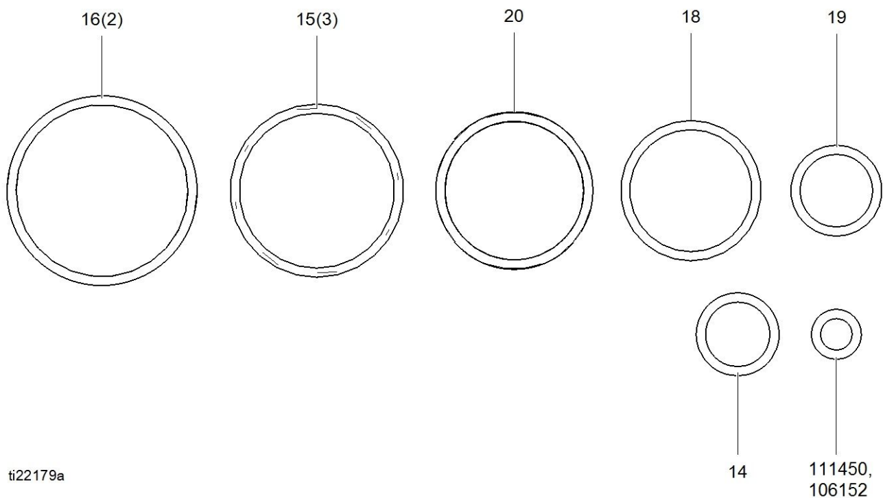
Figure 4 Kit 24T848 et Kit 24Y671 Tailles de joint torique
