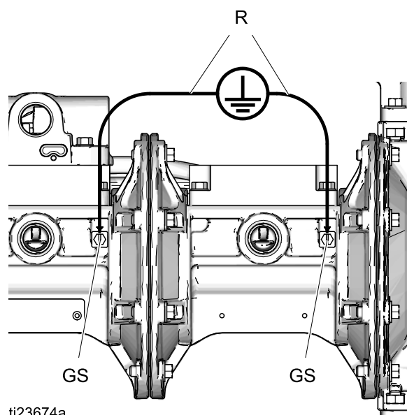
Figure 1 Jordningsskruvar och -ledningar
