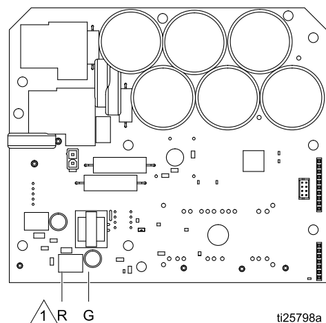
Figure 12 Placa de alimentación
