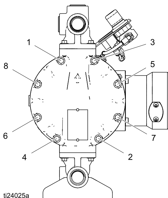
Tornillos de la tapa de fluido
