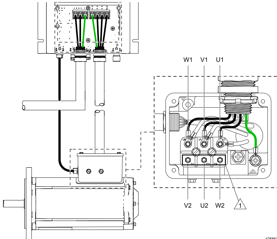
Figure 9 Cableado al motor
