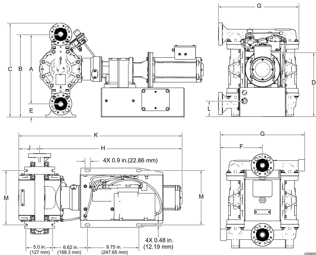
Figure 16 Bombas con secciones de fluido de polipropileno, polipropileno conductor o PVDF, con compresor (mostrado modelo BLDC)
