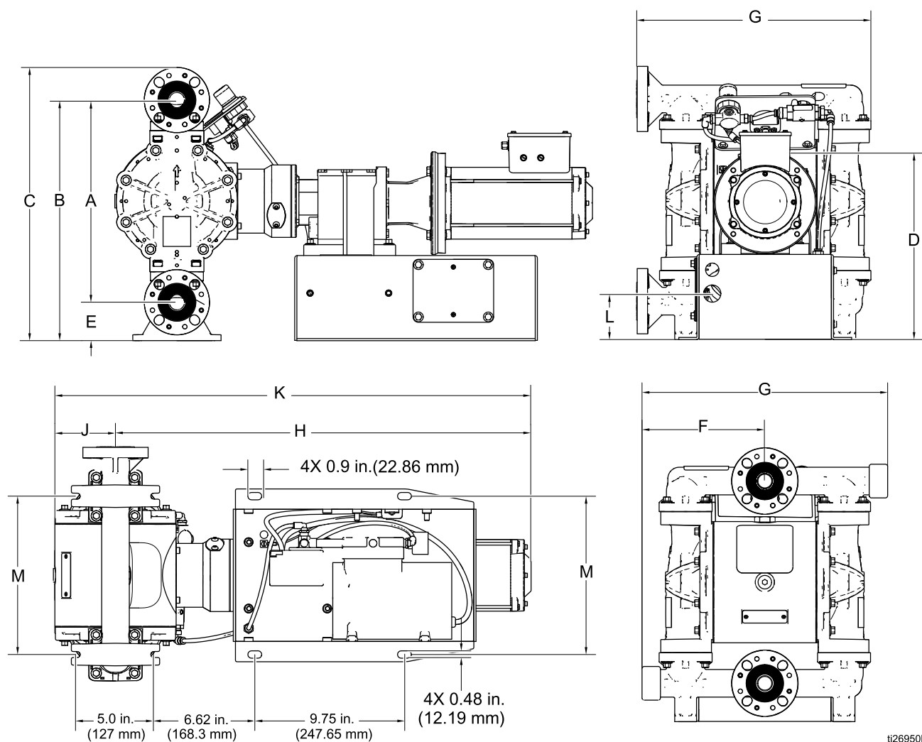
Figure 16 Насосы с жидкостными секциями из полипропилена, токопроводящего полипропилена или поливинилиденфторида (PVDF), с компрессором (показана модель с бесщеточным электродвигателем постоянного тока)
