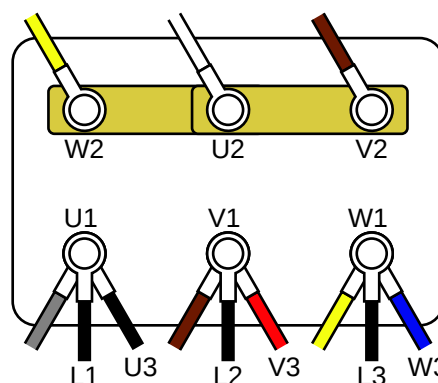
Figure 4 Соединения для электропроводки на 230 В
