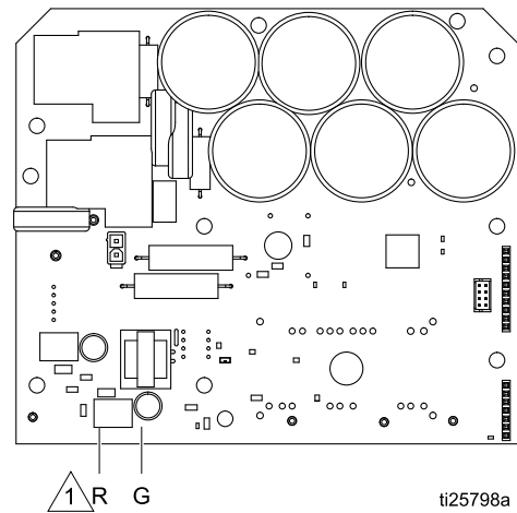
Figure 12 전원 보드
