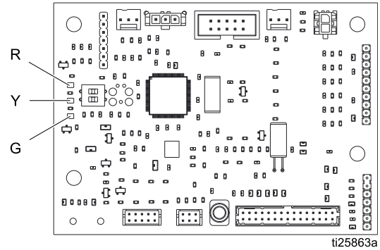
Figure 11 제어 보드
