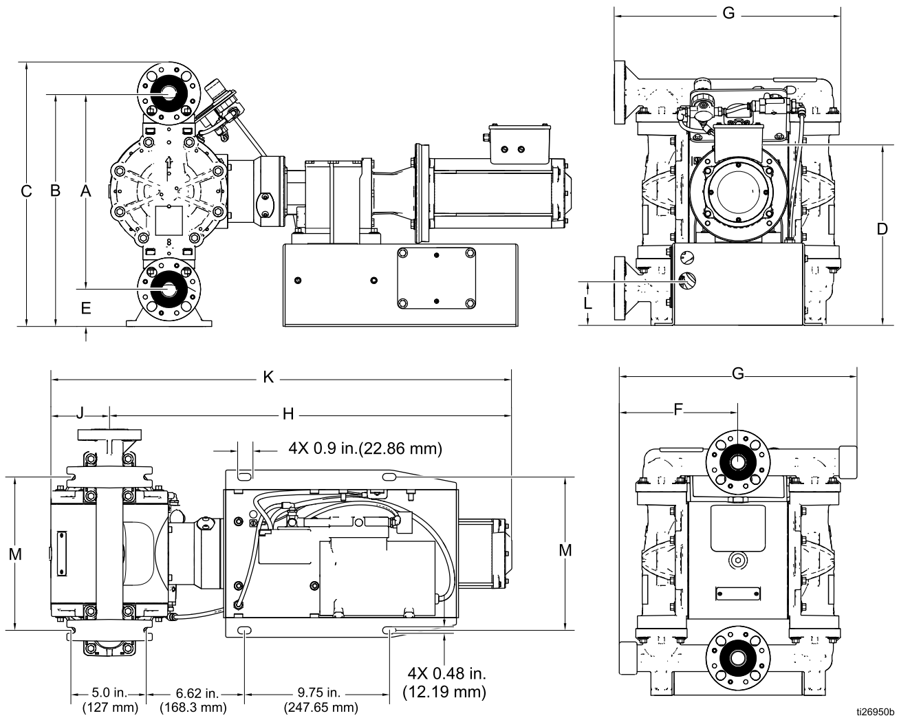
Figure 16 폴리프로필렌, 전도성 폴리프로필렌 또는 PVDF 유체 섹션이 있는 펌프, 압축기 포함(그림은 BLDC 모델임)
