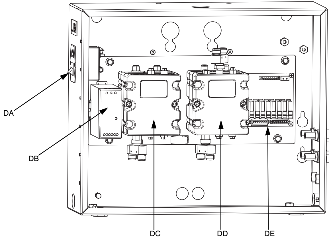
FIG. 8: Armario eléctrico
