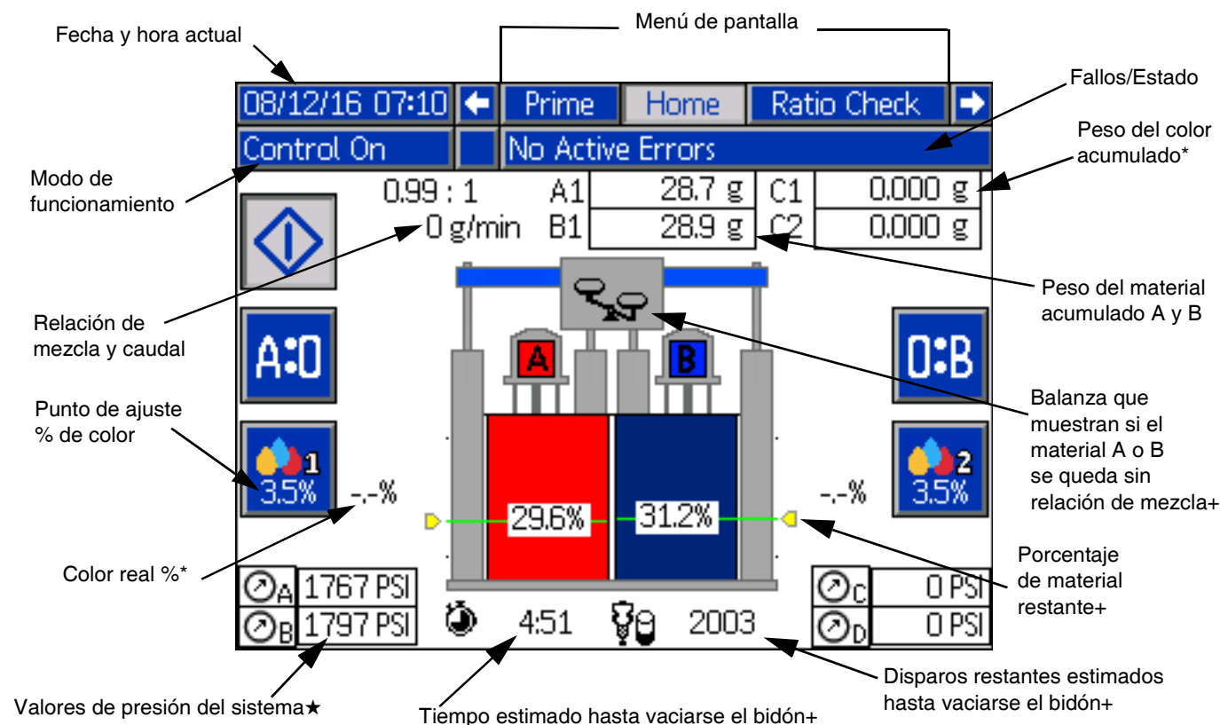
Fig. 5: Componentes de la pantalla de inicio del ADM
