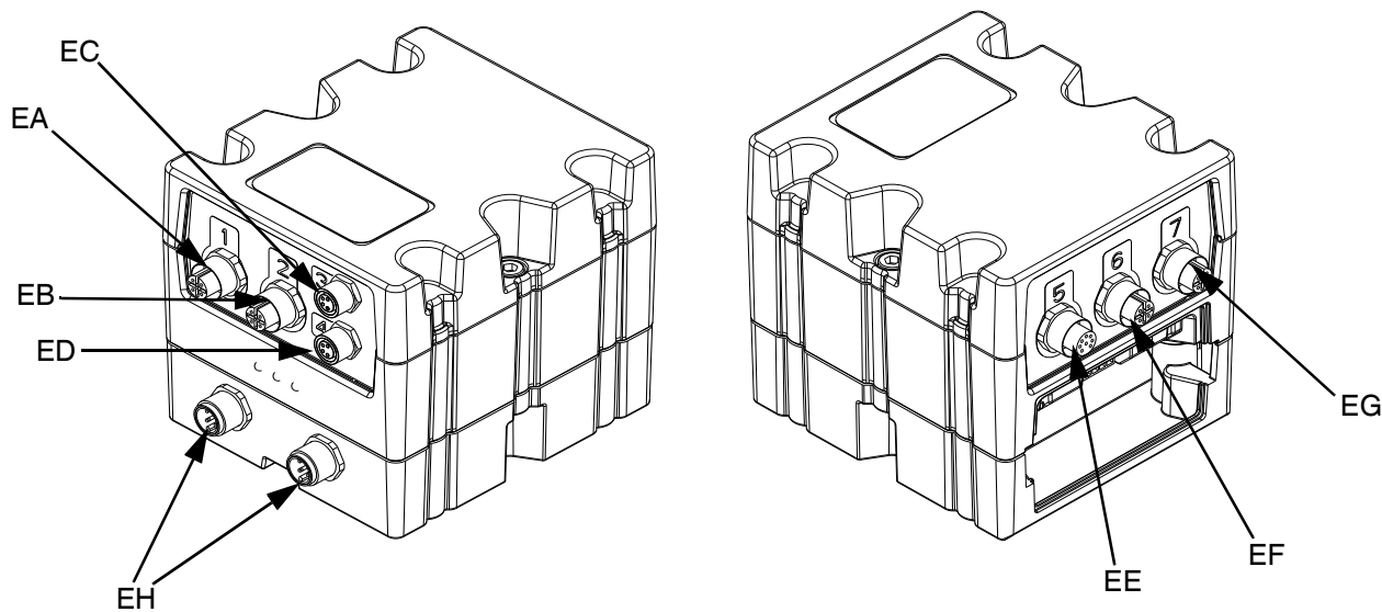
FIG. 9: Conexiones de FCM 1 y 2
