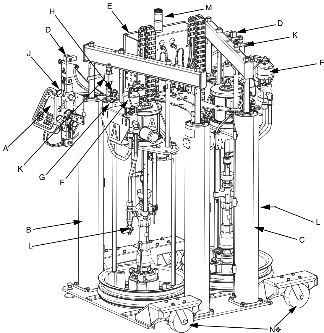
FIG. 2: Modelo F4-55
