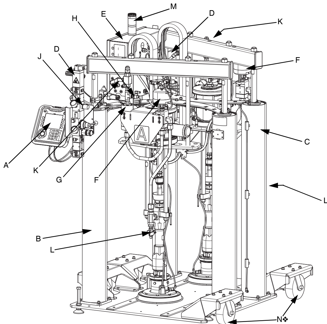
FIG. 3: Modelo F4-55-5
