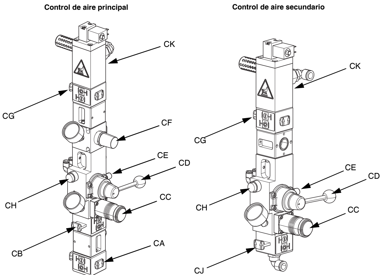
FIG. 7: Controles de aire integrados
