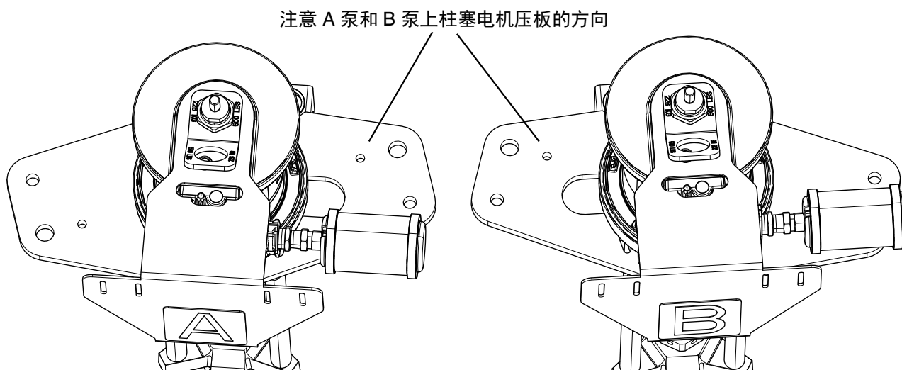
图 19: A 和 B 泵压板对齐
