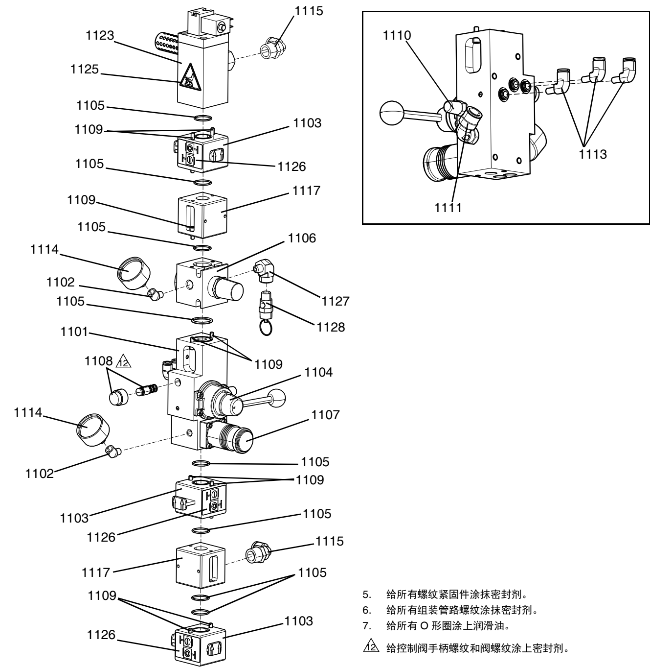
图 16主集成气流控制
