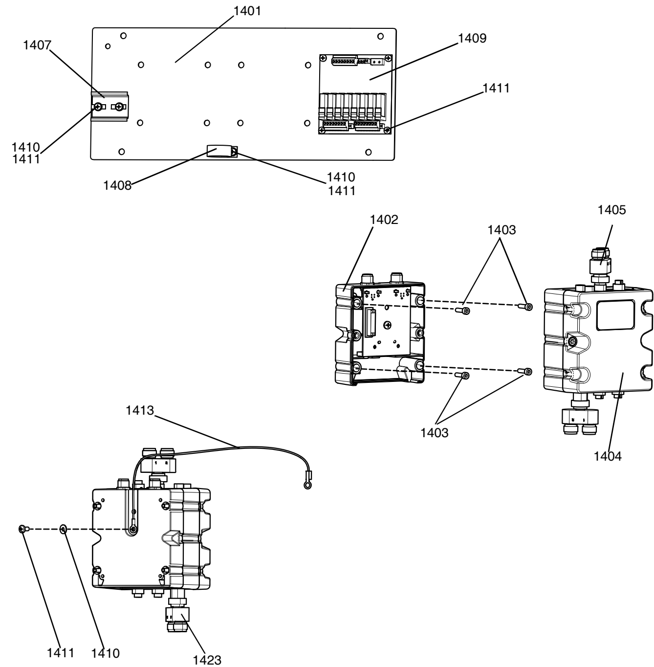
图 15 显示了电子外壳的控制面板和流体控制模块（FCM）的零件。
