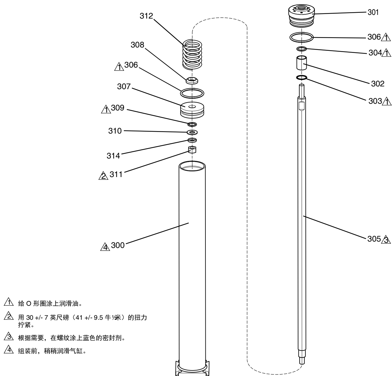
图 4: F4-5 柱塞气缸
