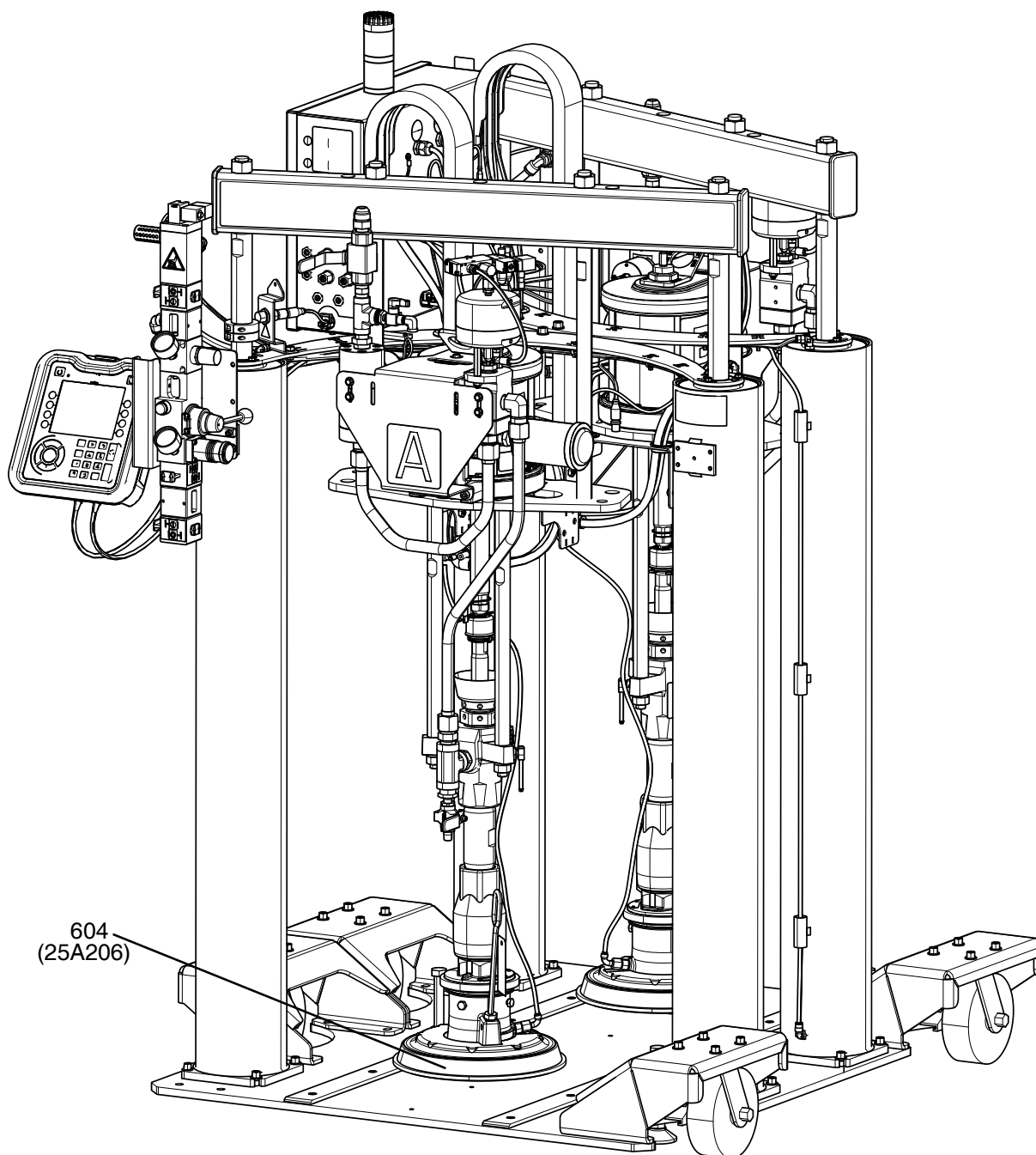
图 12: F4-55-5 型号, 24X166 带脚轮
