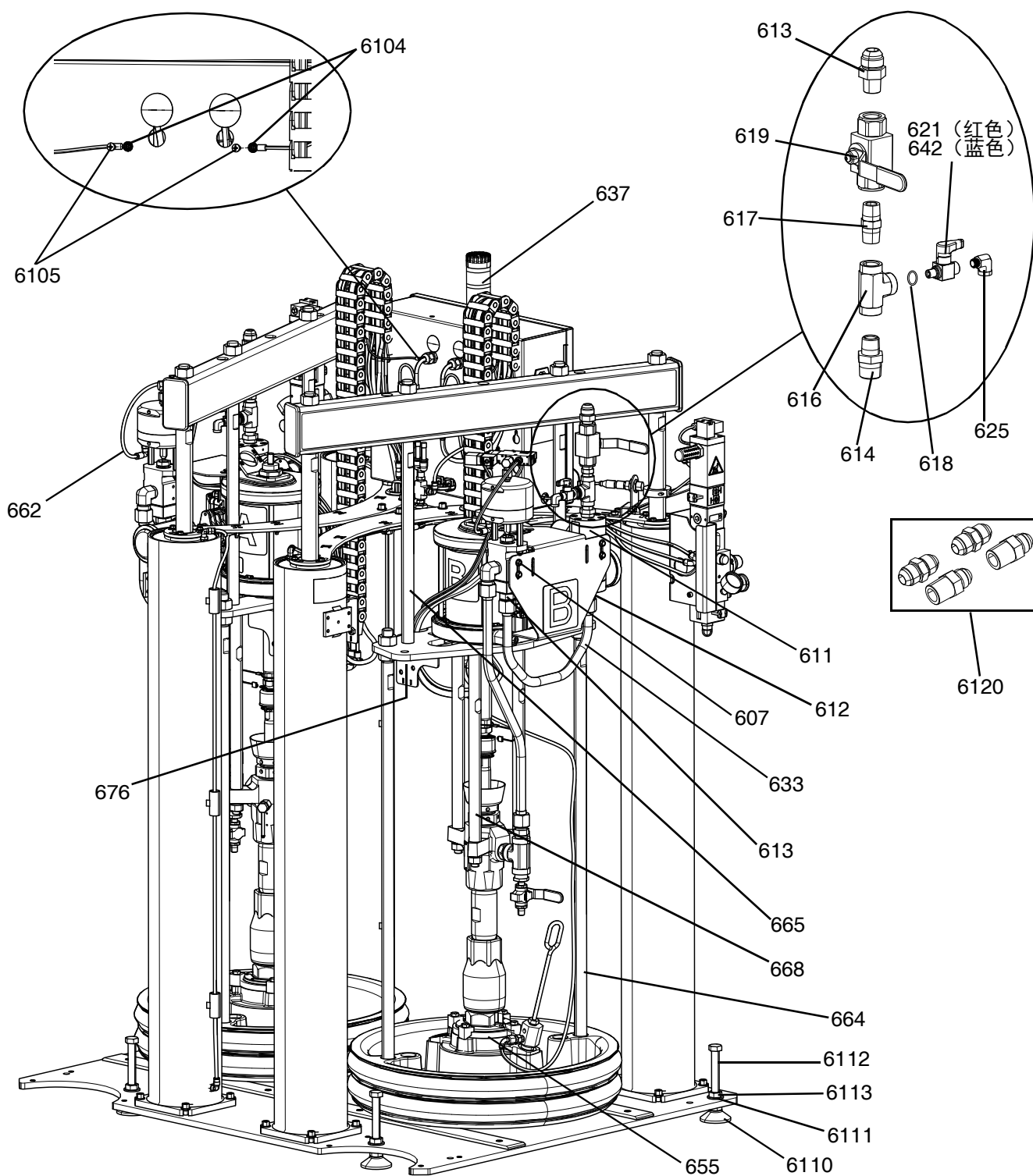
图 8: F4-55 型号, 24X169 不带脚轮 - 视图 2
