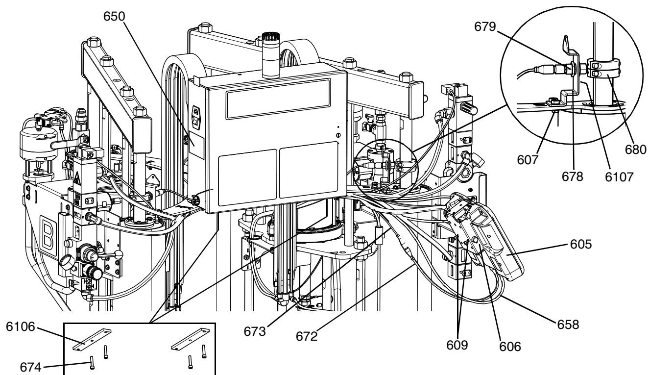
图 9: F4-55 型号 - 视图 3
