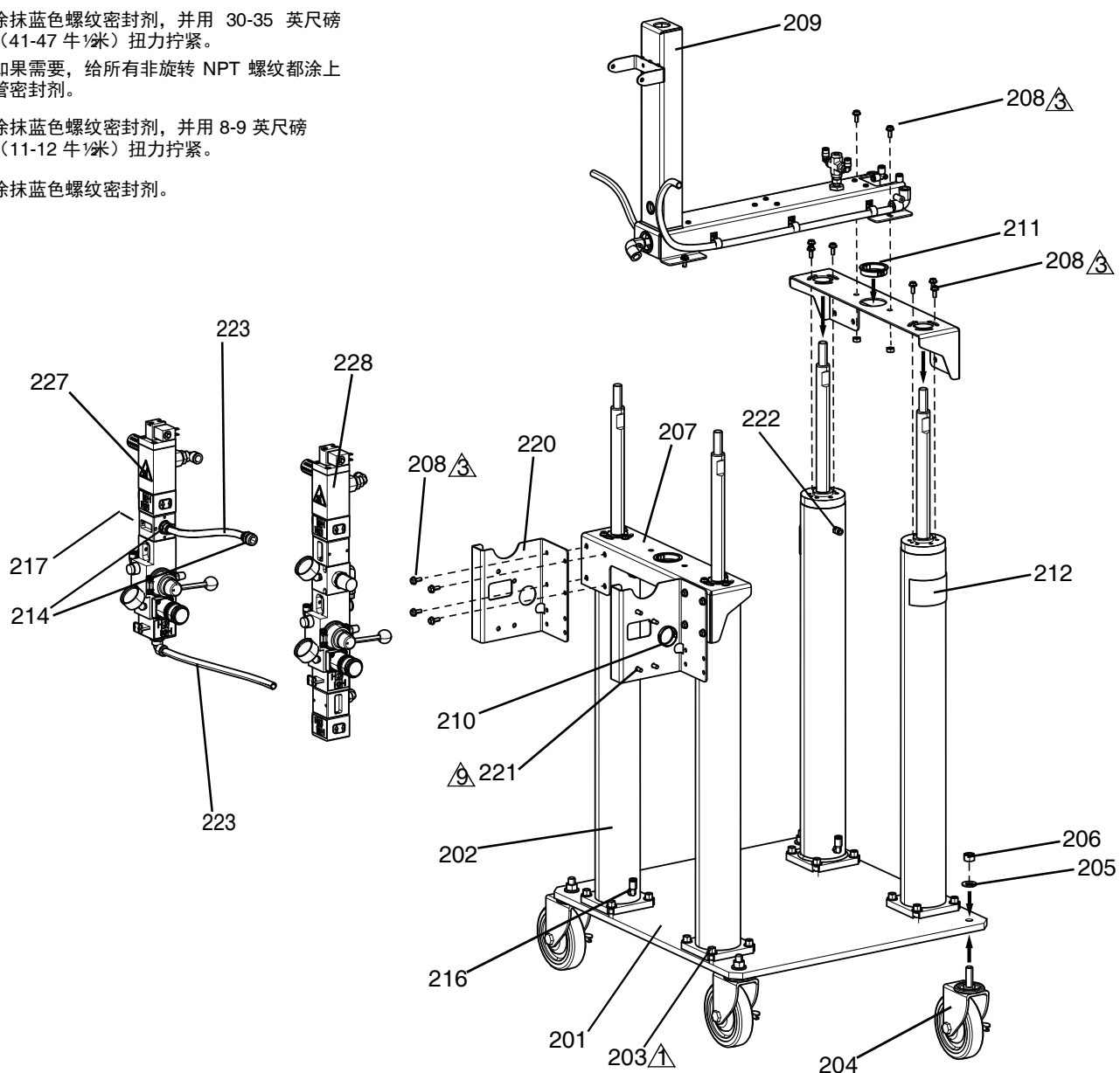
图 3: F4-5 底座 - 柱塞, 双列
