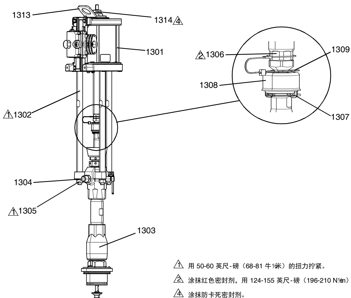
图 20: 泵组件套件
