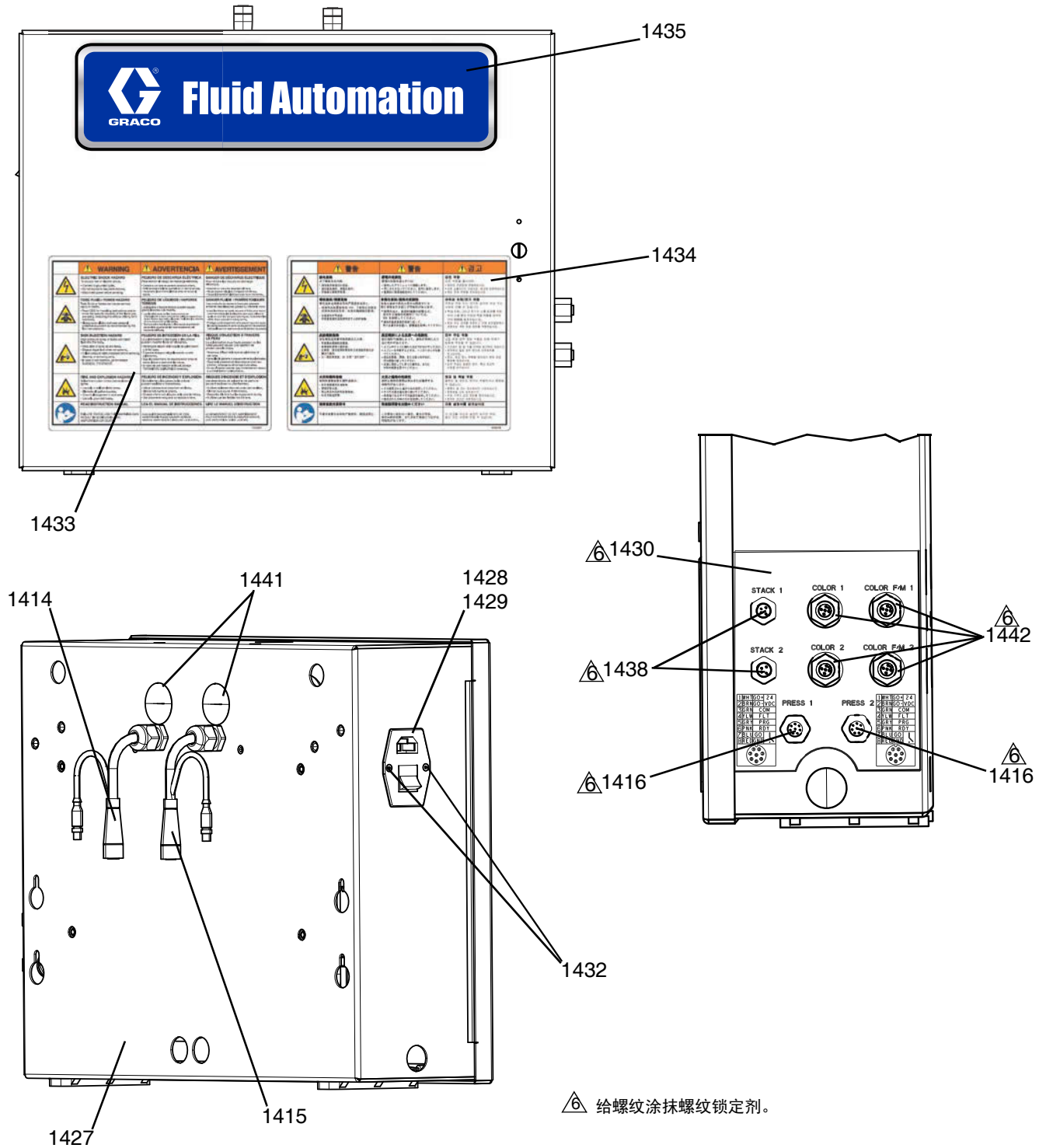
图 23: 电子柜 - 外部
