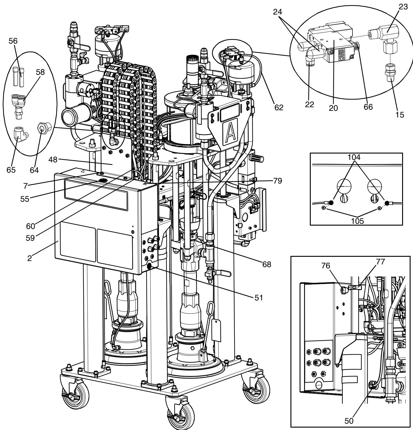
图 2: F4-5 模型后视图
