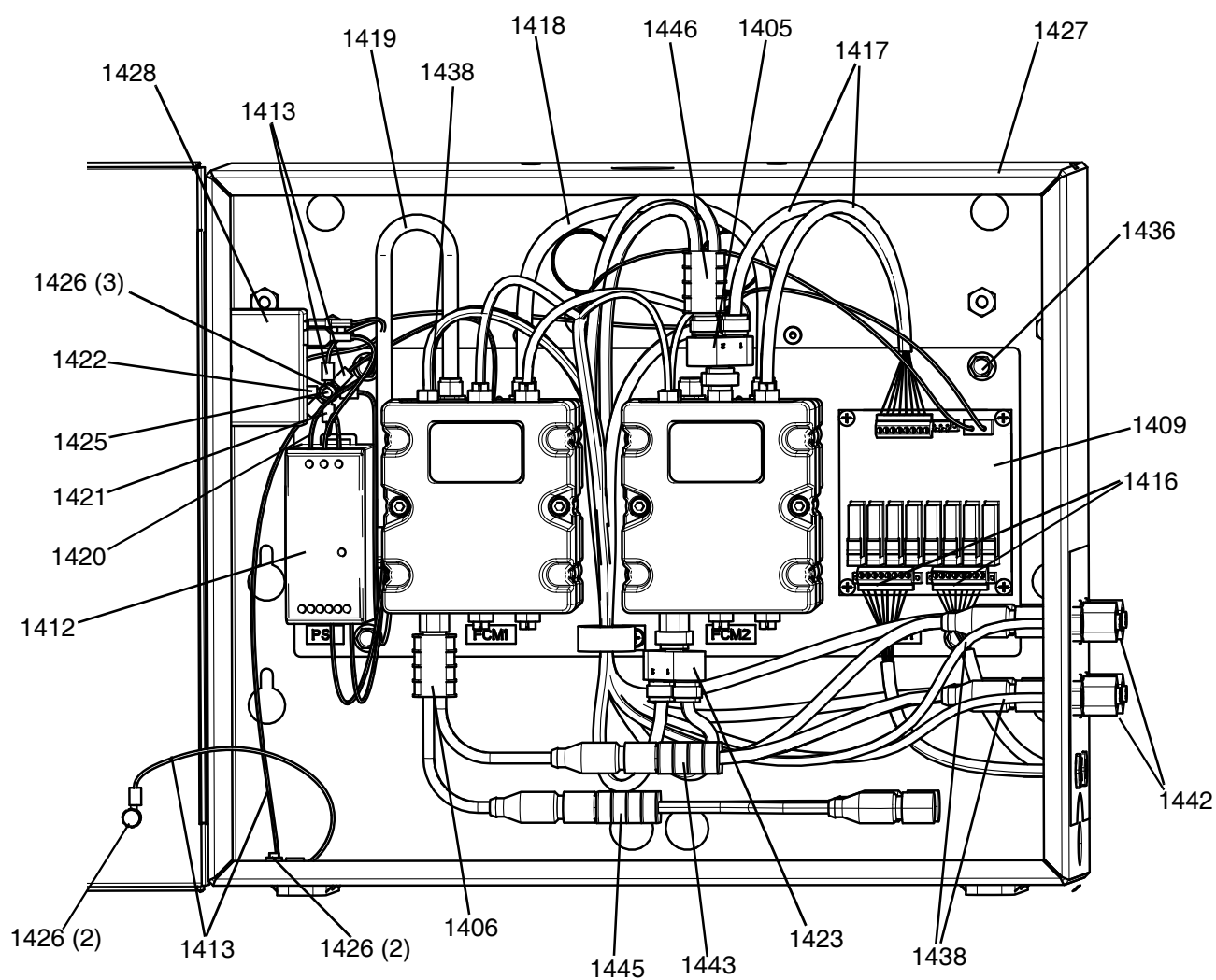
图 21：电子柜 - 内部
