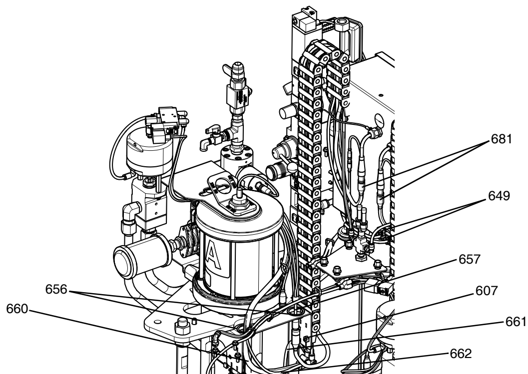
图 10: F4-55 型号 - 视图 4
