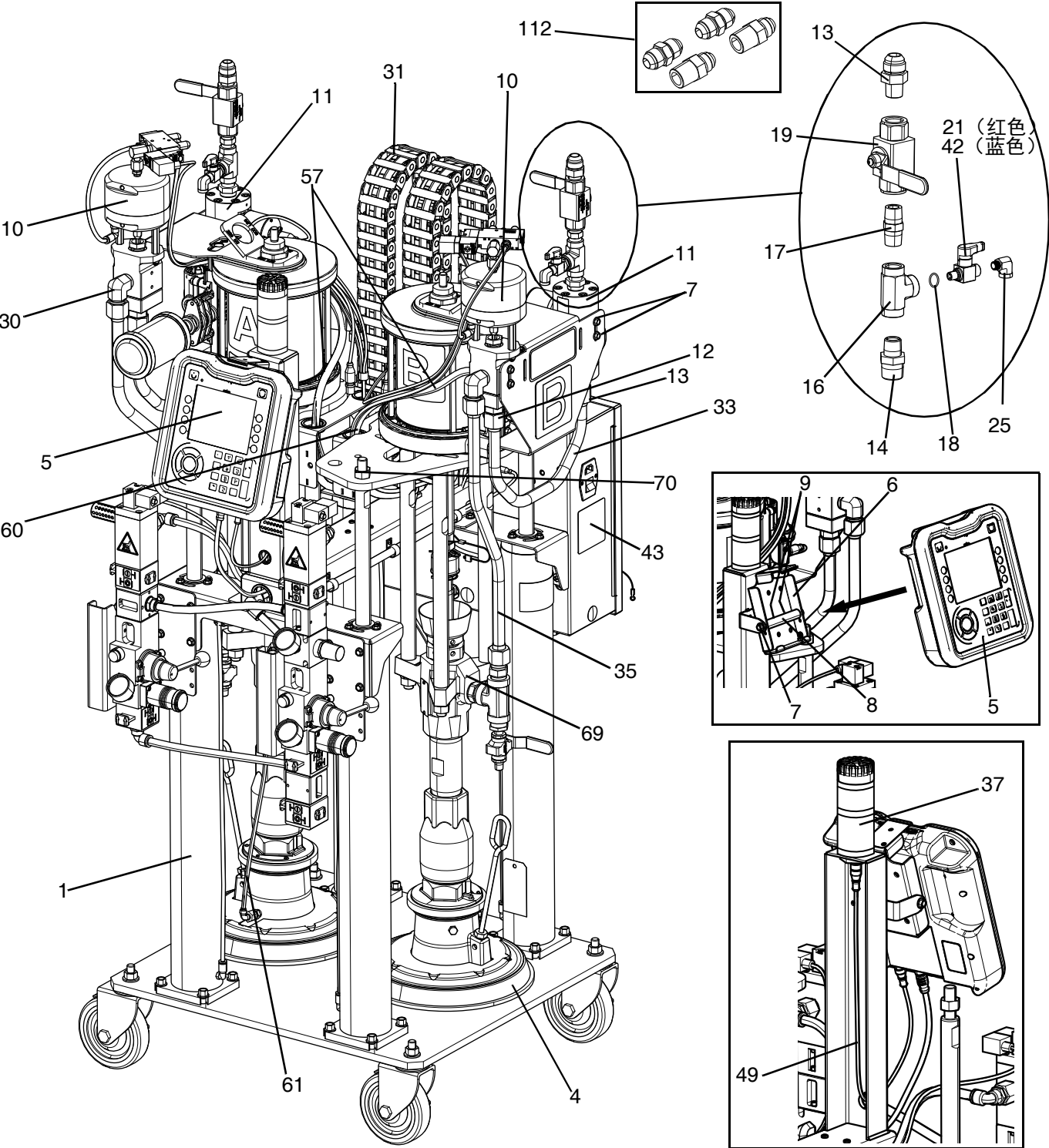
图 1: F4-5 模型前视图
