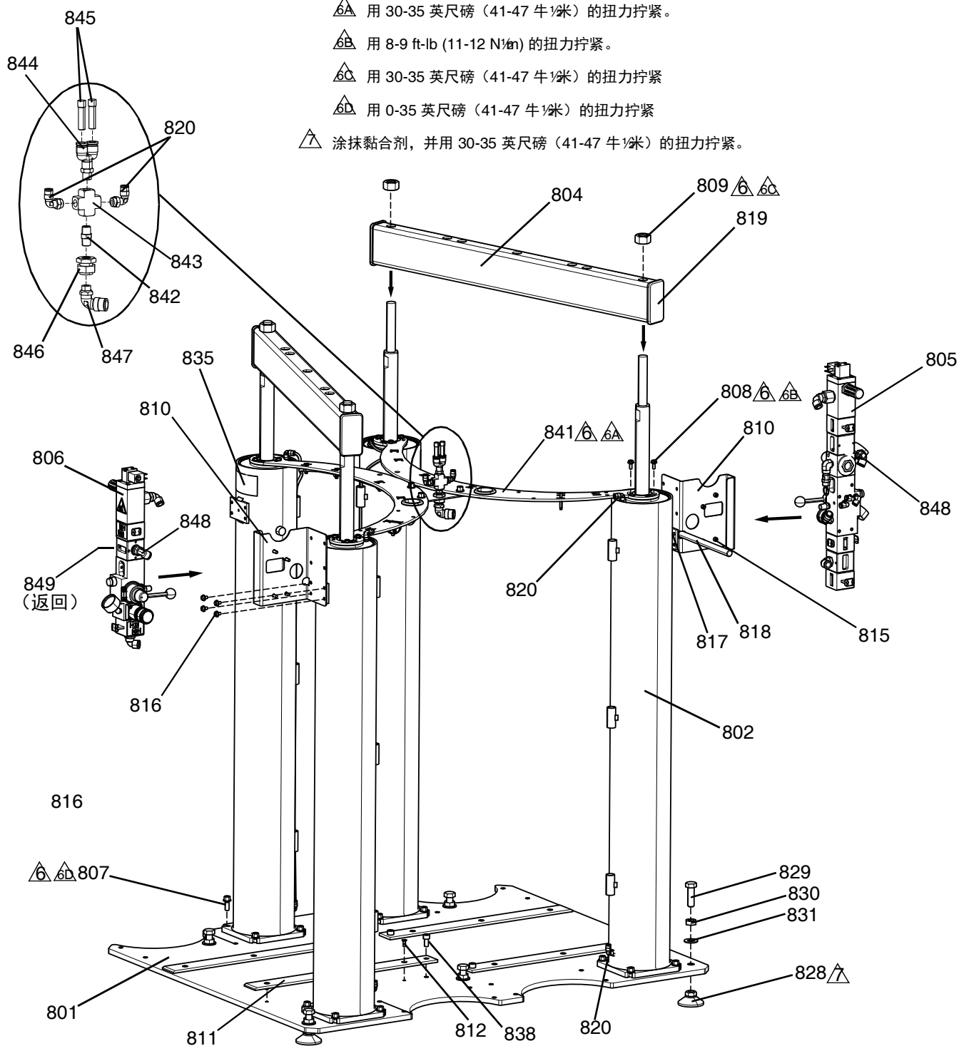
图 13: F4-55 底座 - 柱塞, 双列
