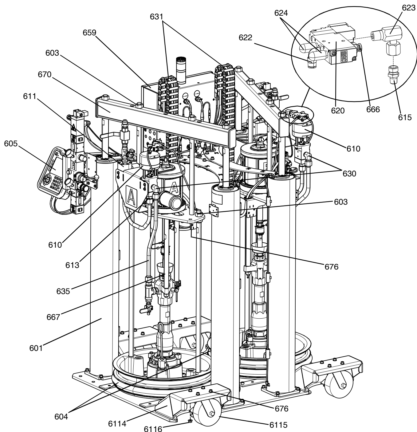
图 7: F4-55 型号, 24X167 带脚轮 - 视图 1
