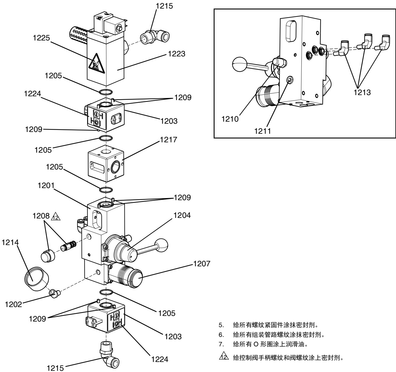
图 17：辅助集成空气控制器
