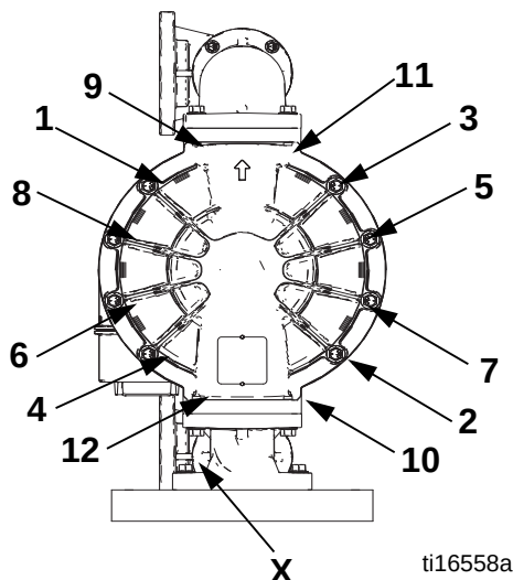
FIG. 5. Instrucciones de apriete, sujetadores de las cubiertas de fluido y de la válvula de aire (todos los modelos, se representa el de aluminio)
