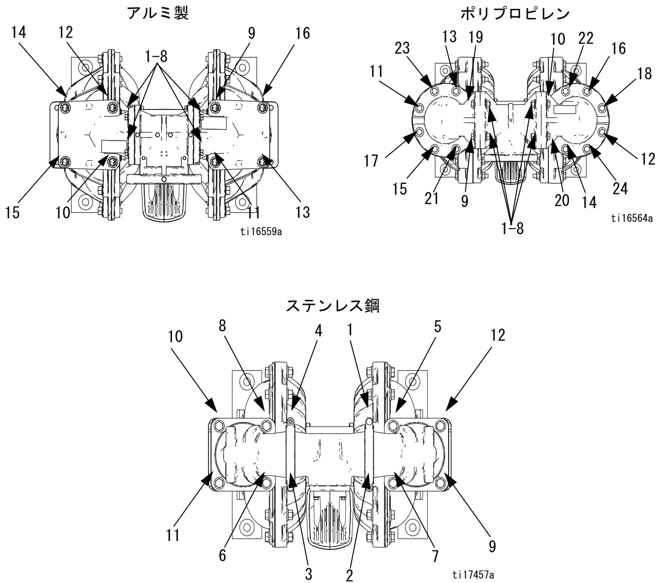
図 6. トルクの手順 - マニホールドファスナー
