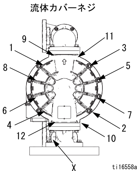
図 5. トルクの手順、液体カバーとエアバルブファスナー（全モデル、アルミニウム製を表示）
