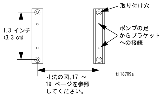
図 2. 取り付け図
