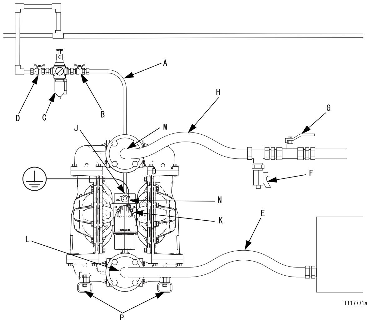
図1. 一般的な取り付け（アルミニウム製ポンプ）
