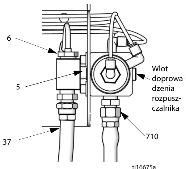
Rys. 21. Odłączyć przewody cieczy
