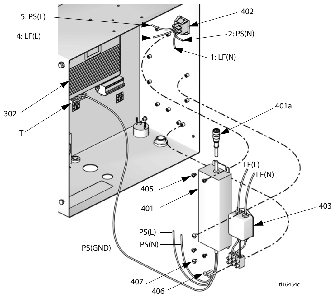
Rys. 8. Wymiana zasilacza naściennego
