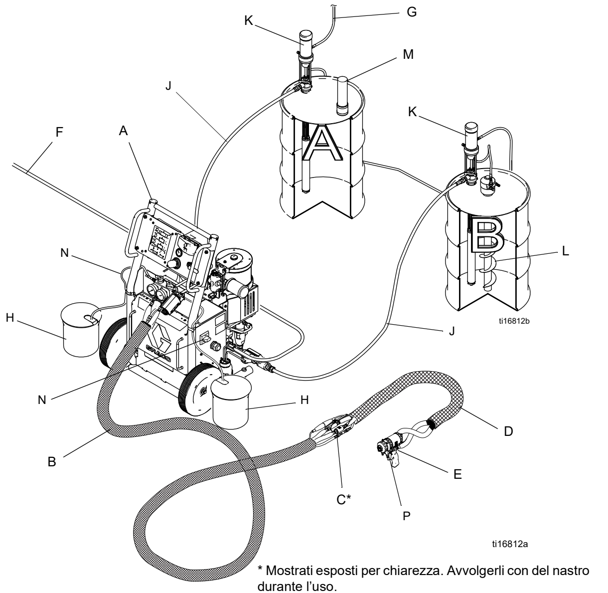
FIG. 1: Installazione tipica, senza ricircolo
