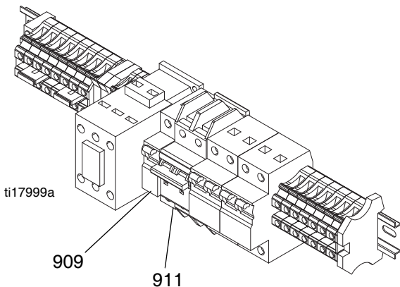
FIG. 13: Modulo interruttore
