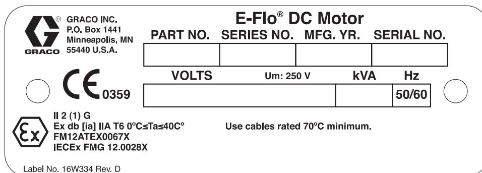
Figure 4 Moteur avancé avec étiquette d'identification des homologations spécifiques à chaque région
