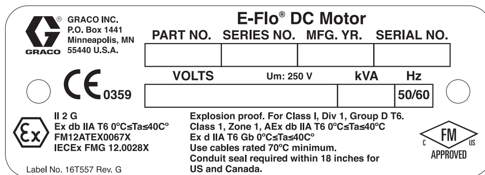
Figure 1 Étiquette d'identification du moteur de base
