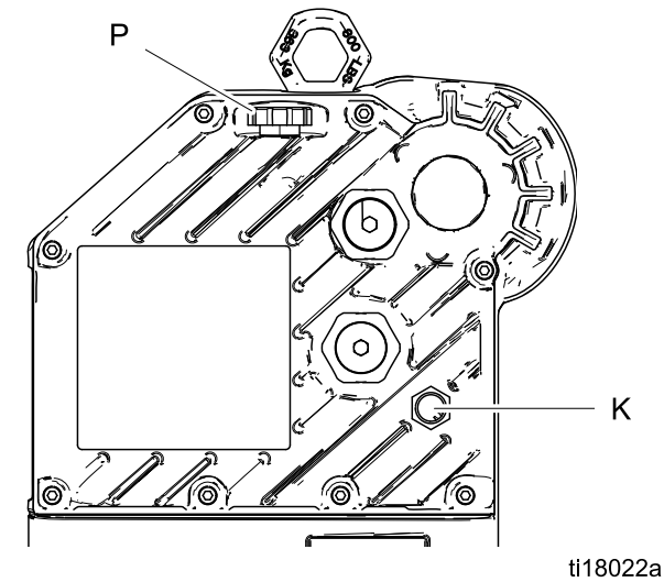
Figure 5 Fenêtre et bouchon de remplissage d'huile
