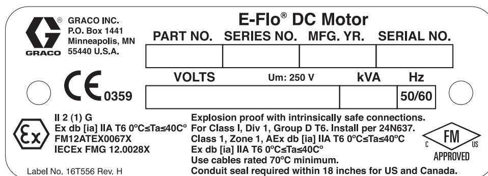
Figure 3 Étiquette d'identification du moteur avancé
