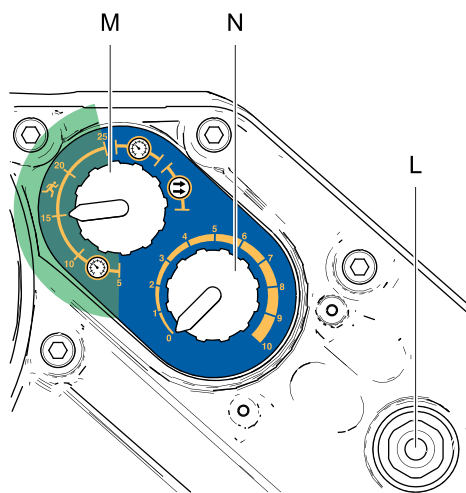
Figure 12 Mode Pression avec protection d'emballement intégrée
