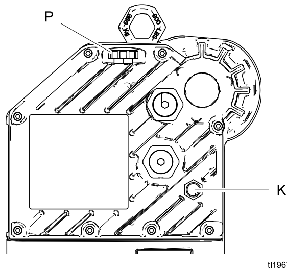
Figure 15 Fenêtre et bouchon de remplissage d'huile
