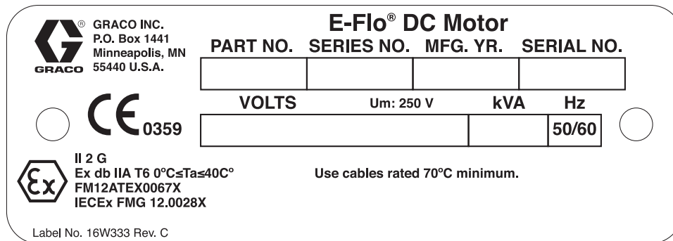
Figure 2 Motore di base con etichette identificative delle approvazioni regionali
