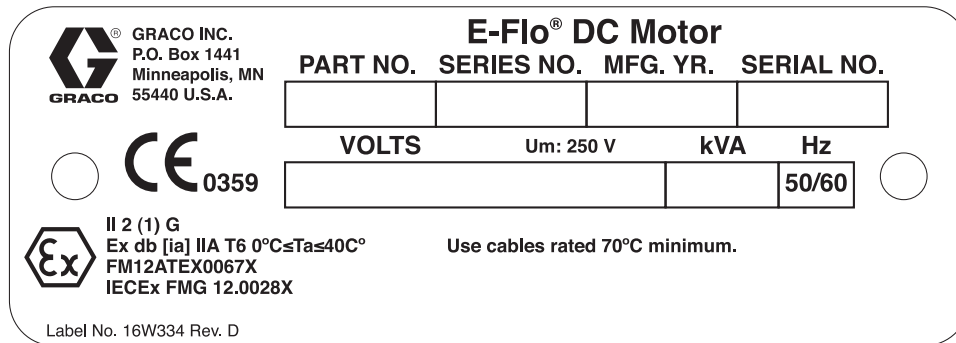
Figure 4 Motore avanzato con etichette identificative delle approvazioni regionali
