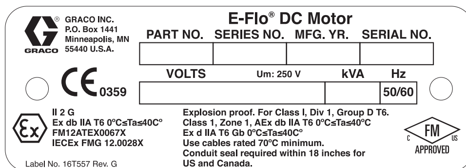
Figure 1 Etichetta identificativa del motore di base
