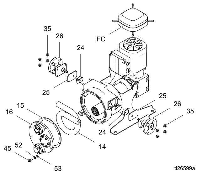
Figure 2 Remoção ou instalação da mangueira
