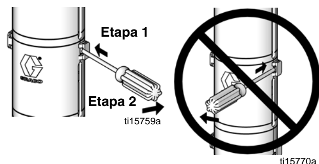
FIG. 3. Desmontagem das proteções
