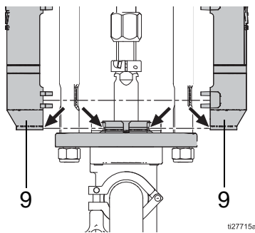
FIG. 4. Remontagem das proteções
