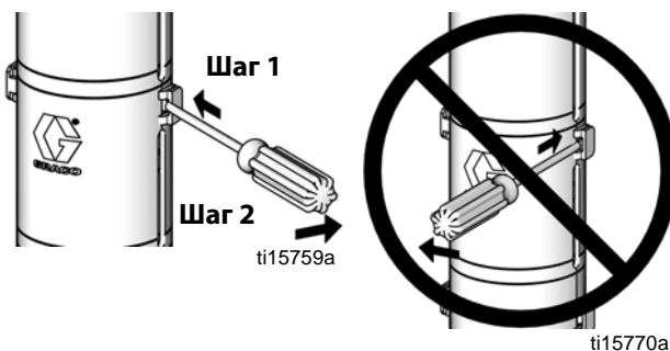
Рис. 3. Разборка экрана
