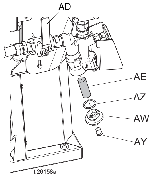
图 54：入口阀组装
