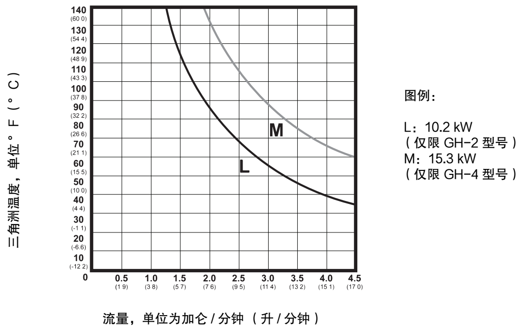
图 79：加热器性能
