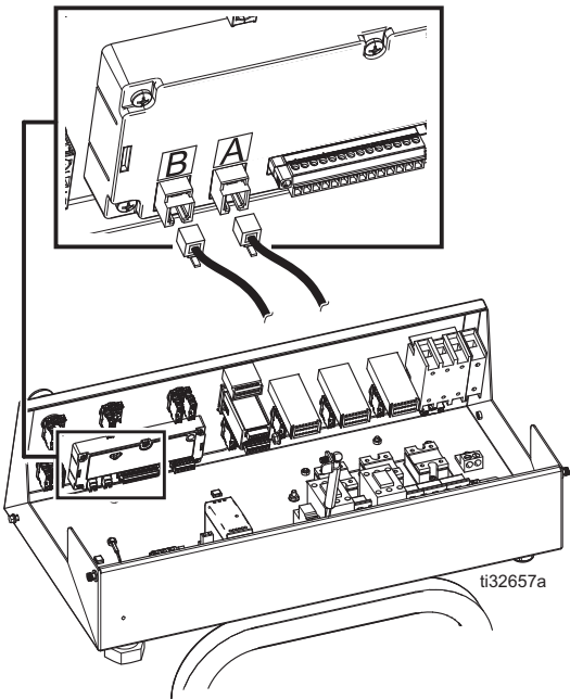
图 66：传感器电缆
