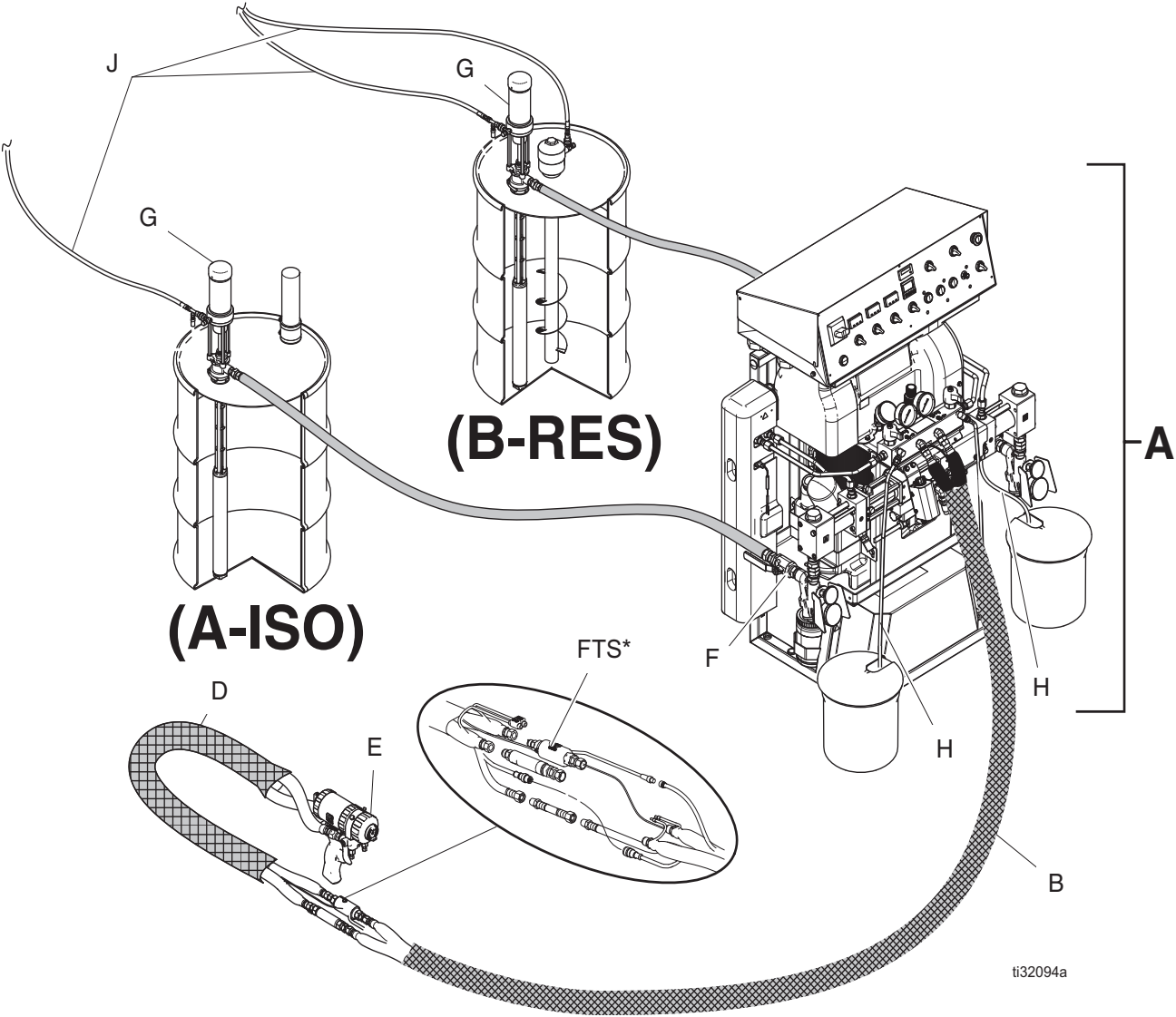
图 1：典型安装
