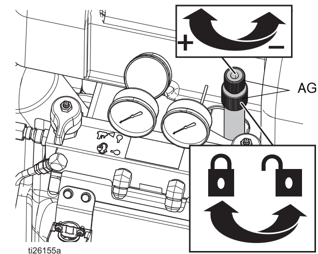
图 31：液压调节
