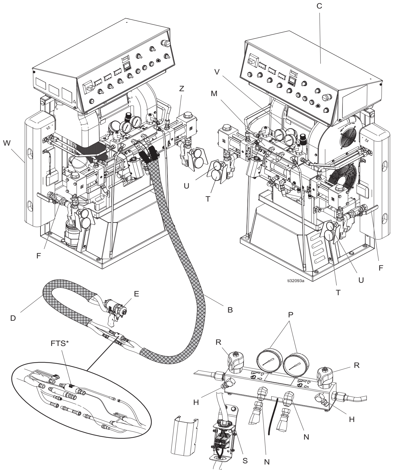
图 4：组件识别
