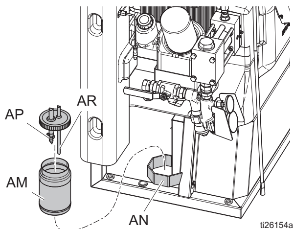
图 55：泵润滑系统
