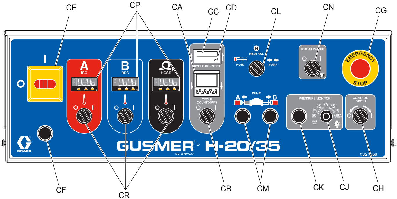
图 5：控制面板
