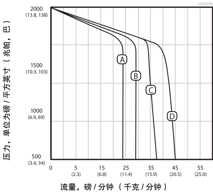
图 78: GH-2 与 GH-4 泡沫性能
