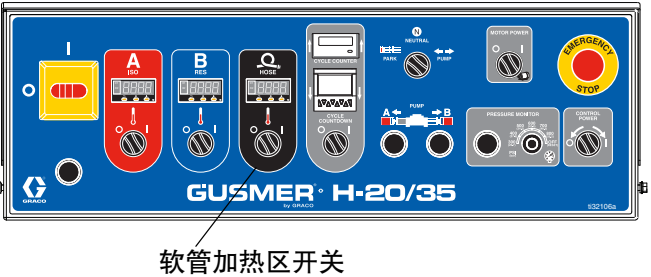
图 24：软管加热区开关
