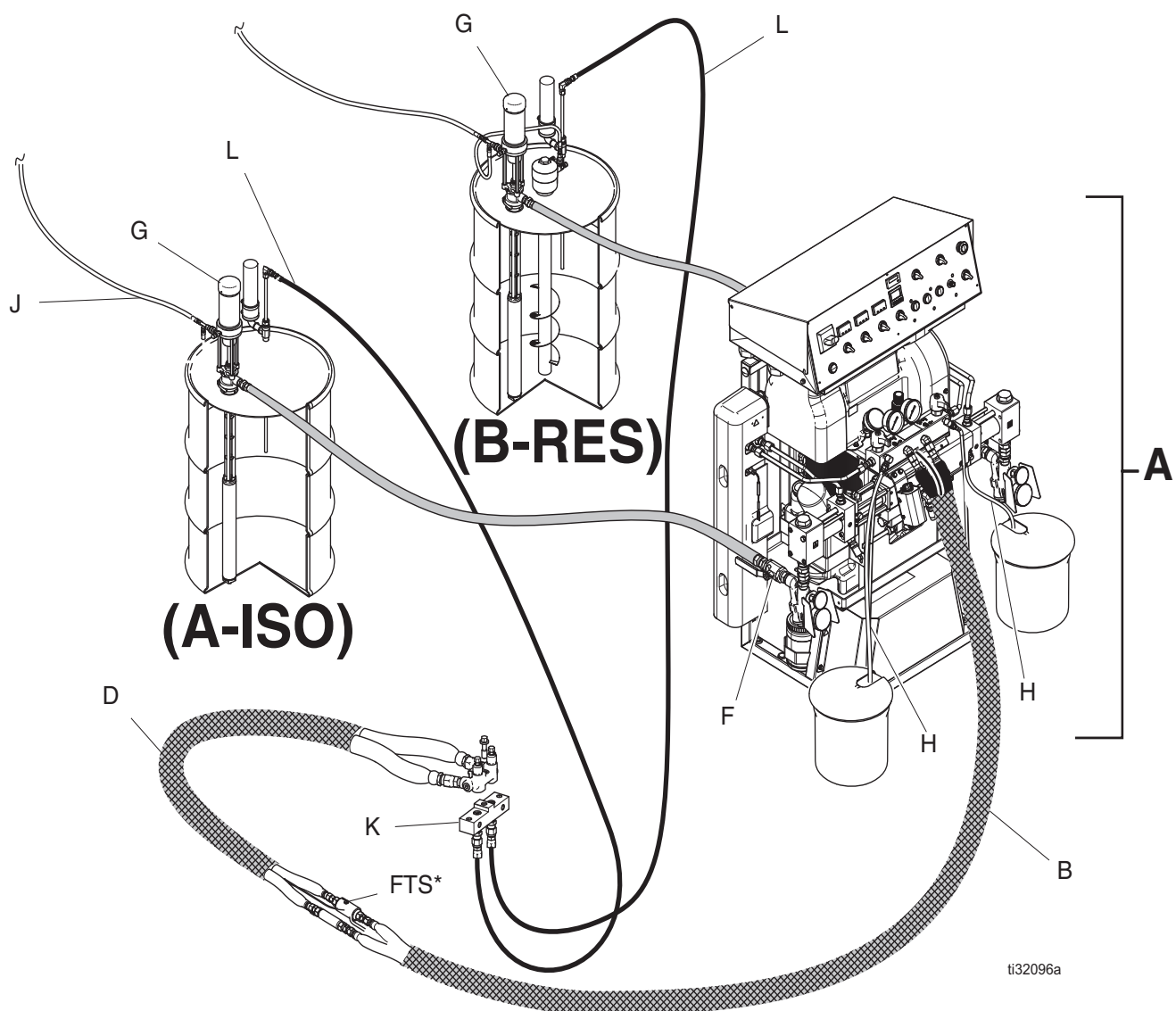
图 3: 典型安装
