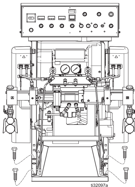
图 6：安装到地面
