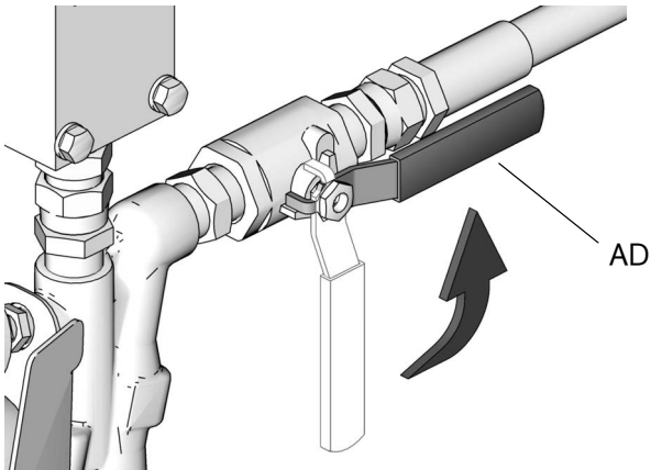
图 38：入口阀组装
