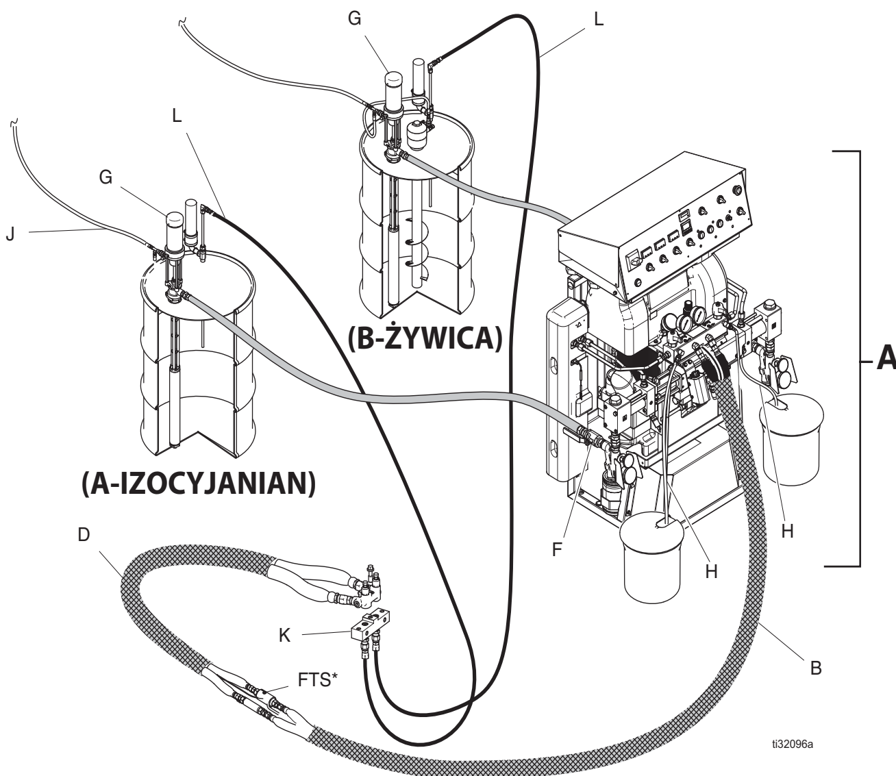
Rys. 3 Typowa instalacja
