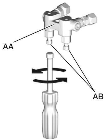
Rys. 11: Rozdzielacz pistoletu
