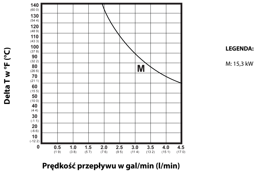
Rys. 79: Wydajność podgrzewacza
