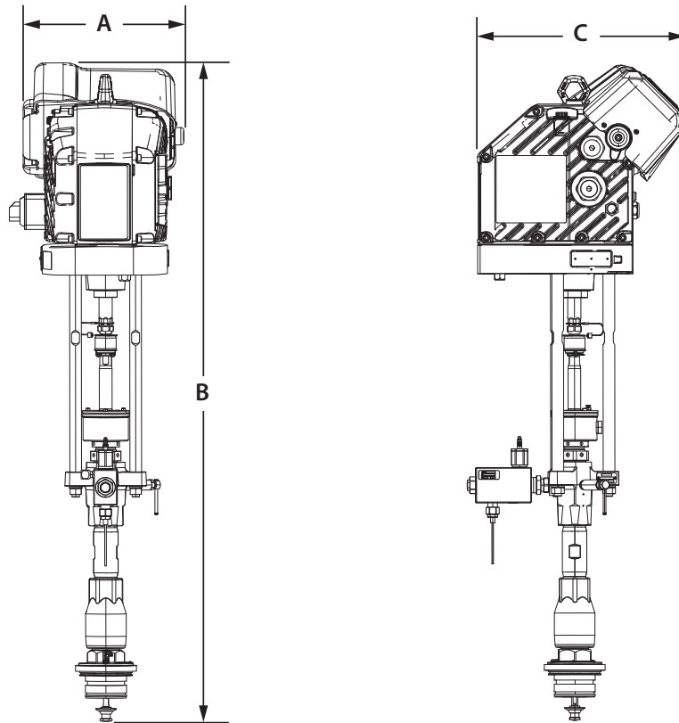
図 31: 220cc Dura-Flo CS ポンプシステム寸法
