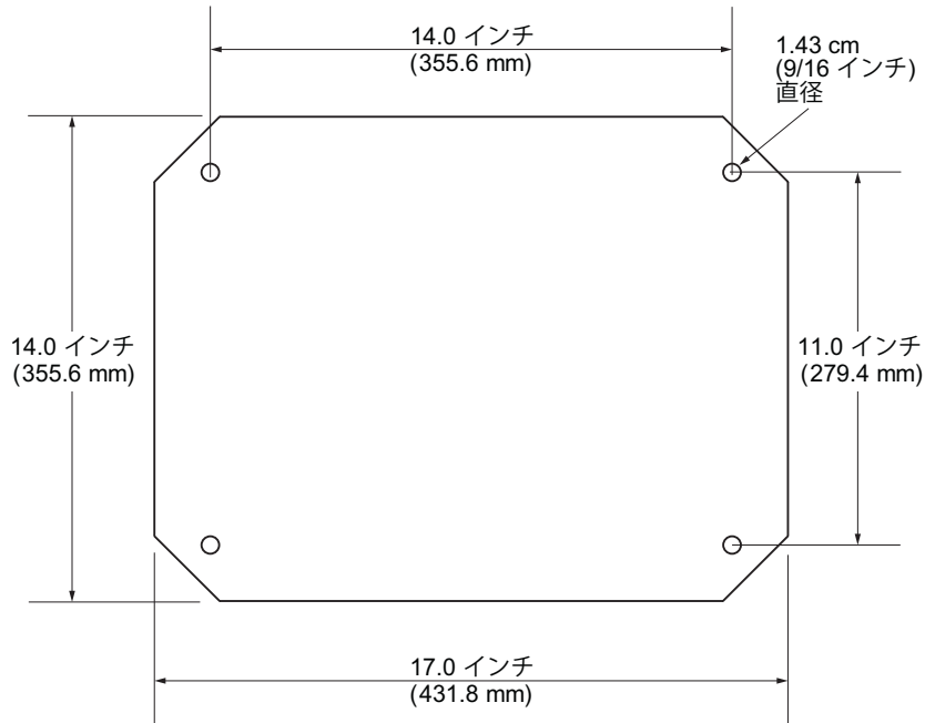
図 33: フロアスタンド取り付け穴
