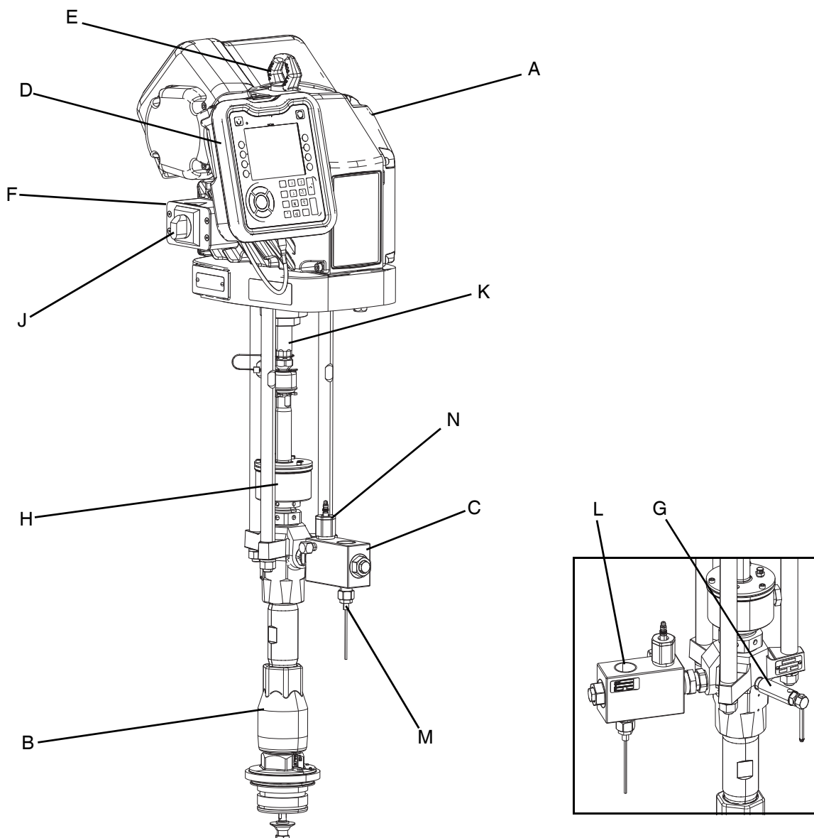
図 1: E-Flo SP 構成部品
