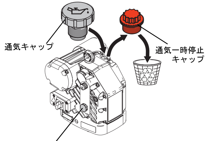
図 10: 通気一時停止キャップおよび通気オイルキャップ
