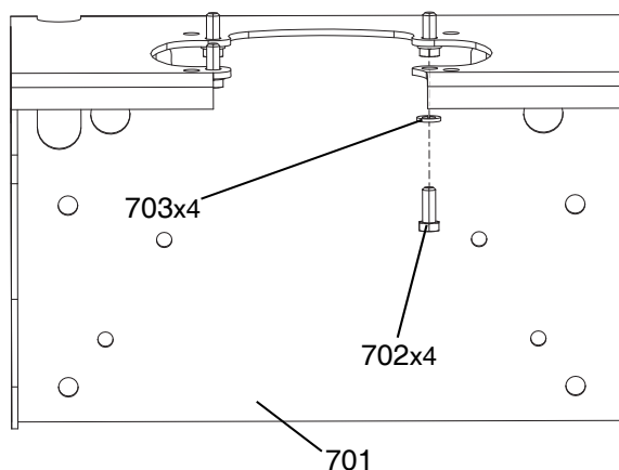
図 28: 壁取り付けブラケット
