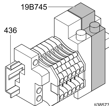
Figure 20 Монтажные соединения комплекта 26B414
