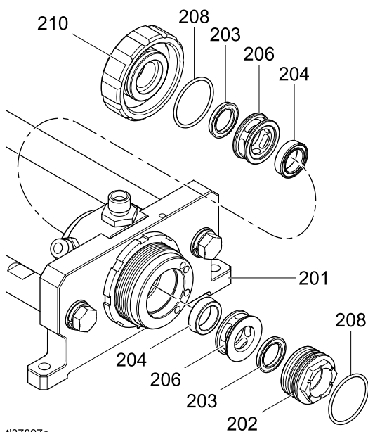
Figure 45 Нижний фиксатор
