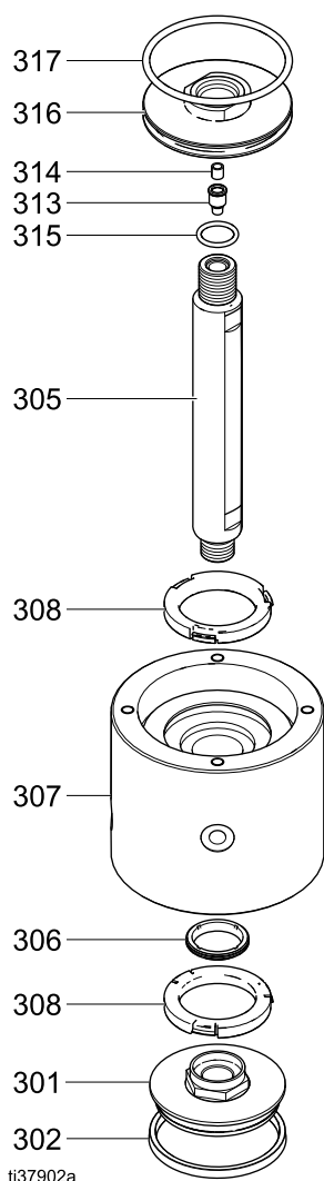
Figure 51 Части среднего корпуса
