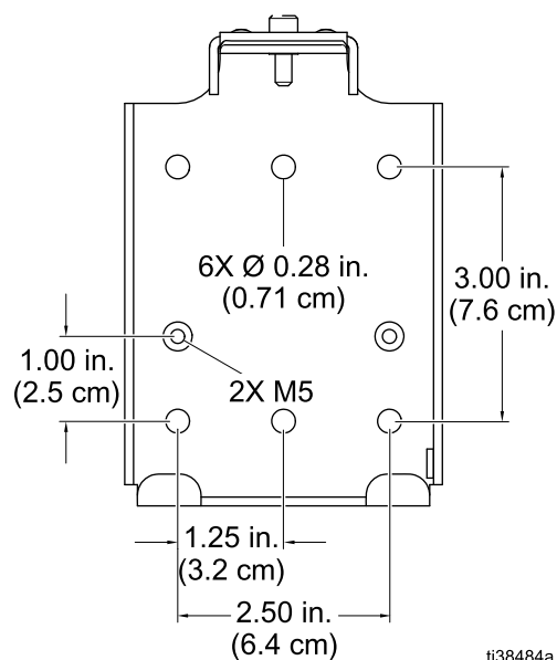
Figure 16 Монтажные отверстия кронштейна (41)
