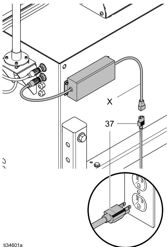
Figure 17 Подключения блока питания
