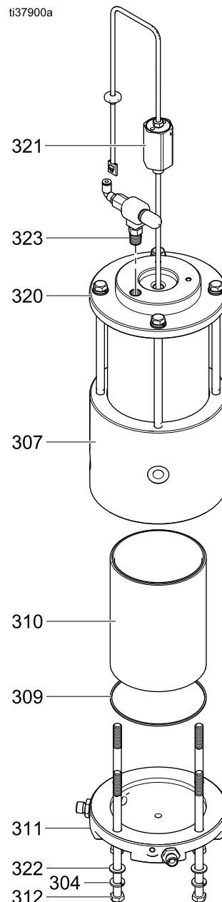
Figure 49 Снимите крышку смачиваемой секции.
