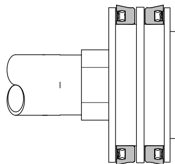
Figure 44 U-образные детали обращены в противоположные стороны
