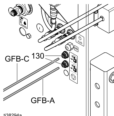
Figure 19 Соединения блока промывки краскораспылителя на изолирующей системе
