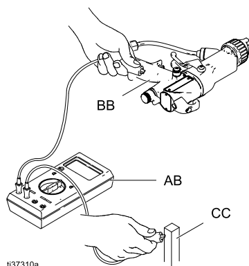
Figure 22 Проверка электрического заземления краскораспылителя
