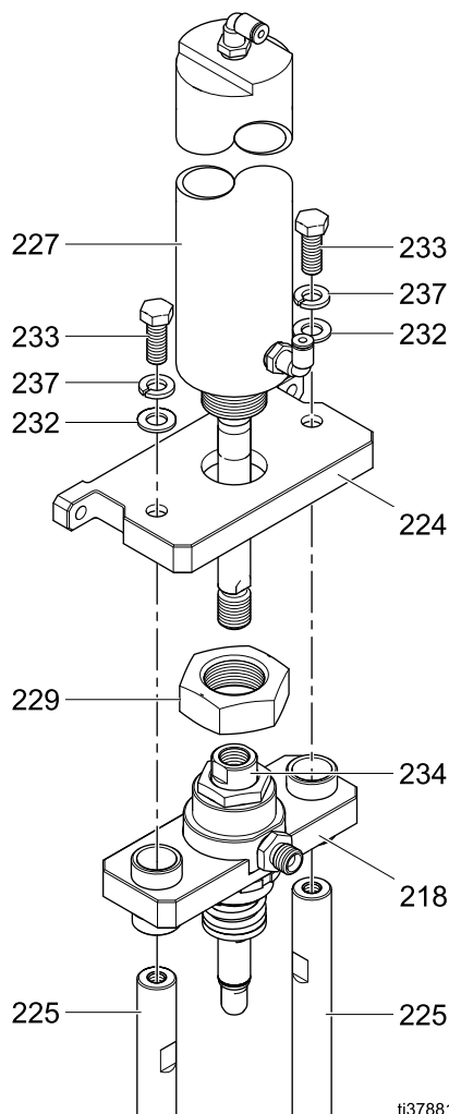
Figure 38 Узлы и детали изоляционного клапана
