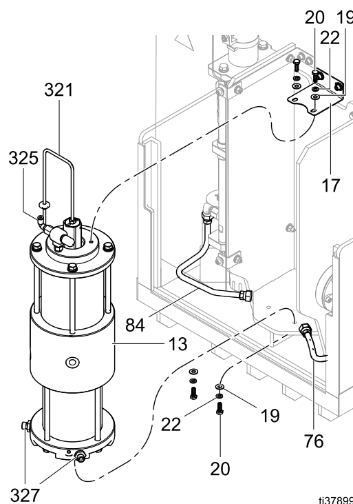
Figure 48 Извлечение изоляционного насоса
