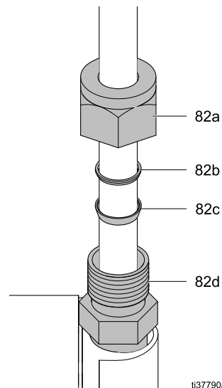
Figure 10 Ориентация муфты на шланге для материала
