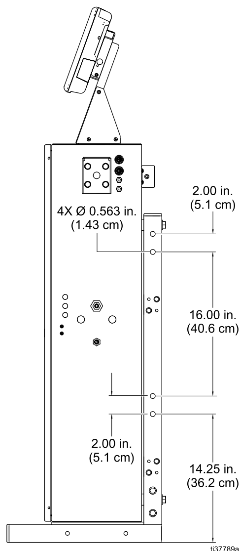
Figure 4 Схема расположения монтажных отверстий для настенного монтажа
