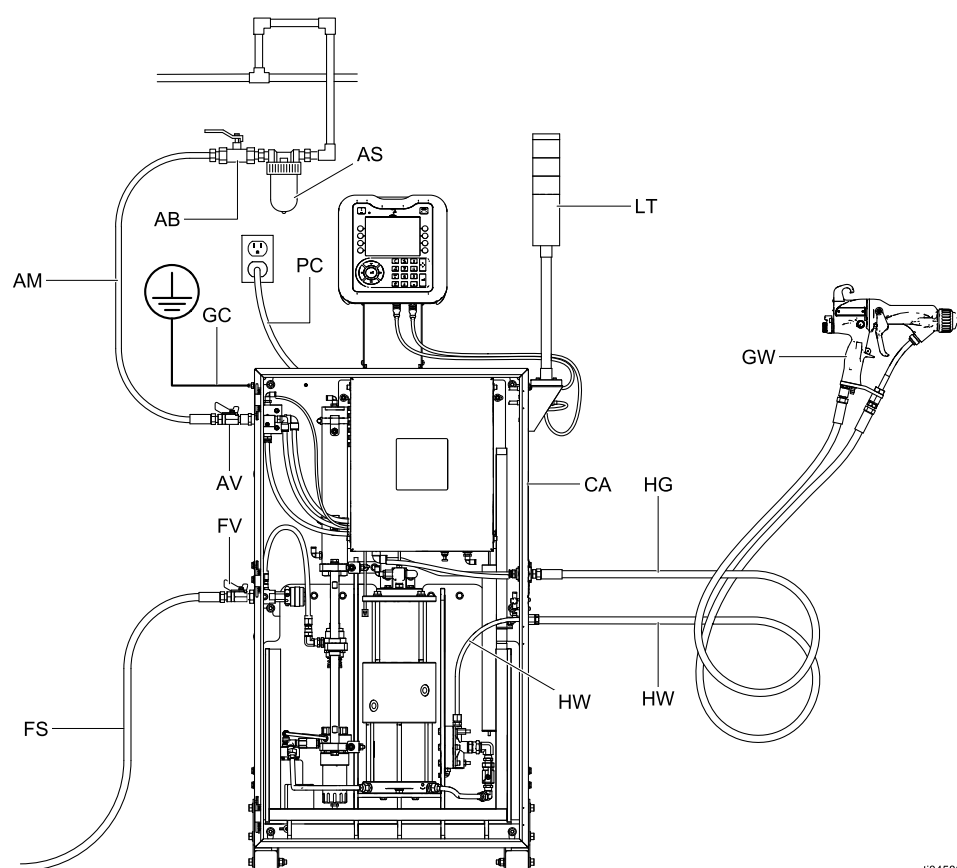
Figure 2 Типовой монтаж ручной системы воздушного распыления материала на водной основе для безопасной зоны
