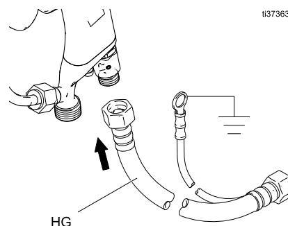
Figure 21 Заземление красного шланга Graco
