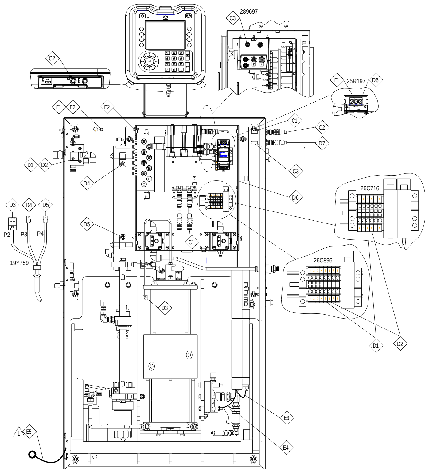
Figure 56 Подключения проводов
