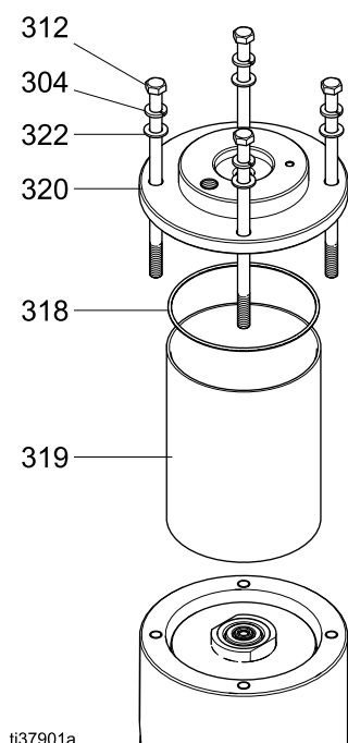
Figure 50 Демонтаж крышки воздушной камеры
