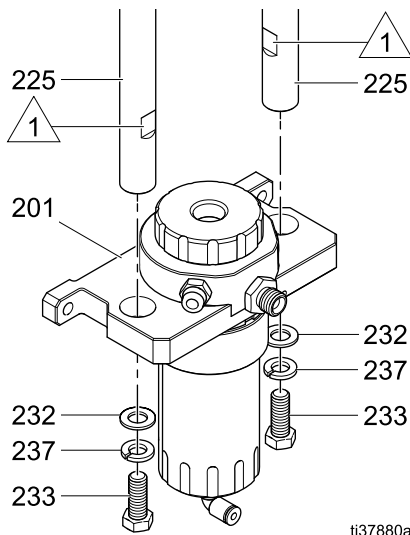
Figure 36 Стержни возле основания корпуса
