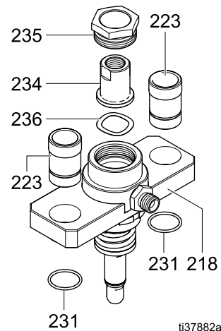
Figure 37 Узлы и детали корпуса челнока
