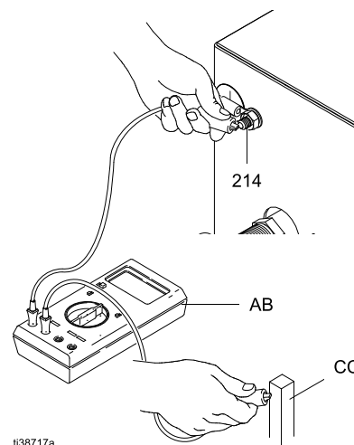
Figure 23 Проверка заземления шкафа
