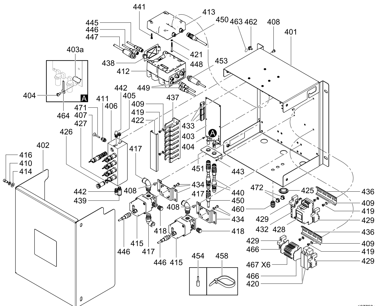
Figure 62 Электронные средства управления
