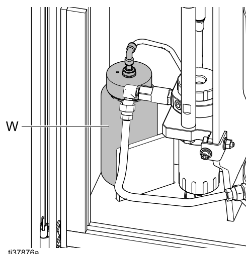
Figure 12 Замена емкости с моющей жидкостью
