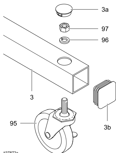
Figure 3 Детали крепления колеса
