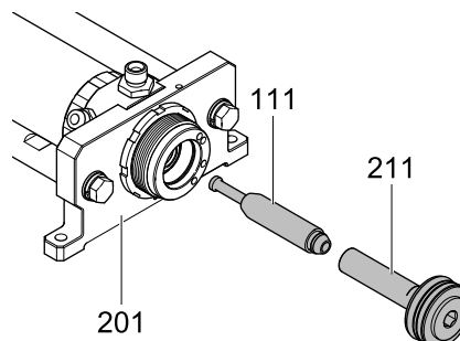
Figure 46 Прохождение инструмента поршня через нижнюю часть корпуса
