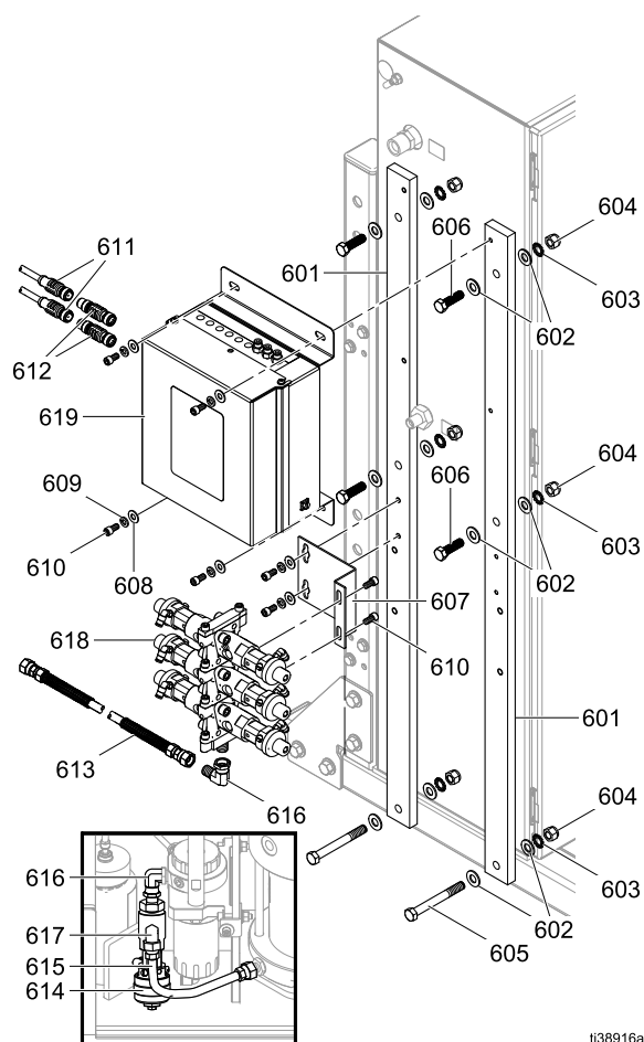
Figure 63 Комплект блока смены цвета 26B415
