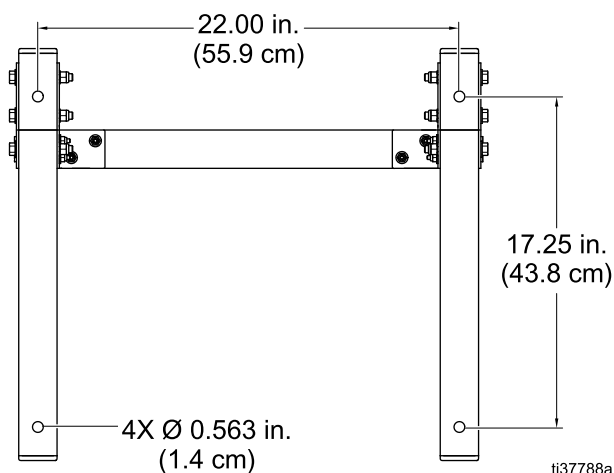
Figure 6 Схема расположения болтов для напольного монтажа
