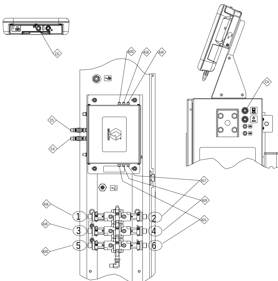
Figure 57 Пневматические и электрические соединения модуля смены цвета
