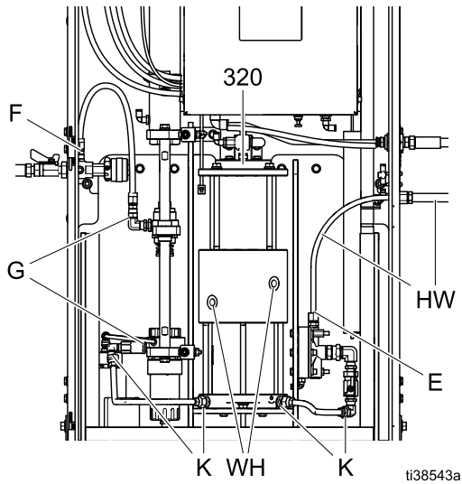
Figure 31 Проверьте наличие утечек материала
