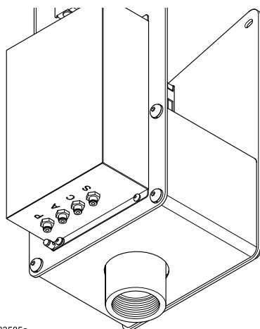
Figure 18 Разъемы блока промывки краскораспылителя
