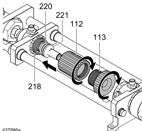
Figure 39 Инструменты для снятия штока клапана
