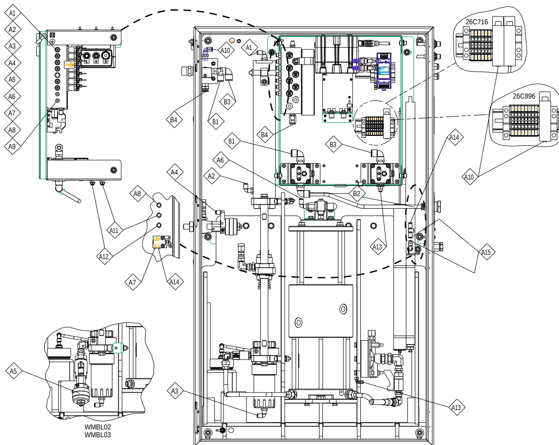
Figure 55 Пневматические соединения
