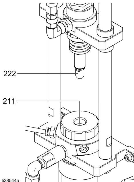
Figure 32 Вытрите узлы и детали изоляционного клапана
