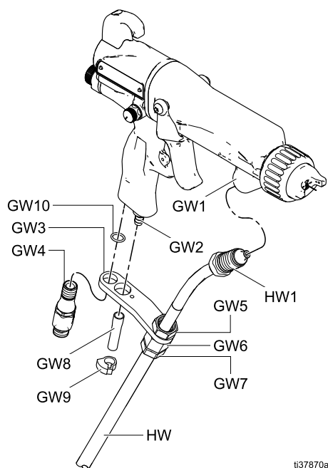
Figure 7 Присоединение шланга для материала к краскораспылителю
