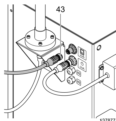
Figure 14 Подключение кабеля CAN контроллера к шкафу (без блока смены цвета)
