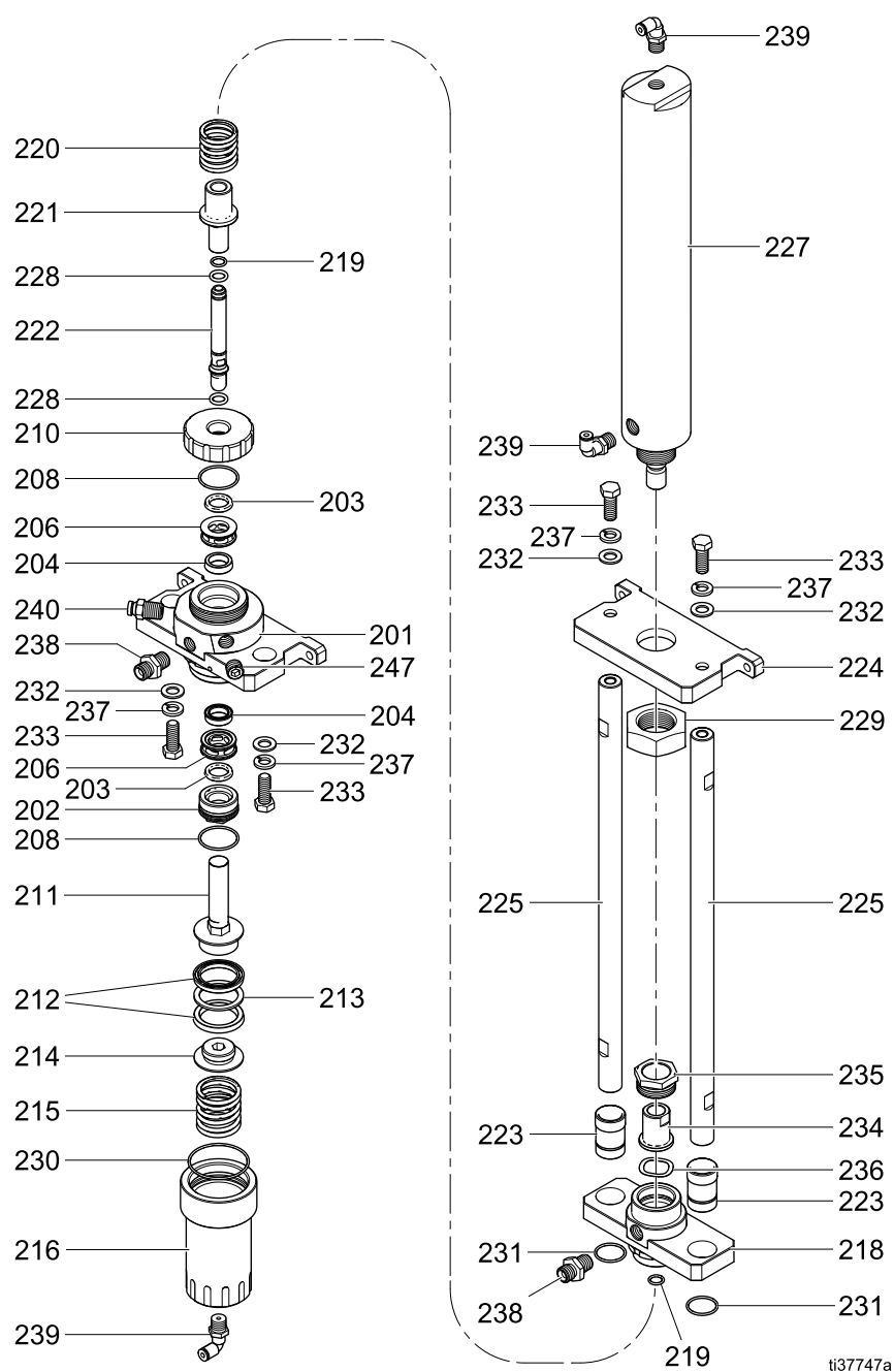
Figure 60 Изоляционный клапан
