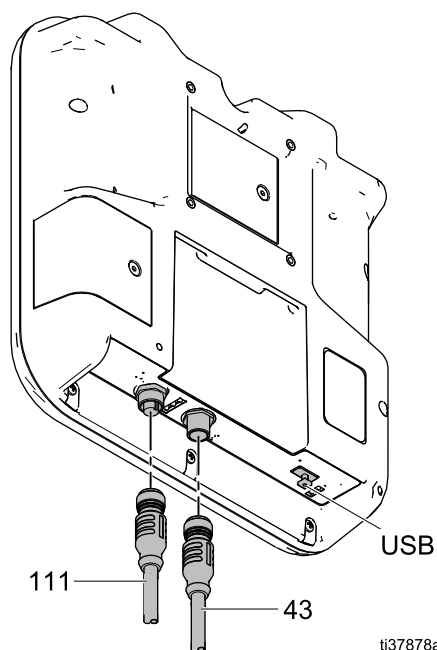
Figure 15 Подключения к интерфейсу управления (системы без блока смены цвета)
