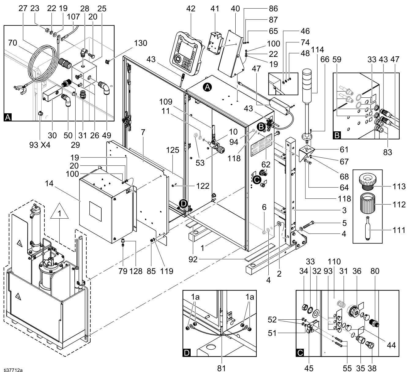
Figure 58 Изолирующий шкаф
