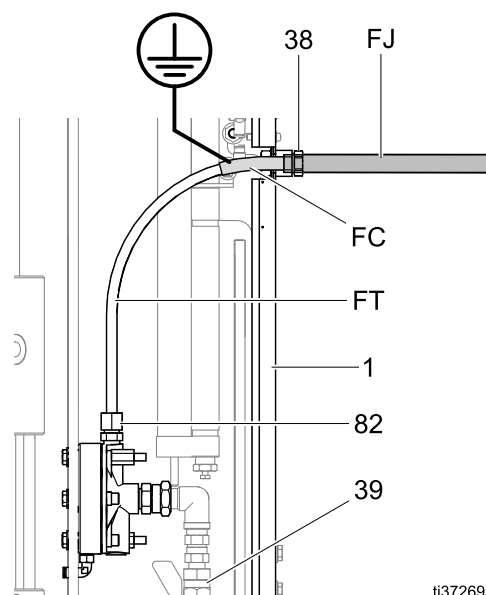
Figure 8 Экранированный соединитель шлангов в изолирующем шкафу
