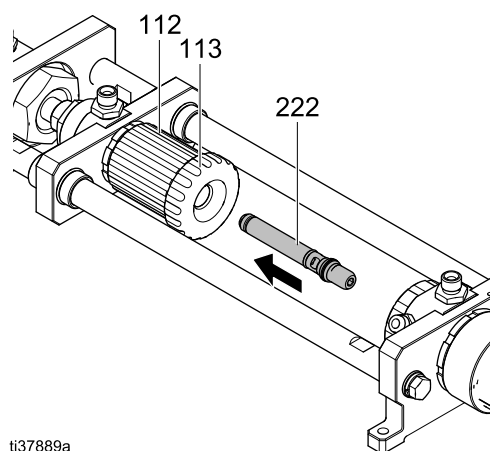
Figure 42 Вставка штока клапана в инструменты
