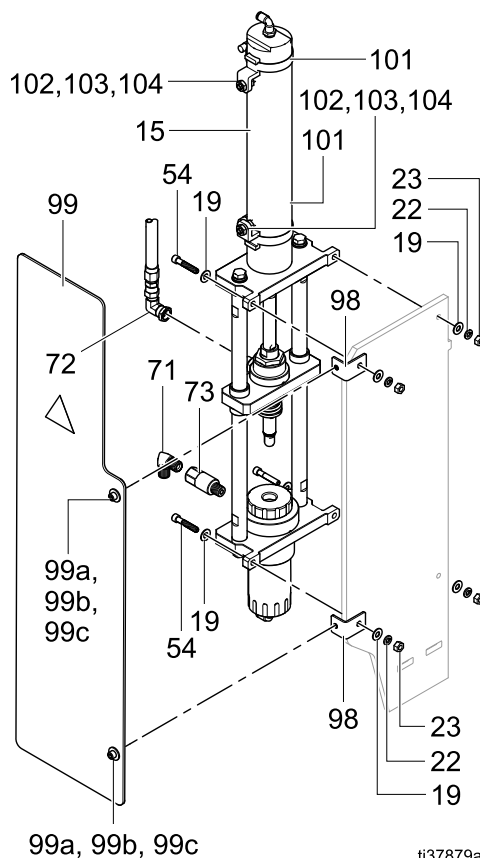
Figure 34 Крепление изоляционного клапана к стойке шкафа
