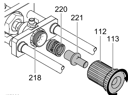
Figure 41 Установка пружины и муфты в инструмент
