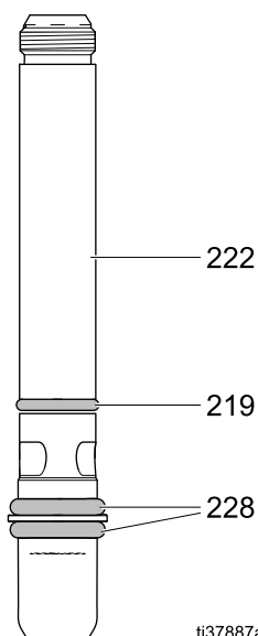
Figure 40 Замена уплотнительных колец изоляционного клапана
