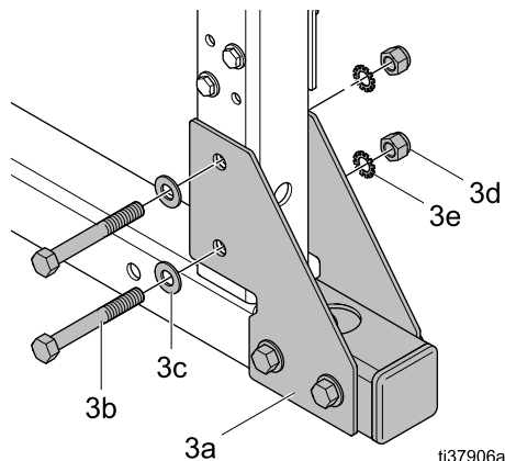
Figure 5 Снятие ножек рамы
