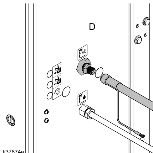
Figure 11 Расположение воздушного соединения
