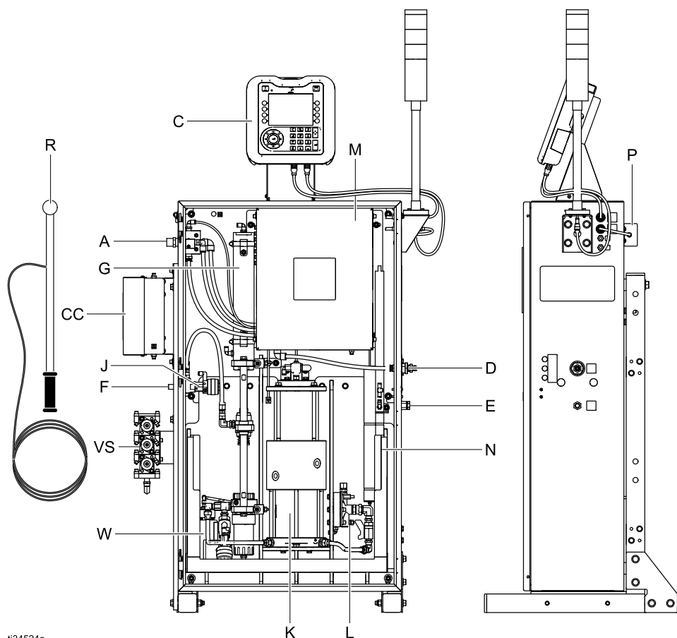
Figure 1 Узлы и детали изолирующей системы пневматического распыления в типичной системе ручного дозирования материалов на водной основе
