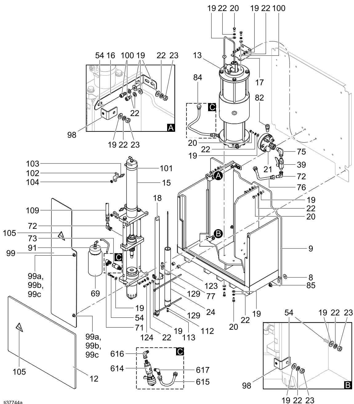
Figure 59 Внутренняя часть изолирующего шкафа
