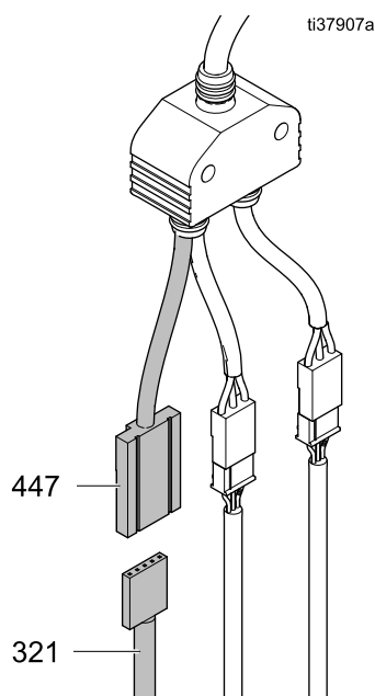
Figure 47 Подключение датчика насоса на панели электроники
