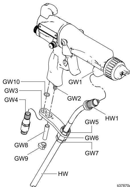
Figure 7 Ansluta färgslangen till pistolen
