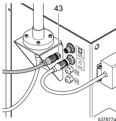
Figure 14 Anslutningar för styrningens CAN-kablar i skåpet (utan kulörbyte)
