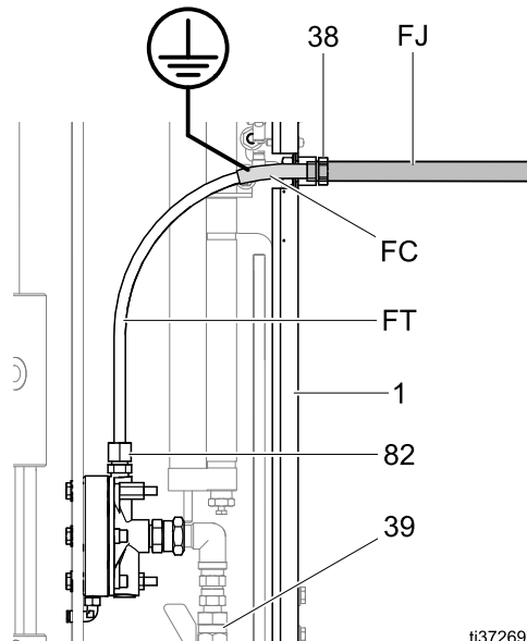
Figure 8 Skärmad slanganslutning vid isolationsskåp
