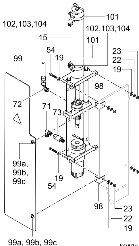
Figure 34 Fästa isolationsventilen på skåpsstativet
