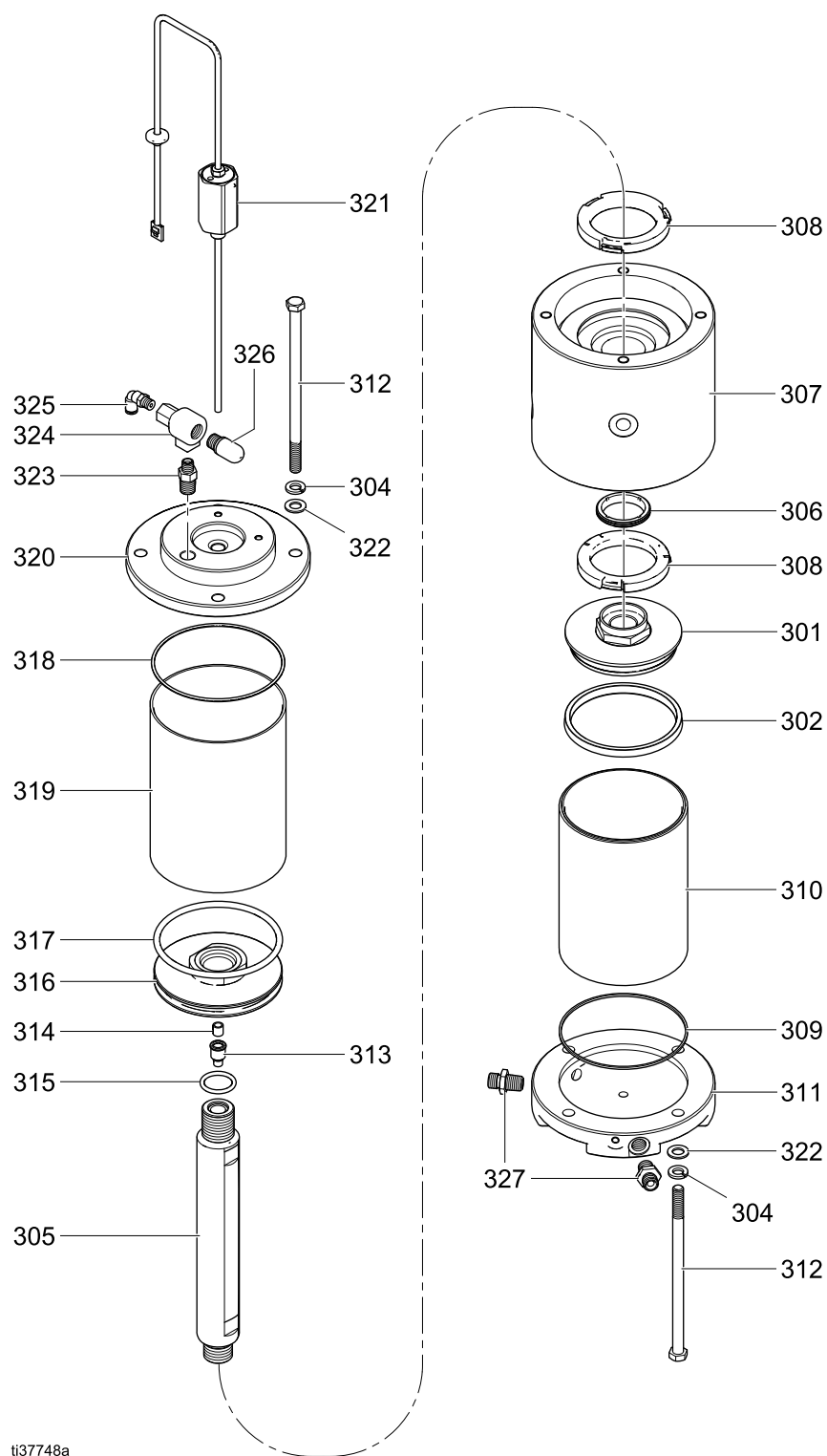
Figure 61 Isolationsvätskepump
