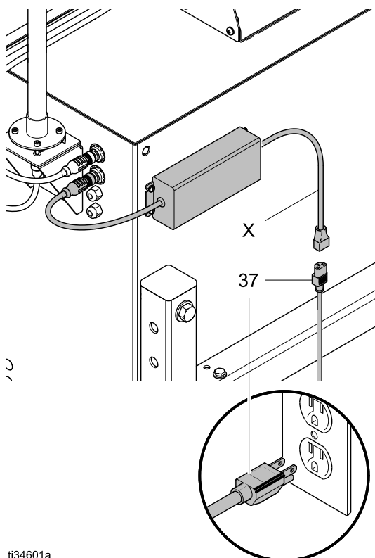
Figure 17 Anslutning av nätaggregat
