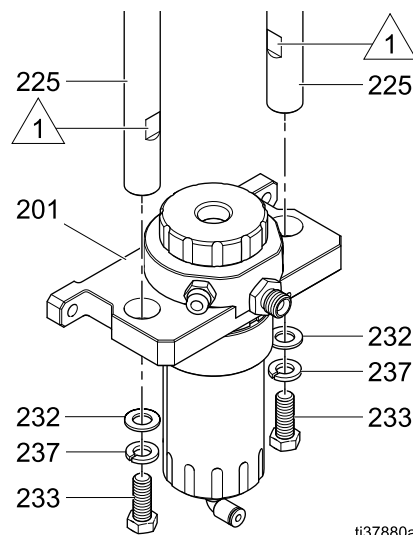
Figure 36 Stänger invid basplattan
