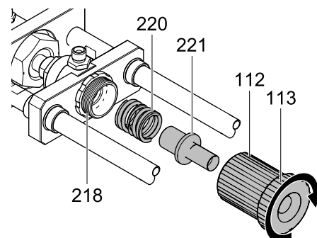
Figure 41 Återmontera fjäder och hylsa i verktyget
