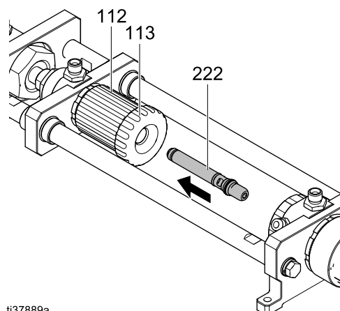
Figure 42 Föra in ventilskaftet i verktygen
