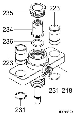
Figure 37 Skyttelhusets komponenter
