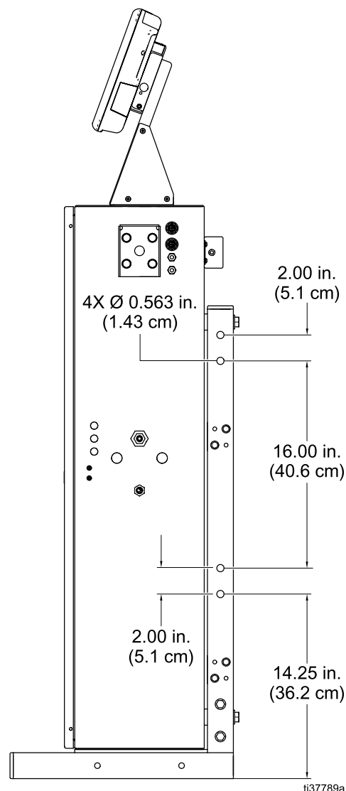
Figure 4 Hålmönster för väggmontering
