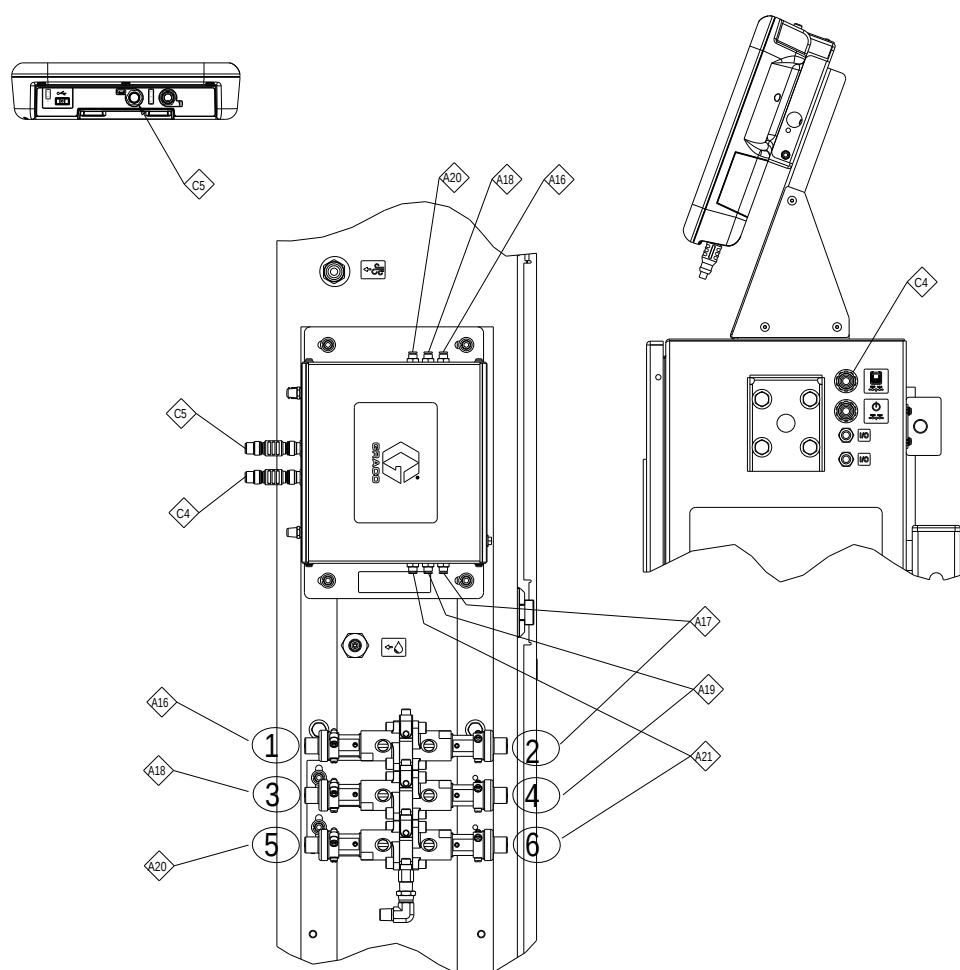
Figure 57 Kulörbytesmodulens elanslutning och pneumatiska anslutningar
