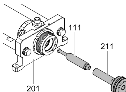
Figure 46 Kolvverket förs genom nedre hus
