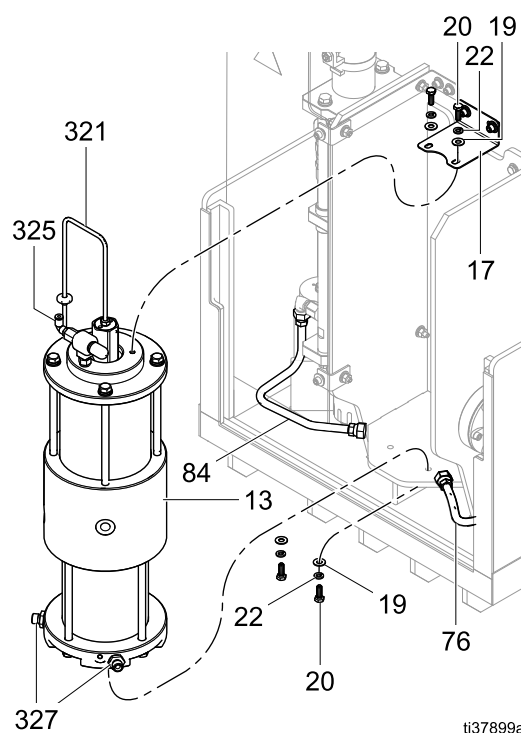
Figure 48 Ta bort isolationsvätskepumpen
