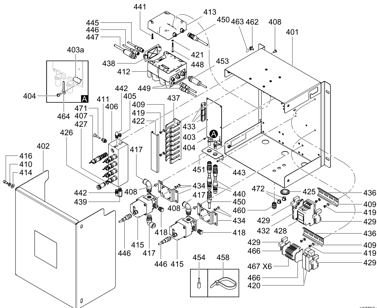
Figure 62 Elektriska komponenter
