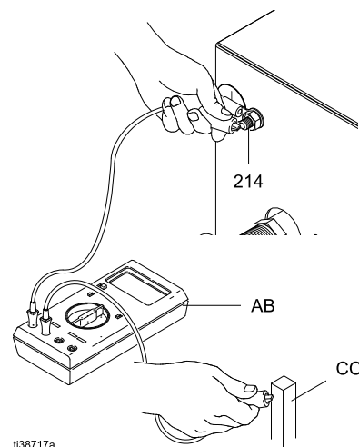
Figure 23 Kontrollera jordning av skåp
