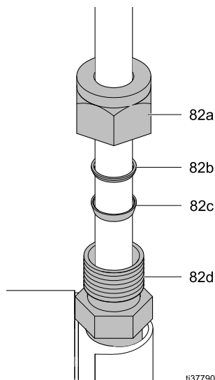
Figure 10 Hylsornas placering på vätskeslangen
