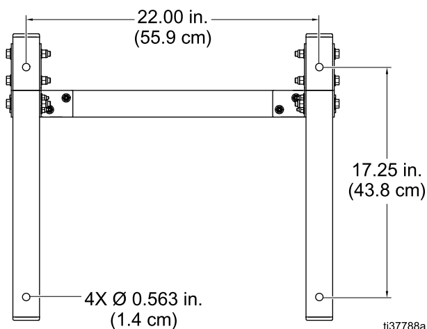
Figure 6 Skruvhålsmönster för golvmontering
