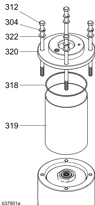
Figure 50 Ta bort luftkåpan
