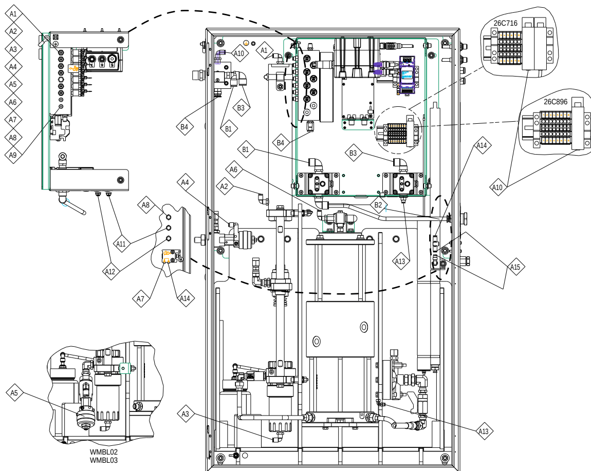
Figure 55 Pneumatiska anslutningar
