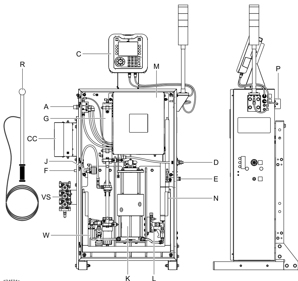
Figure 1 Komponenter i isolationssystemet för en tryckluftsspruta i ett typiskt manuellt batchsystem för vattenburna material
