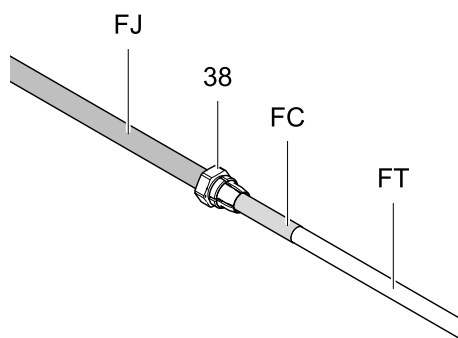
Figure 9 Montering på slitlagret på slang för vattenburna material
