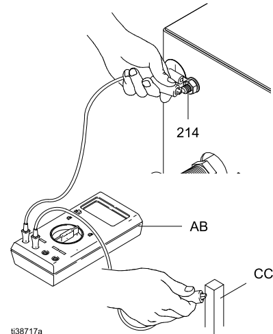
Figure 23 캐비닛 접지 점검
