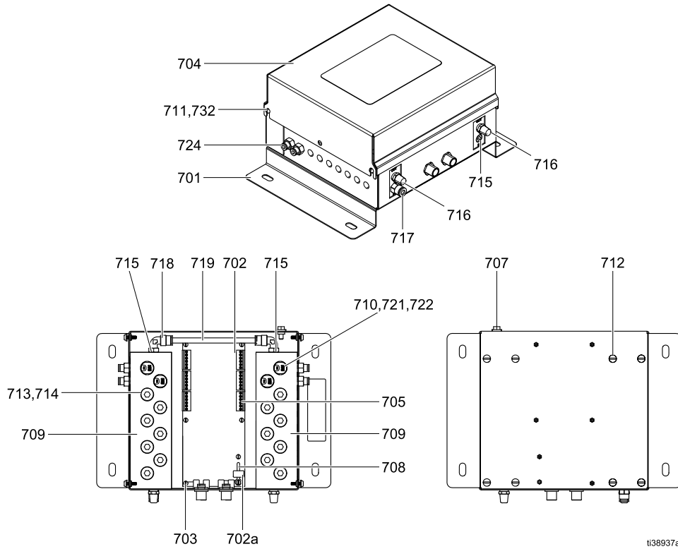
Figure 64 제어 모듈 수리(비 IS 모듈이 표시됨)
