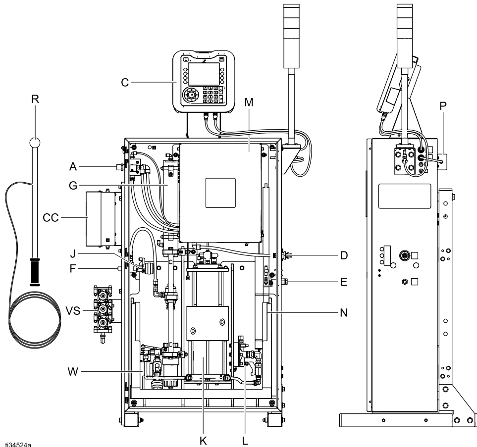
Figure 1 일반적인 수성 수동 배치 시스템의 에어 스프레이 절연 시스템 구성품
