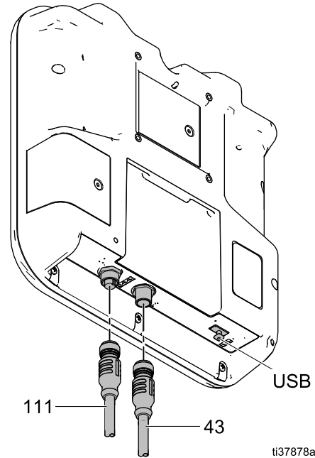
Figure 15 제어 인터페이스 연결부(컬러 체인지 없는 시스템)
