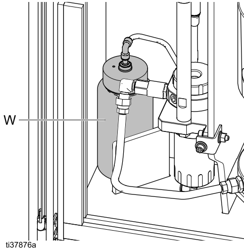
Figure 12 세척액 병 교체
