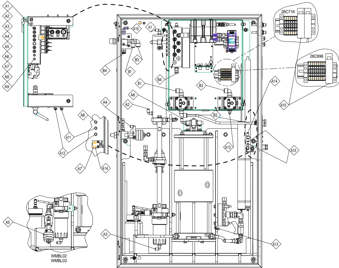
Figure 55 공압 연결
