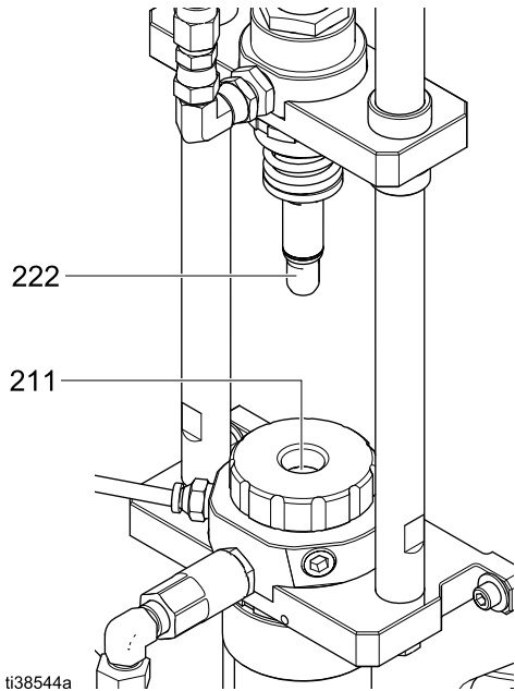
Figure 32 격리 밸브 구성품 뉘기
