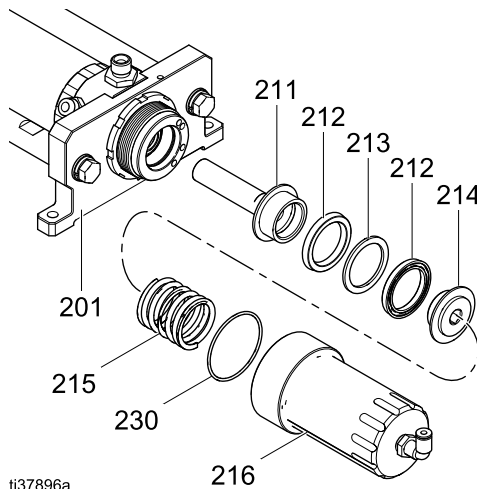
Figure 43 피스톤에서 고정 캡 제거
