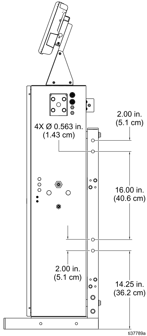
Figure 4 벽 장착 구멍 패턴
