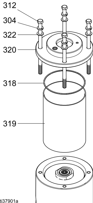
Figure 50 에어 커버 분리
