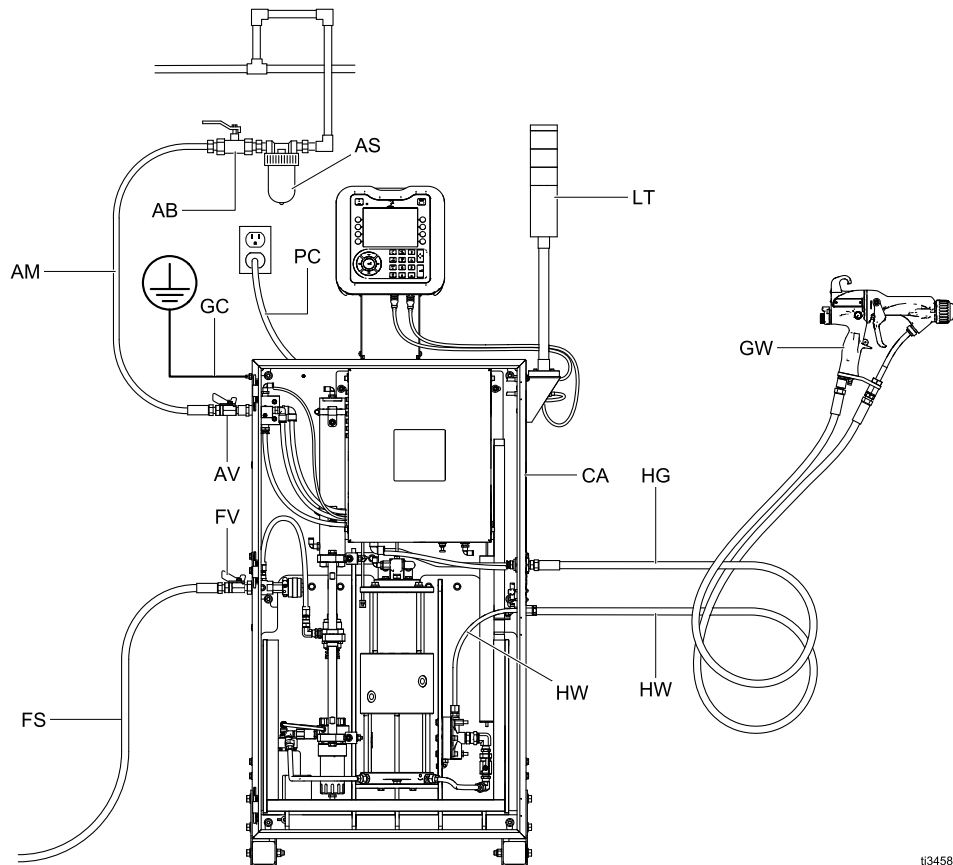
Figure 2 일반 설치, 에어 스프레이 수성 수동 배치 시스템, 비위험 장소
