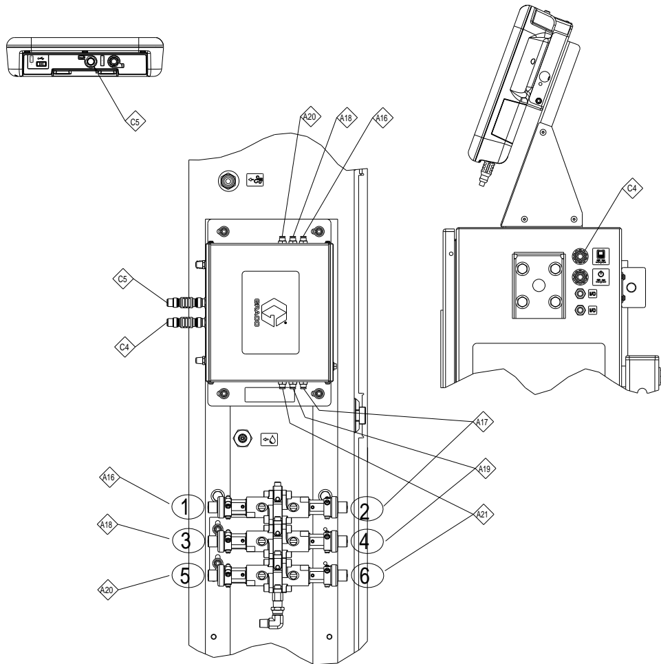
Figure 57 컬러 체인지 모듈 배선 및 공압 연결
