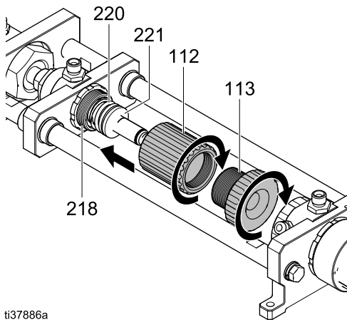
ti37886a Figure 39 밸브 스템 분리 도구
