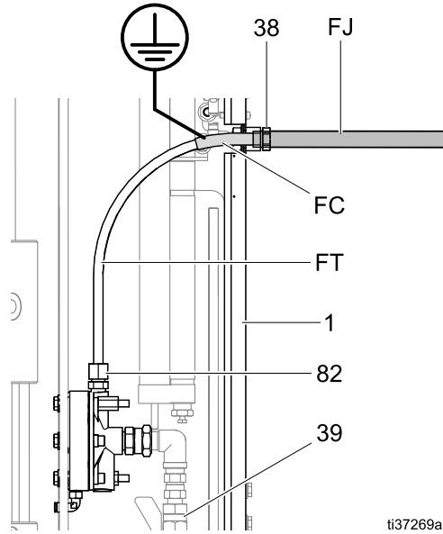
Figure 8 절연 캐비닛에서 차폐 호스 연결
