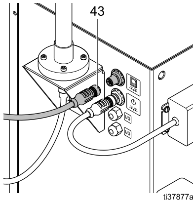
Figure 14 캐비닛의 컨트롤러 CAN 케이블 연결부(컬러 체인지 없음)
