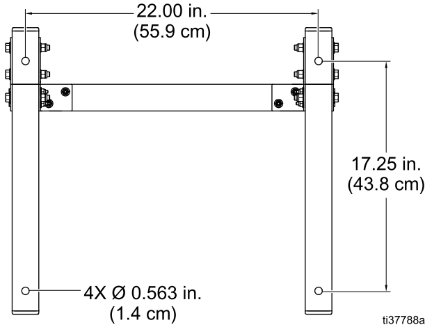
Figure 6 바닥 설치용 볼트 패턴
