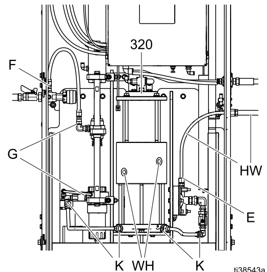
Figure 31 유체 누출 부위 점검
