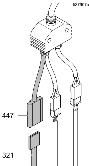
Figure 47 전자 패널의 펌프 센서 연결
