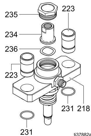
Figure 37 셔틀 하우스 구성품
