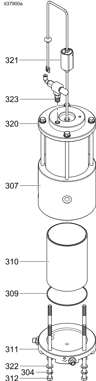
Figure 49 유체 커버 분리
