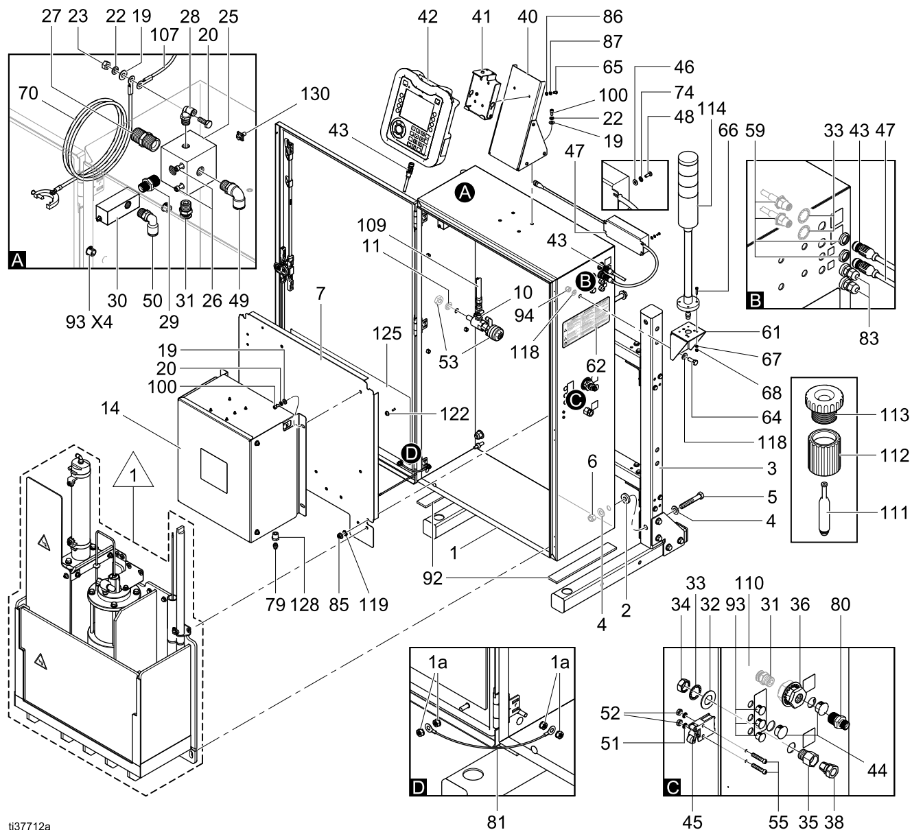
Figure 58 절연 캐비닛
