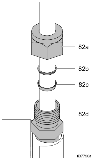
Figure 10 유체 호스의 페룰 방향
