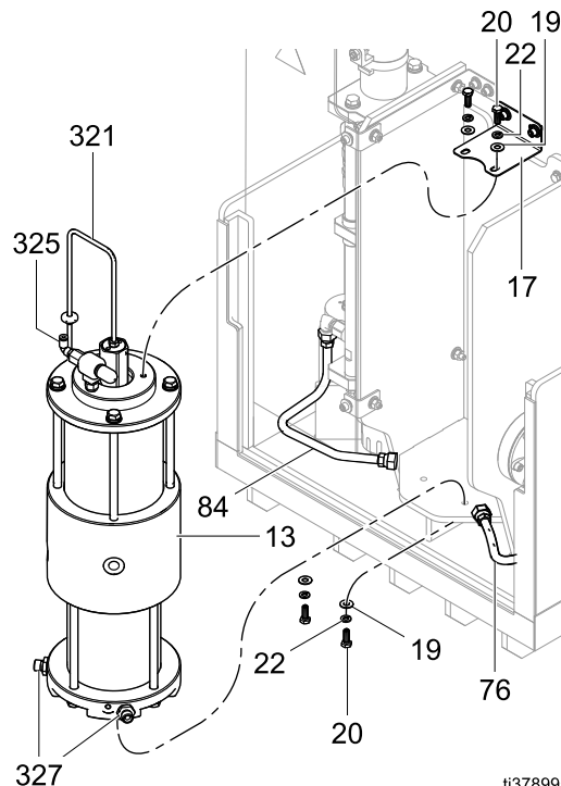
Figure 48 절연 유체 펌프 제거
