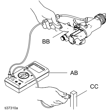
Figure 22 건의 전기 접지 점검
