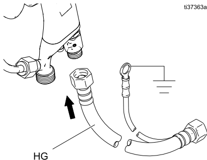
Figure 21 빨간색 Graco 호스 접지
