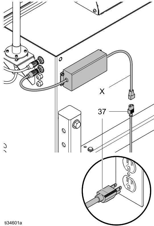
Figure 17 전원 공급 장치 연결
