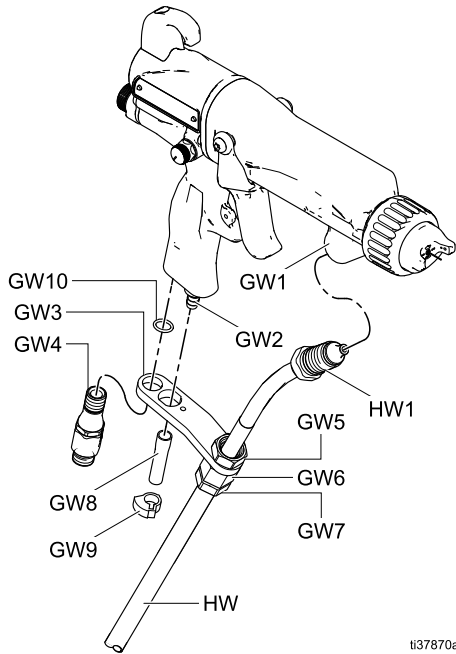
Figure 7 건에 유체 호스를 연결합니다.
