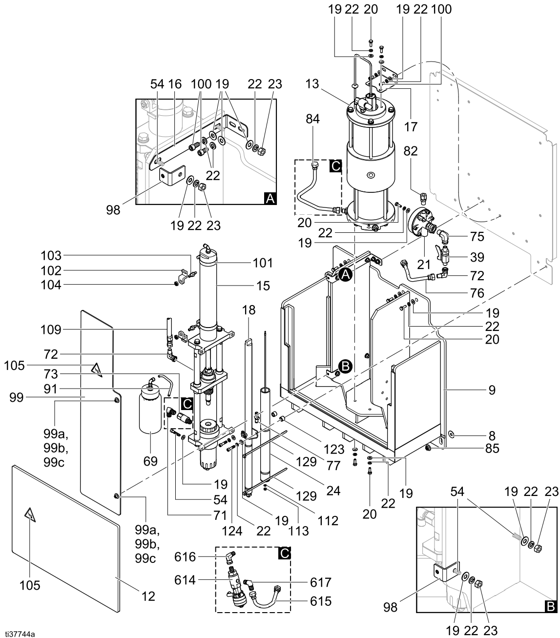
Figure 59 절연 캐비닛 내부
