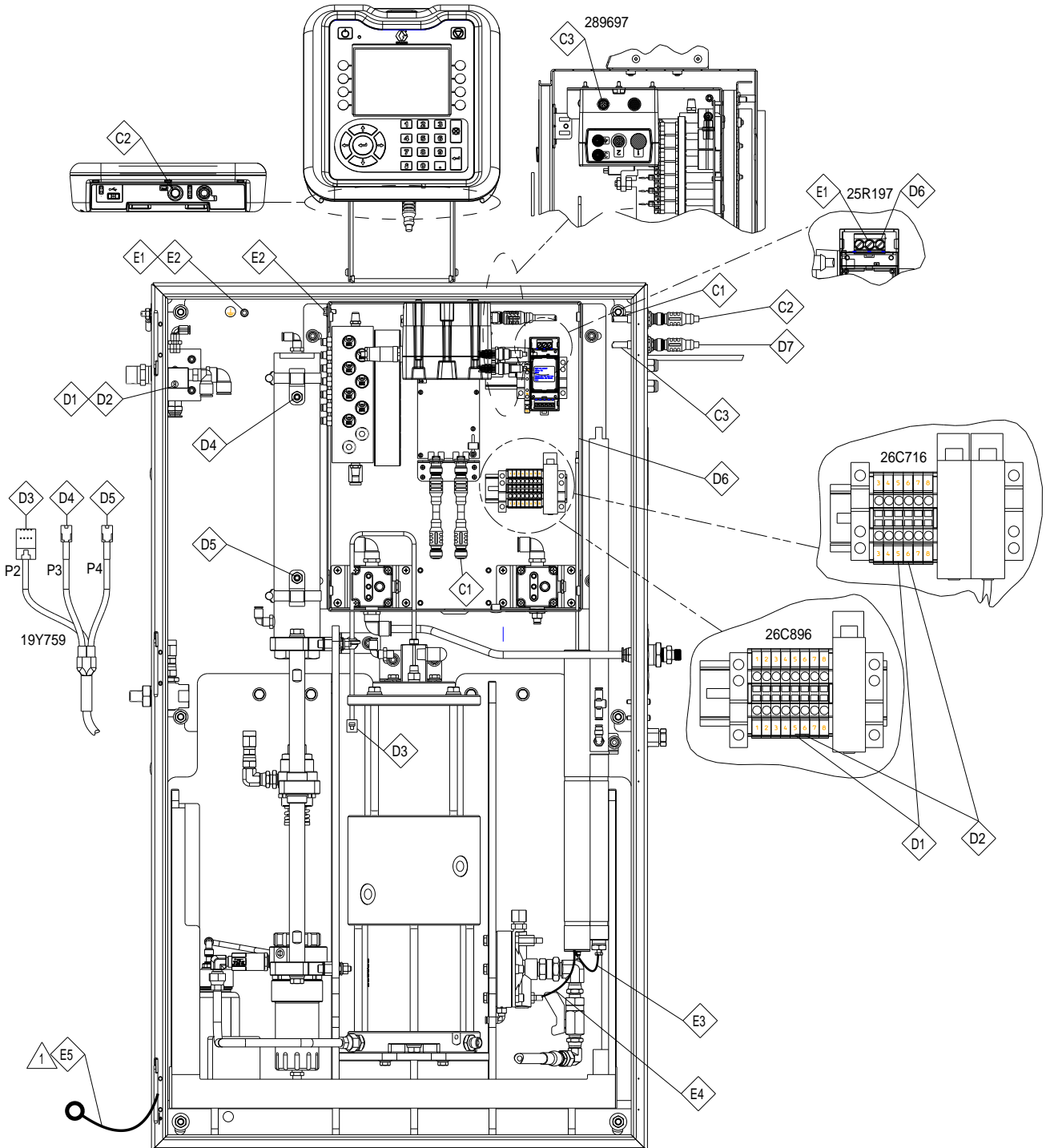
Figure 56 배선 연결
