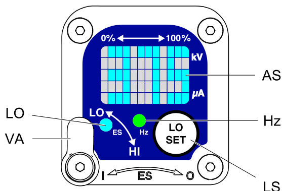
Figure 8 交流发电机速度 ( 赫兹 ) 屏幕
