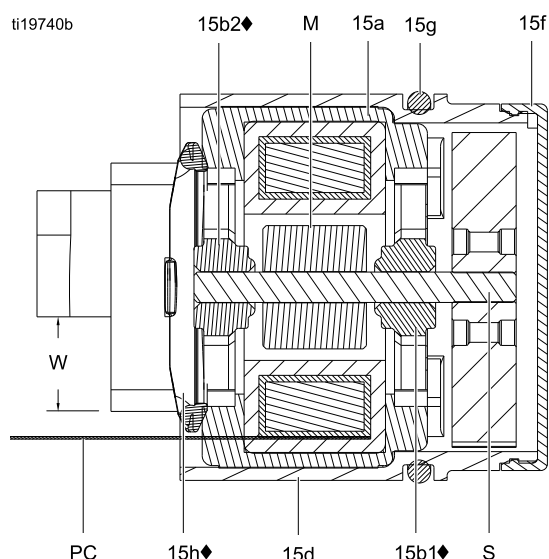
Figure 31 交流发电机横截面
