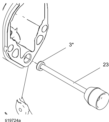
Figure 36 安装 U 形杯
