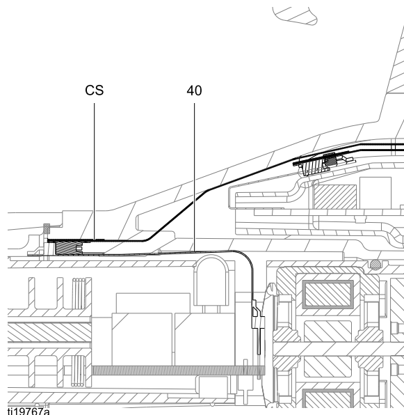
Figure 28 连接柔性电路
