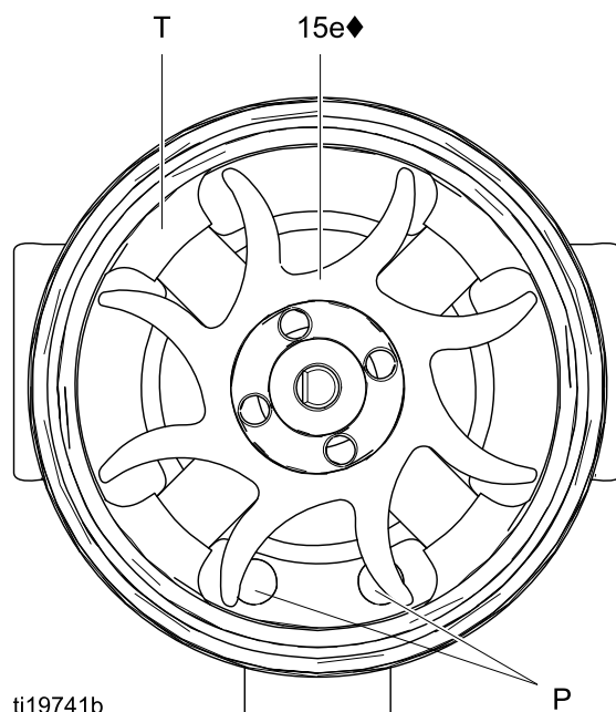
Figure 30 风扇方向
