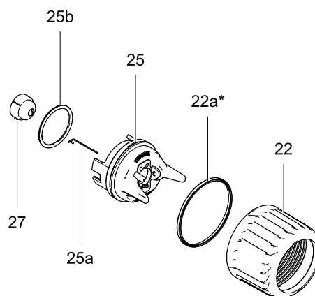
Figure 19 拆卸空气帽组件
