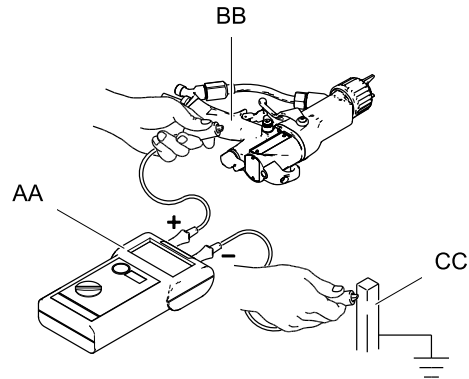
Figure 14 检查喷枪电气接地情况
