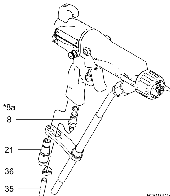
Figure 40 空气入口管接头和排气阀
