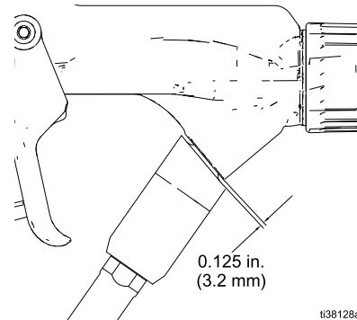
Figure 12 接头和枪筒的方向
