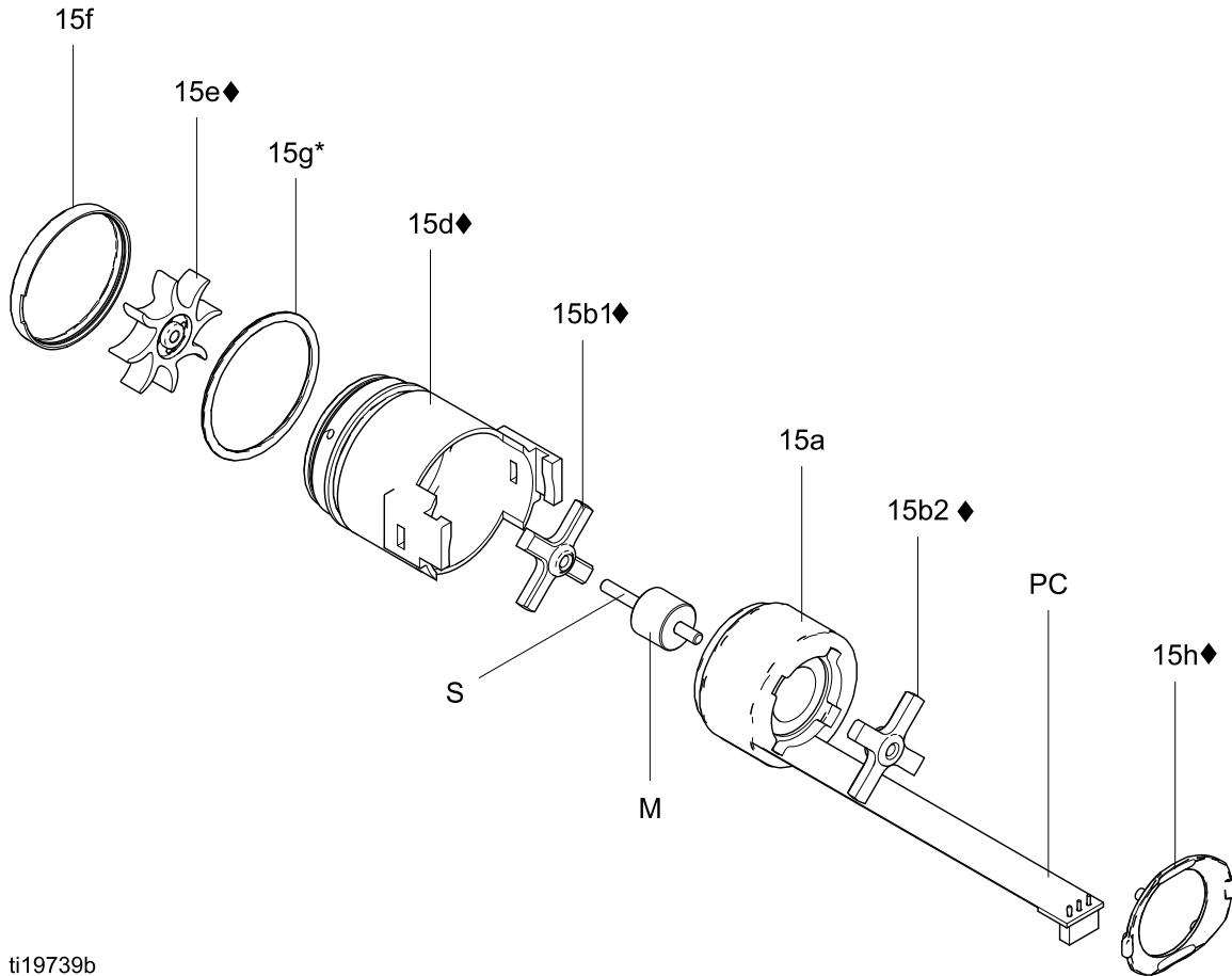
Figure 32 交流发电机
