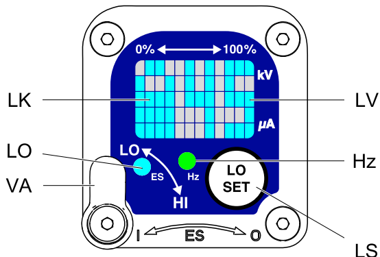
Figure 5 低压设置屏幕 (已锁定)。
