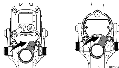
Figure 13 静电喷枪控制器
