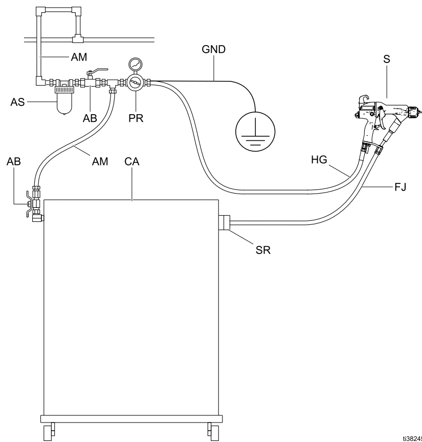
Figure 10 典型安装，Pro Xp 空气辅助式水性系统
