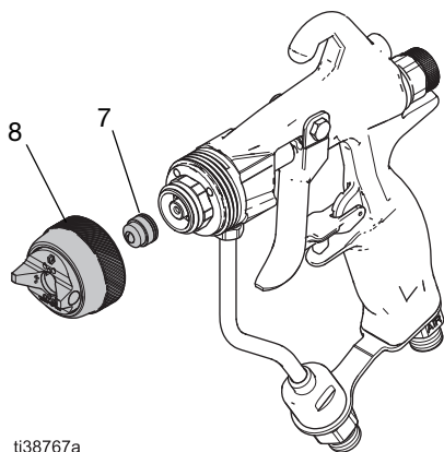
FIG. 26 : Retirez l'ensemble de chapeau d'air et la buse de pulvérisation
