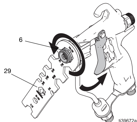
FIG. 50 : Retirez la cartouche de fluide
