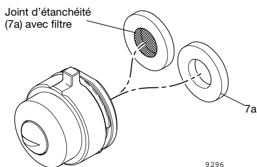
FIG. 56 : Options de joint d'étanchéité de buse de pulvérisation
