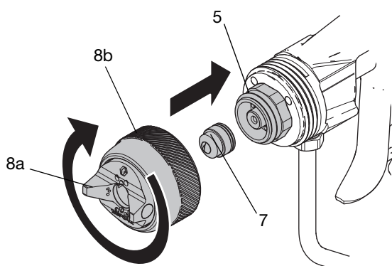
FIG. 40 : Remontez la buse de pulvérisation et le chapeau d'air
