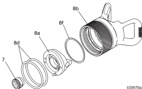
FIG. 45 : Pièces et buse de pulvérisation de l'ensemble de chapeau d'air PerformAA 50
