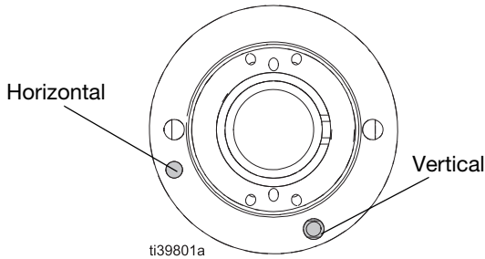
FIG. 10 : Positions de la goupille d'alignement du chapeau d'air
