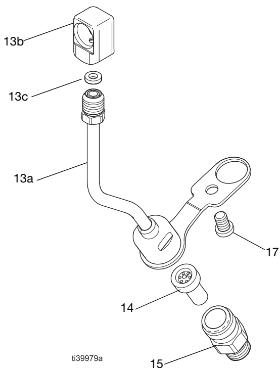
FIG. 57 : Ensemble de tuyau de fluide : modèle 26B711
