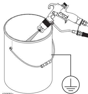
FIG. 27 : Rincez le pistolet
