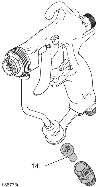
FIG. 31 : Vérifiez le filtre à fluide en ligne
