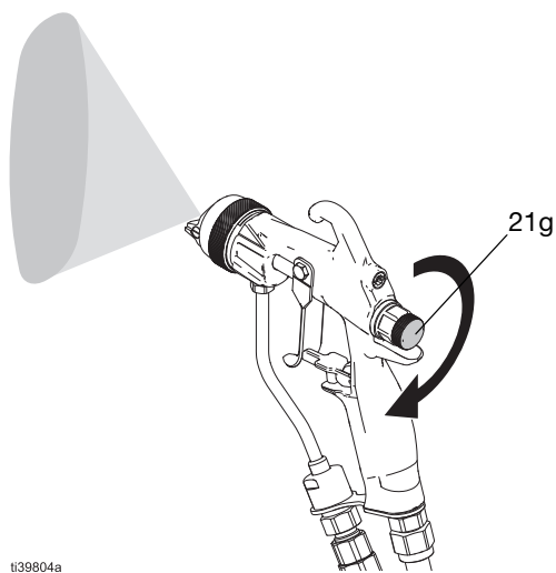
FIG. 23 : Largeur de jet large
