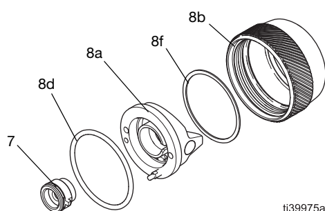
FIG. 46 : Pièces et buse de pulvérisation de l'ensemble de chapeau d'air PerformAA 15
