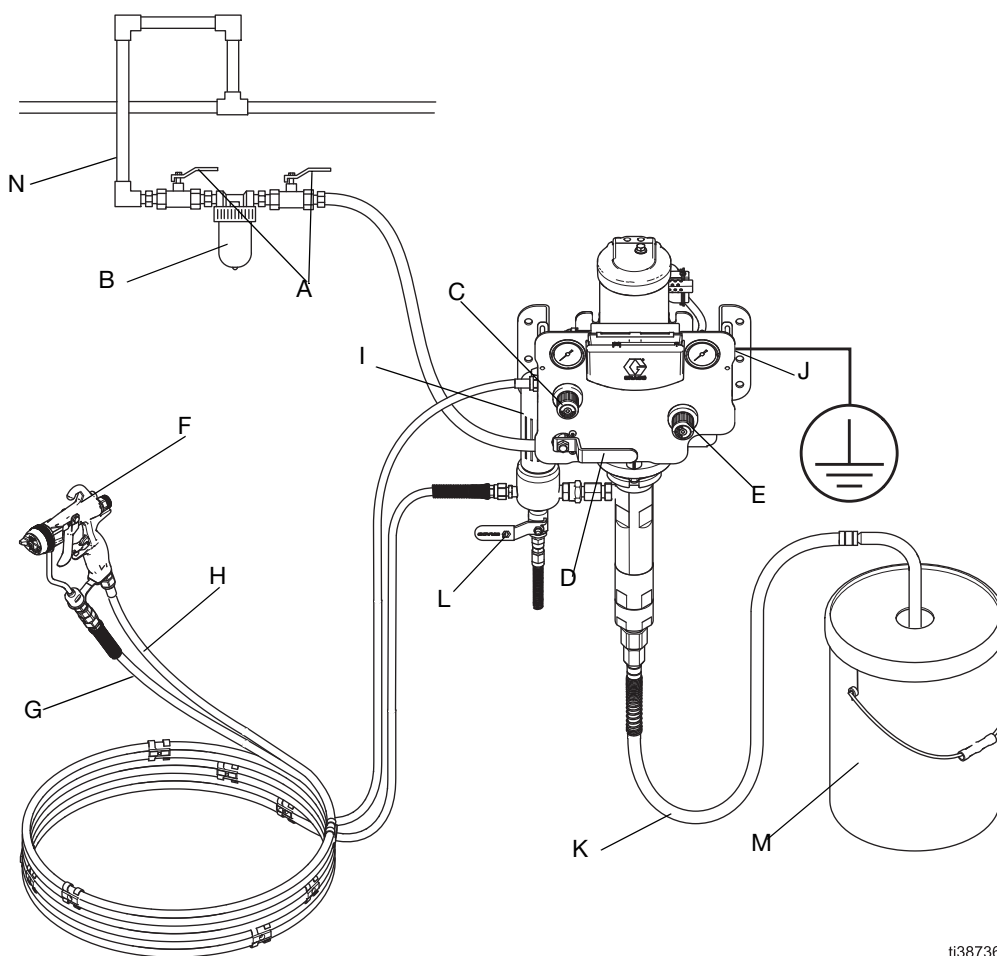
FIG. 3 : Installation type (PerformAA 15 modèle 26B501 représenté)
