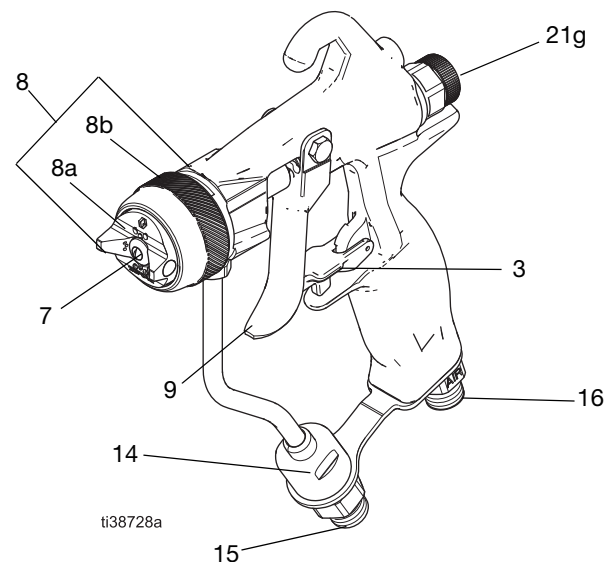
FIG. 1 : PerformAA 50 avec raccord tournant de fluide
