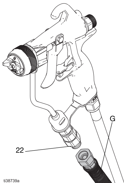
FIG. 6 : Raccordement du flexible d'alimentation en fluide du pistolet
