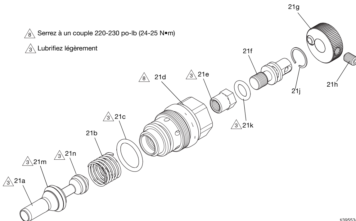
FIG. 48 : Ensemble de cartouche d'air (pour modèles air assistés)
