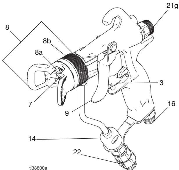
FIG. 1 : PerformAA 50 avec raccord tournant de fluide
