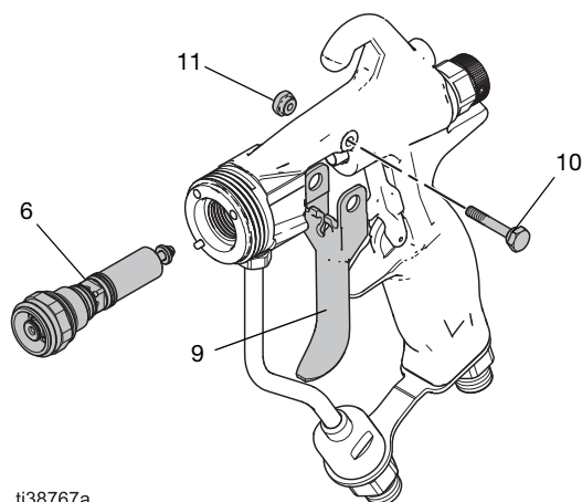
Fig. 51 : Retirez la gâchette pour libérer la cartouche de fluide
