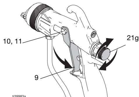
FIG. 41 : Vérifiez la gâchette et le bouton de réglage du ventilateur
