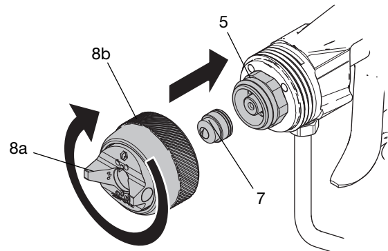
FIG. 8 : Installation du chapeau d'air et du circlip
