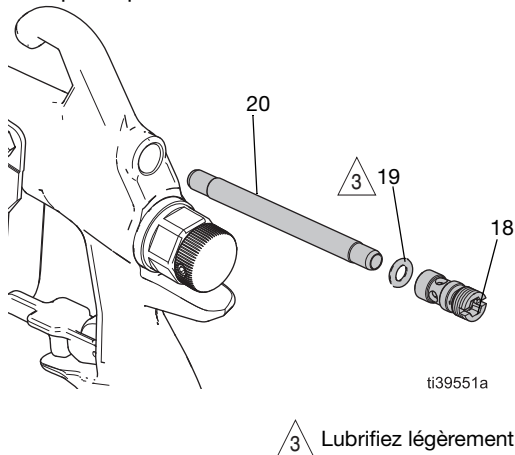
FIG. 49 : Ensemble de tuyau du ventilateur
