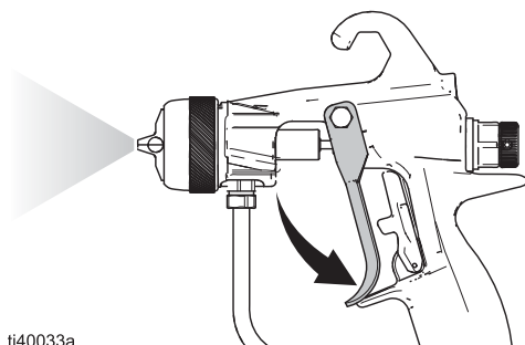
FIG. 19 : Vérifiez la forme de jet
