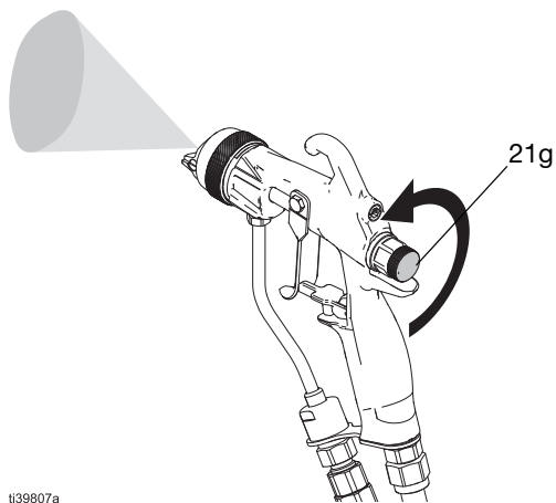
FIG. 22 : Largeur de jet étroit
