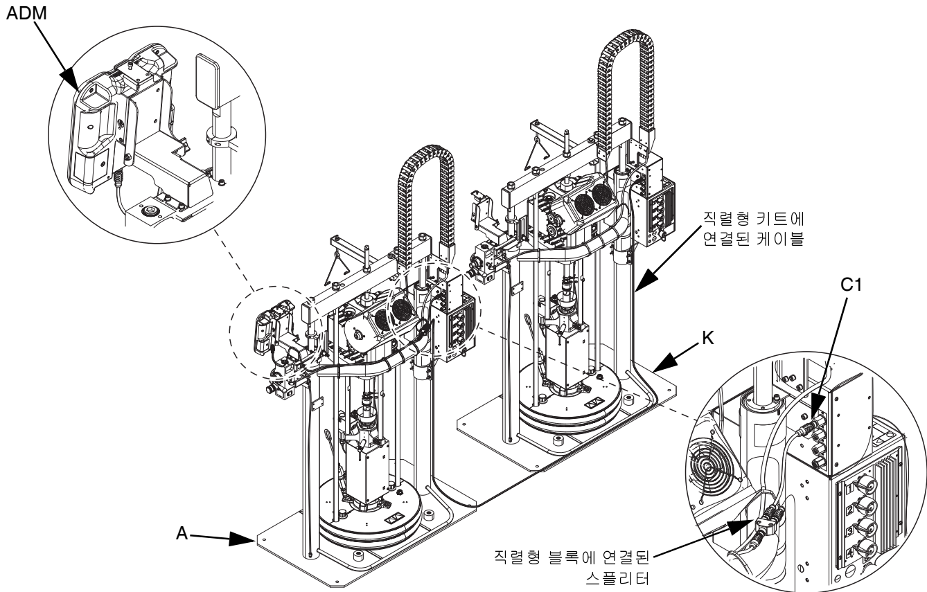
그림 10: 통신 연결
