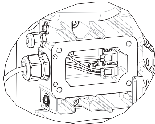
그림 38: 드라이버 하우징 내 와이어
