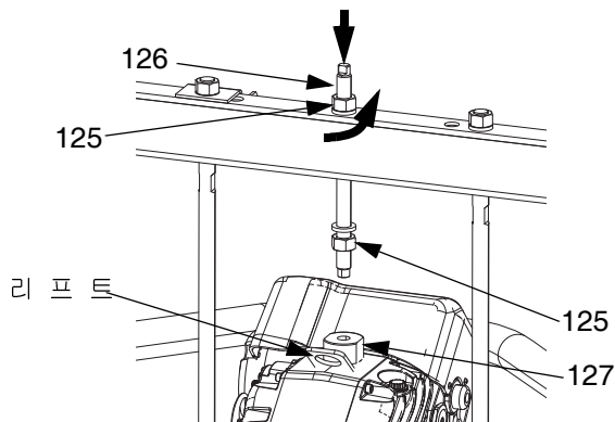
그림 41: 55 갤런 플레이트
