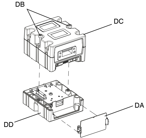
그림 52: CGM 분해
