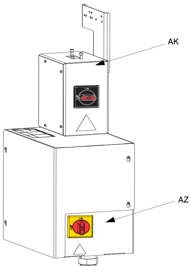
그림 4: 전원 차단
