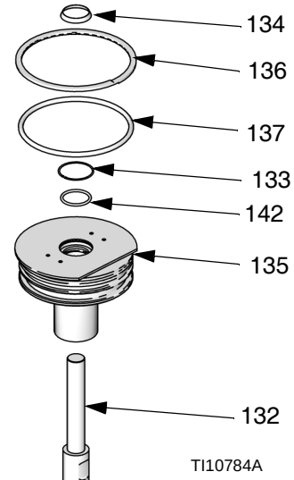
그림 43: 6.5 in 피스톤 로드 쉘
