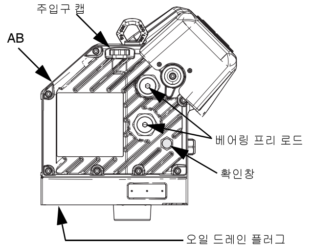
그림 32: : 확인창 및 오일 주입 캡
