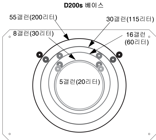
그림 15: 램 베이스
