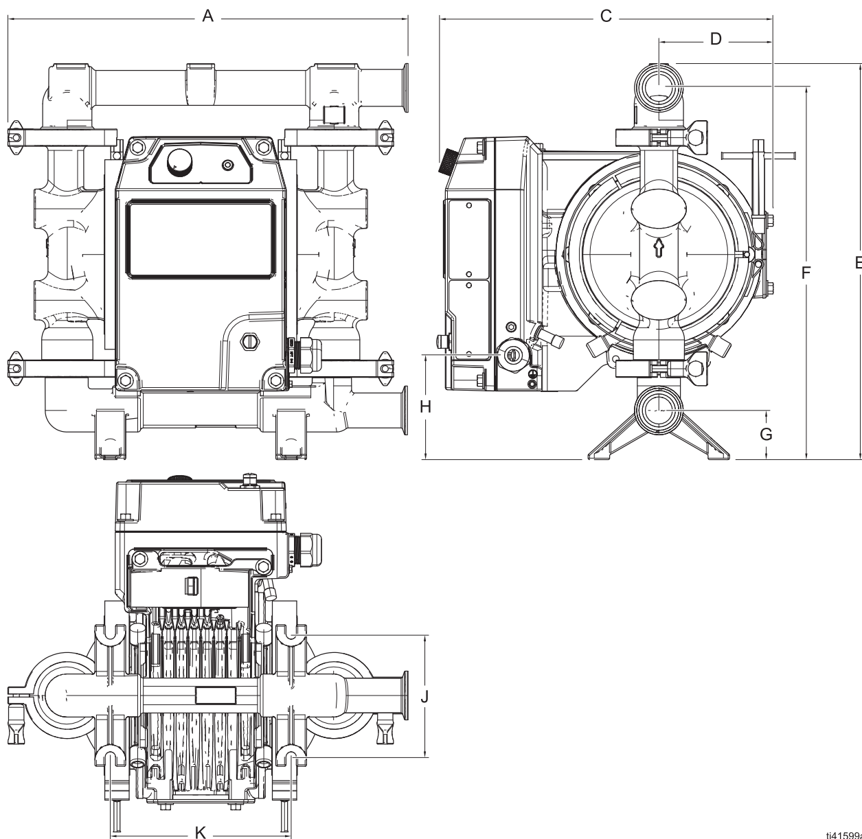
ABB. 22: h30 (QHC) Abmessungen hygienisches Modell (FG-Modell abgebildet)
