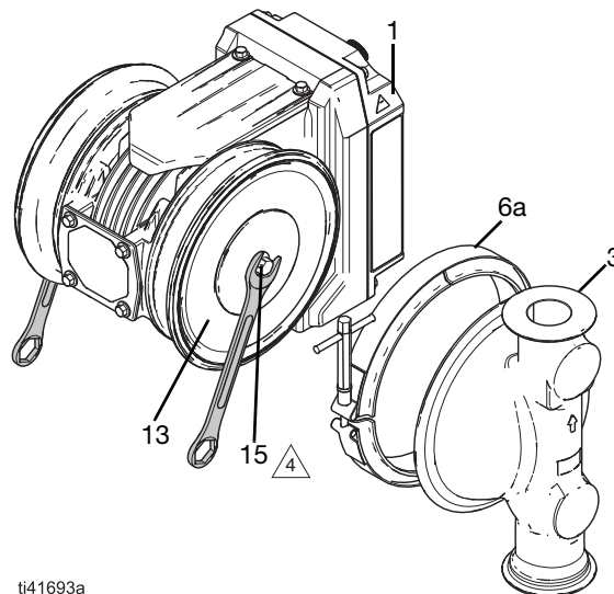
ABB. 18: Standard-Membranen festziehen
