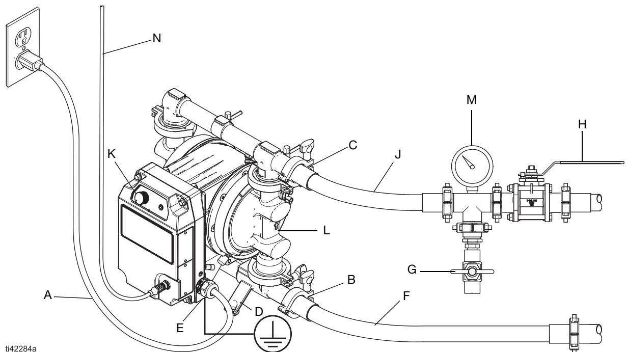
ABB. 3: Typische Installation für Modelle an gewöhnlichen Standorten (Kabel- und Steckeranschluss) (Modell h30 (QHC) abgebildet)
