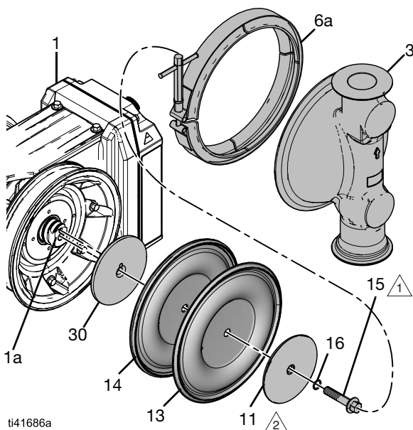
ABB. 17: Zusammenbau der Standard-Membranen (die Abbildung zeigt das hygienische Modell)
