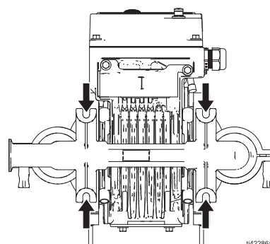
ABB. 5: Montagebohrungen
