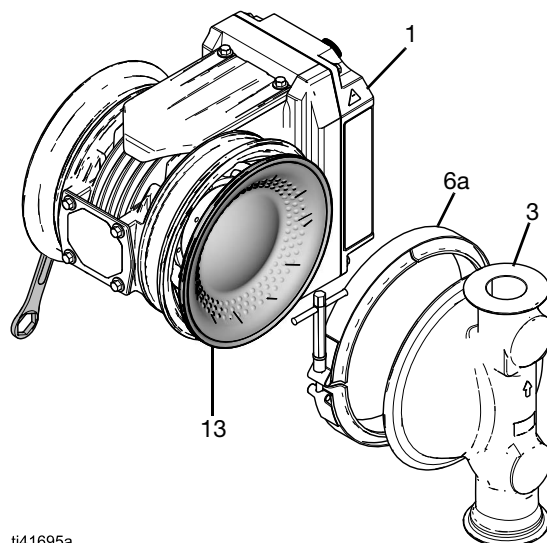
ABB. 21: Einbau – umgossene Membranen
