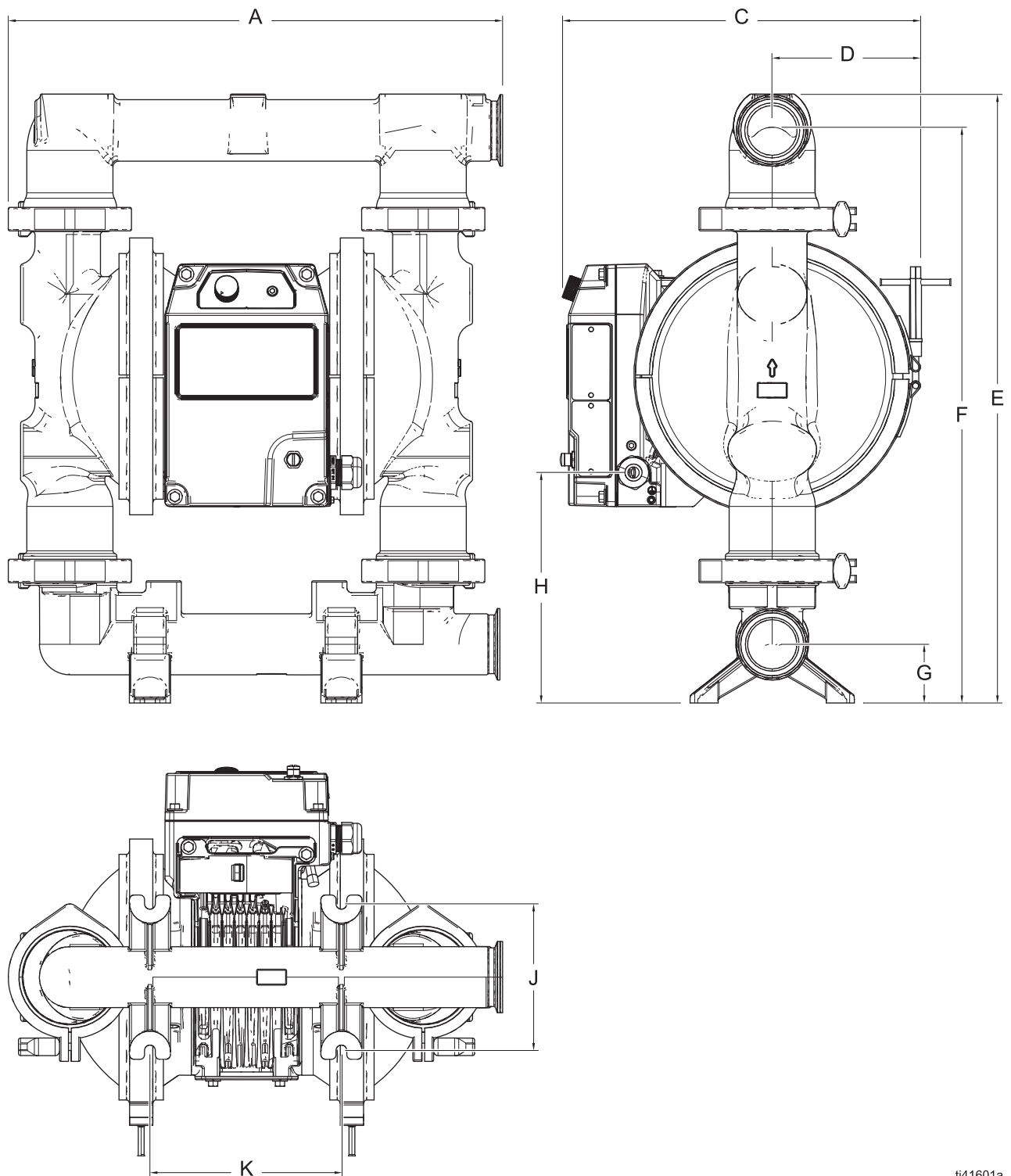
ABB. 26: h120 (QHE) Modell Abmessungen (FG-Modell abgebildet)
