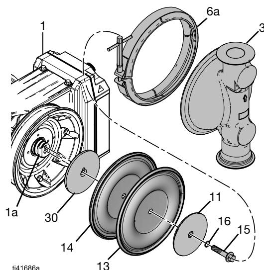
ABB. 16: Standard-Membranen
