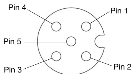
ABB. 11: M12, 5-poliger Stecker für Modelle an gewöhnlichen Standorten
