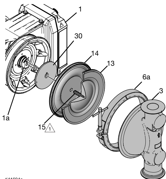
ABB. 20: Einbau – umgossene Membranen
