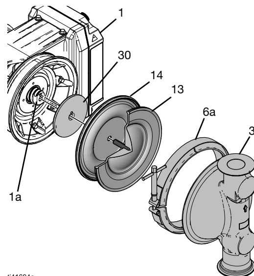
ABB. 19: Umgossene Membranen
