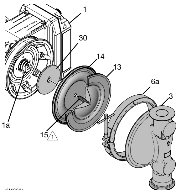
FIG. 20: Montere overstøpte membraner
