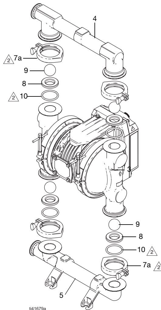
FIG. 15: Tilbakeslagsventiler
