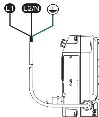
FIG. 9: Kobling for enkelfase-modeller
