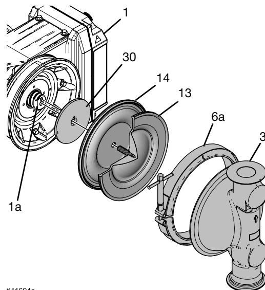
FIG. 19: Overstøpte membraner
