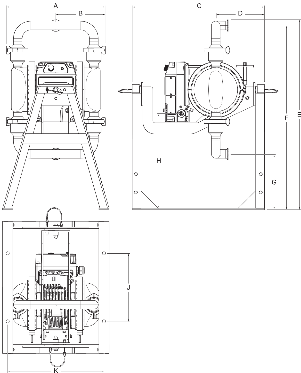
FIG. 25: h80-modell (QHD) dimensjoner (HS-modell vist)
