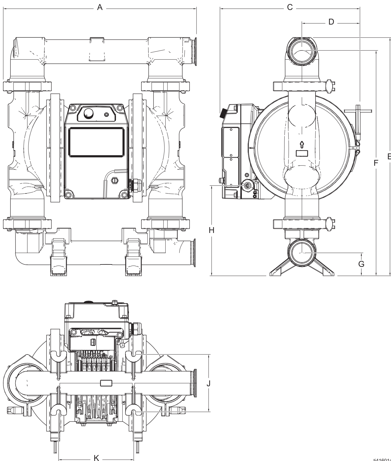
FIG. 26: h120-modell (QHE) dimensjoner (FG-modell vist)
