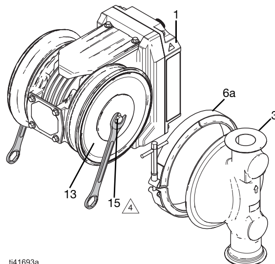
FIG. 18: Stramme standardmembraner
