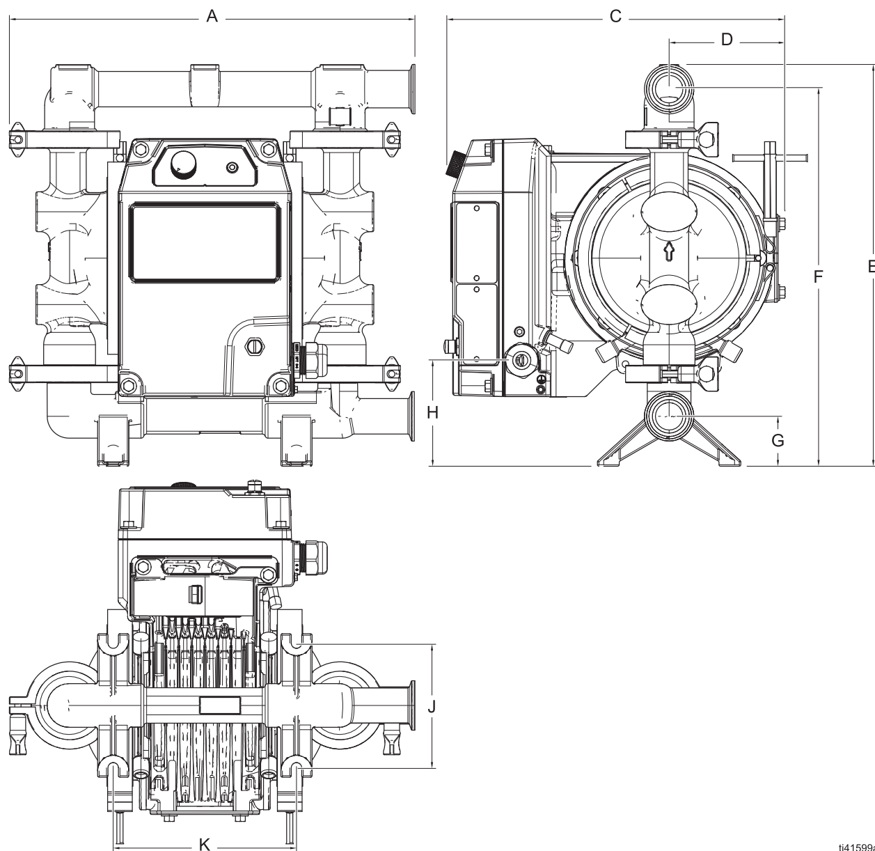
FIG. 22: h30 (QHC) hygienisk modell dimensjoner (FG-modell vist)
