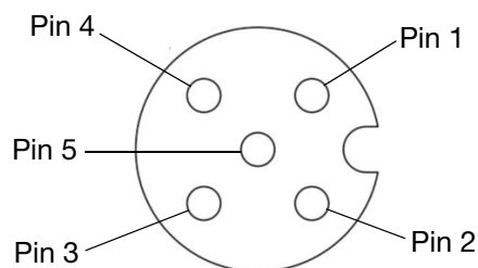
FIG. 11: M-12, 5-pinne tilkobling for modeller i ordinære områder
