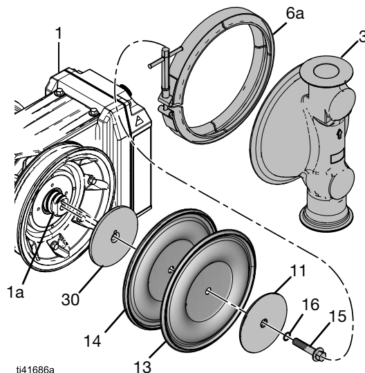
FIG. 16: Standardmembraner
