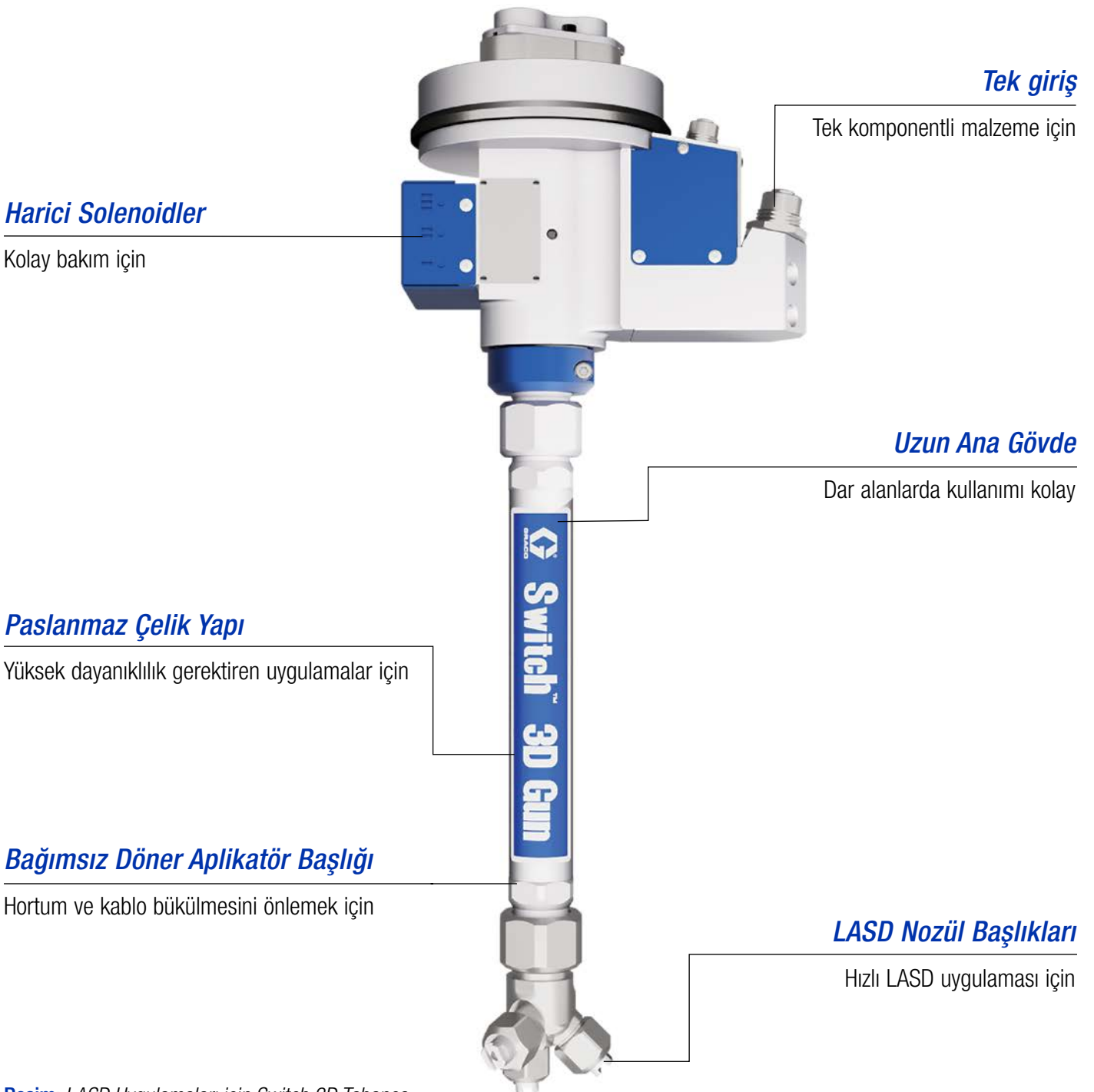
Resim: LASD Uygulamaları için Switch 3D Tabanca
