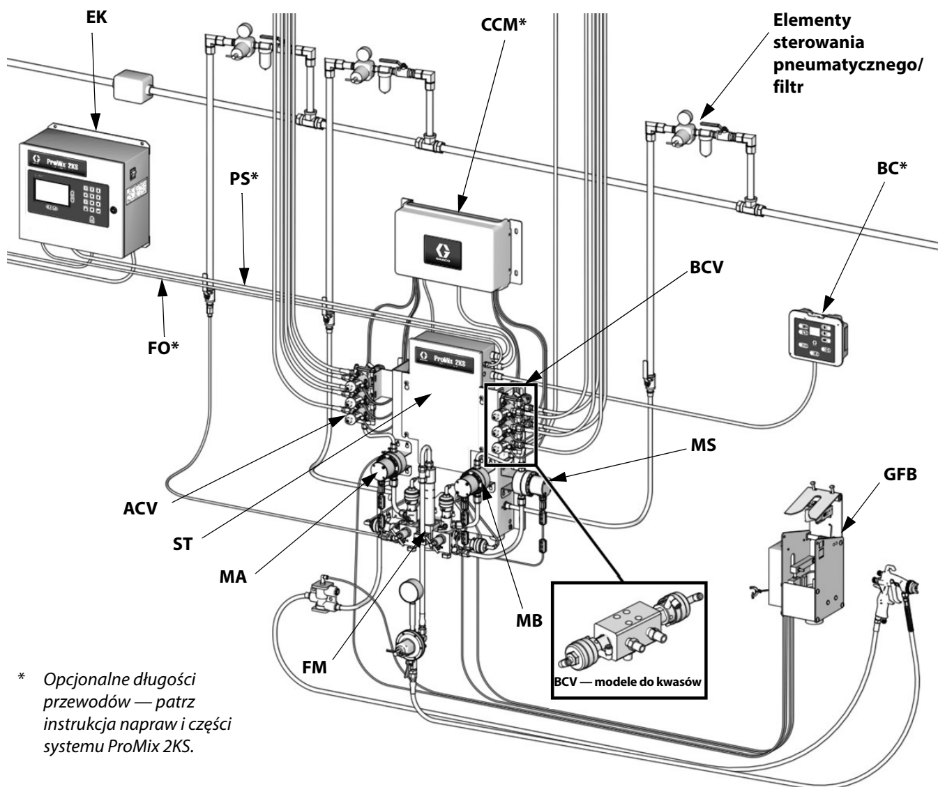
Rys. 2. System ręczny; wyposażony w mierniki G3000, zespół zaworów zmiany koloru/katalizatora, skrzynkę do przepłukiwania pistoletu i przepływomierz rozpuszczalnika
