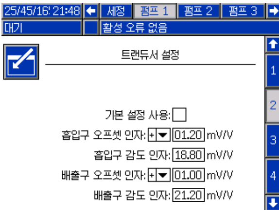
Figure 65 펌프 화면 2, 기본 설정 비활성화됨
