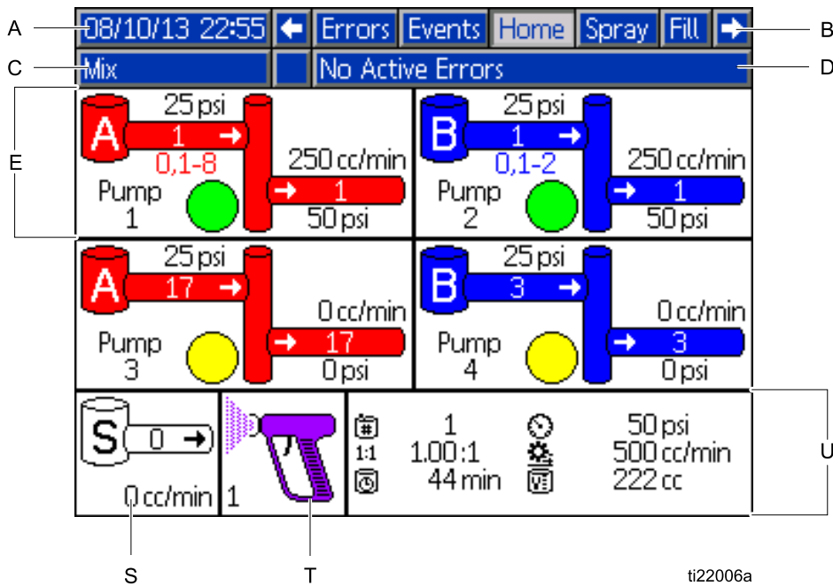
Figure 15 홈 화면, 진단을 컨 혼합 모드
