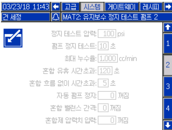
Figure 34 혼합 모드의 시스템 화면 2
