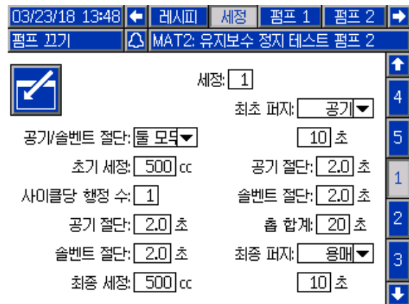
Figure 63 에어/솔벤트 절단이 모두 포함된 세척 화면
