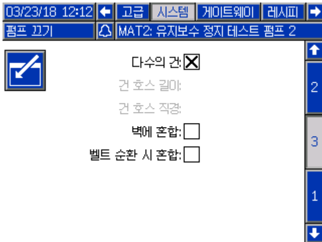
Figure 36 시스템 화면 3 다중 건
