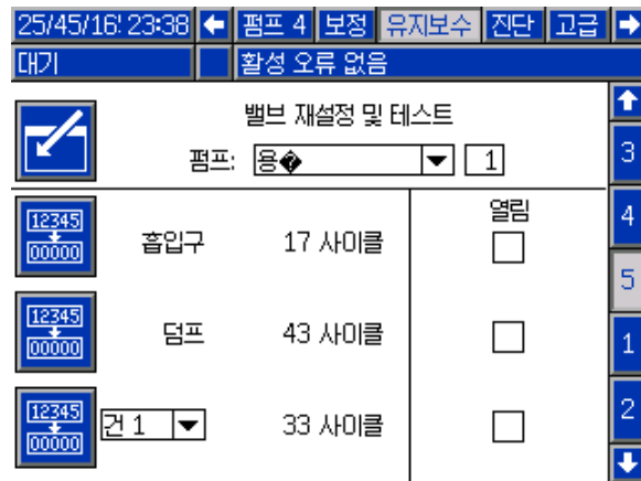
Figure 80 유지보수 화면 5, 용제 밸브 재설정
