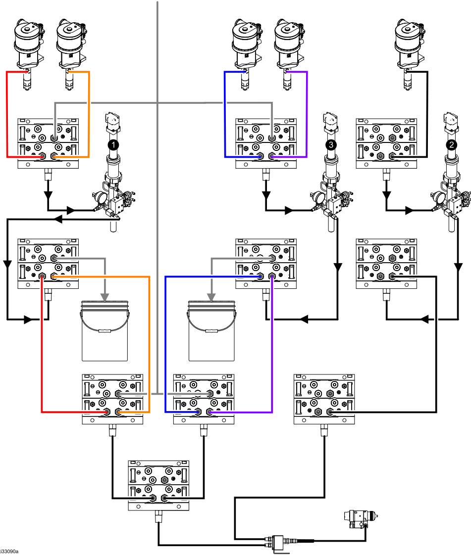
Figure 57 보조 밸브의 적용 예
