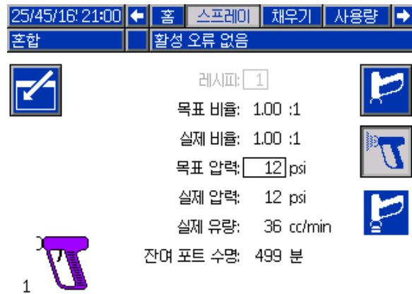
Figure 17 혼합 모드의 스프레이 화면
