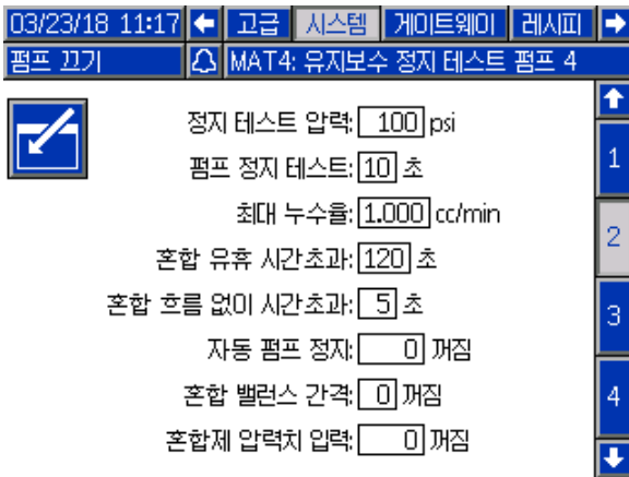
Figure 33 대기 모드의 시스템 화면 2
