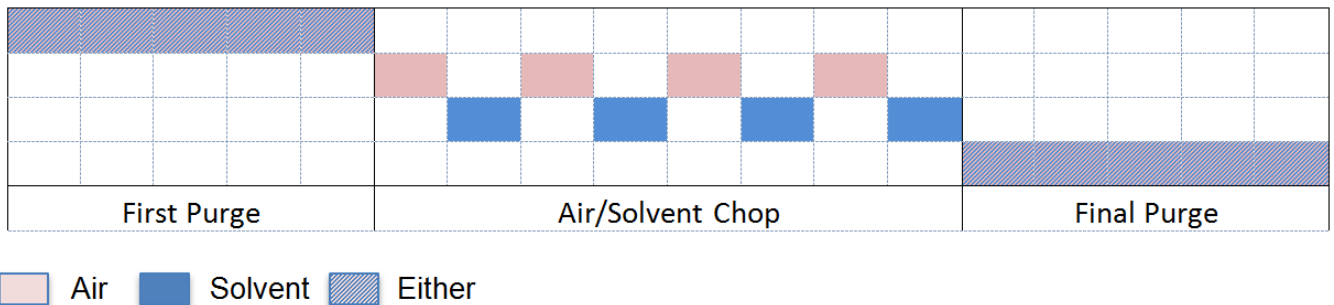
Figure 53 공기/솔벤트 절단 시간표
