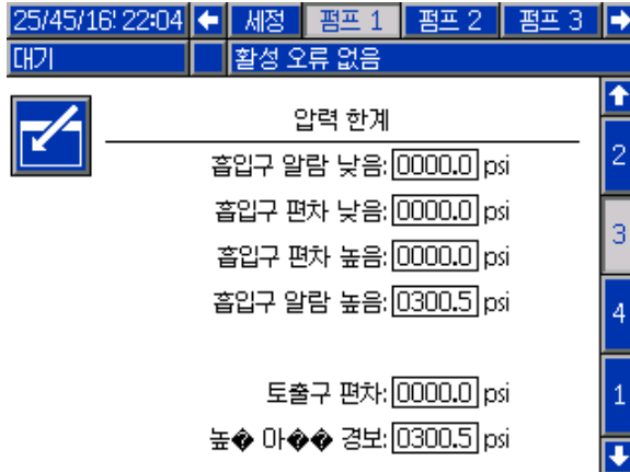
Figure 67 펌프 화면 3, 압력 모니터링 활성화됨
