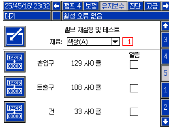
Figure 79 유지보수 화면 5, 색 밸브 재설정
