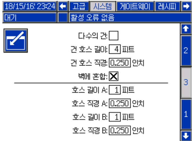
Figure 37 시스템 화면 3. 벽면 혼합(벽에서 혼합)
