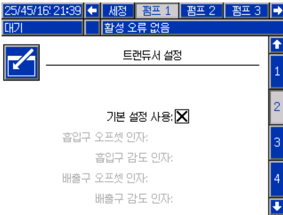
Figure 64 펌프 화면 2, 기본 설정 활성화됨
