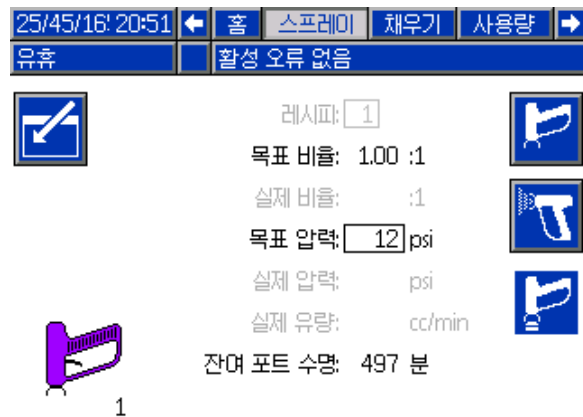
Figure 18 유휴 모드의 스프레이 화면
