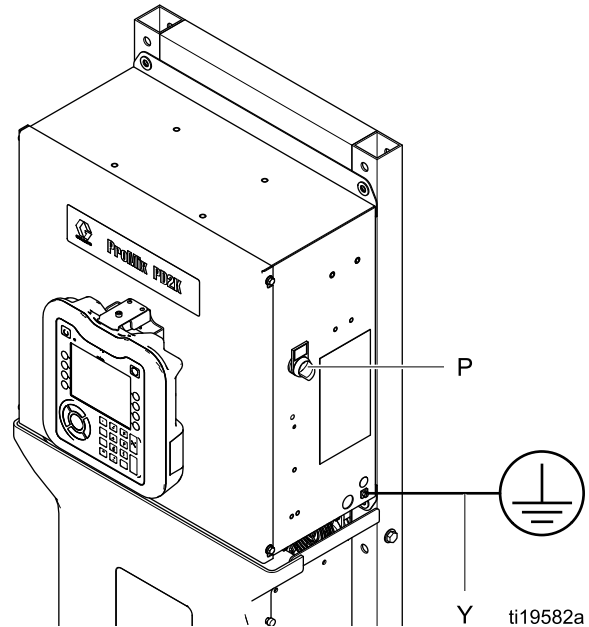
Figure 12 전원 스위치
