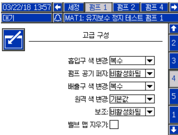
Figure 56 펌프 화면, 고급 구성
