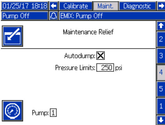
Figure 78 유지보수 화면 4, 수동 펌프 감압
