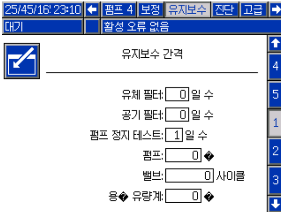
Figure 75 유지보수 화면 1, 간격 설정
