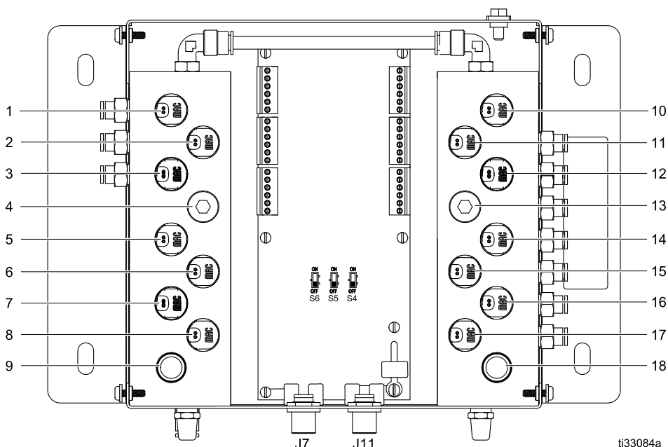
Figure 53 Numérotation d'emplacement d'électrovanne
