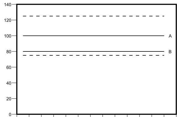
Figure 43 Plage de pression de sortie de la pompe côté B acceptable pour un système dont la pression de pulvérisation cible (A) est d'environ 7 bars (100 psi) et la tolérance de pression de mélange est de 25%.
