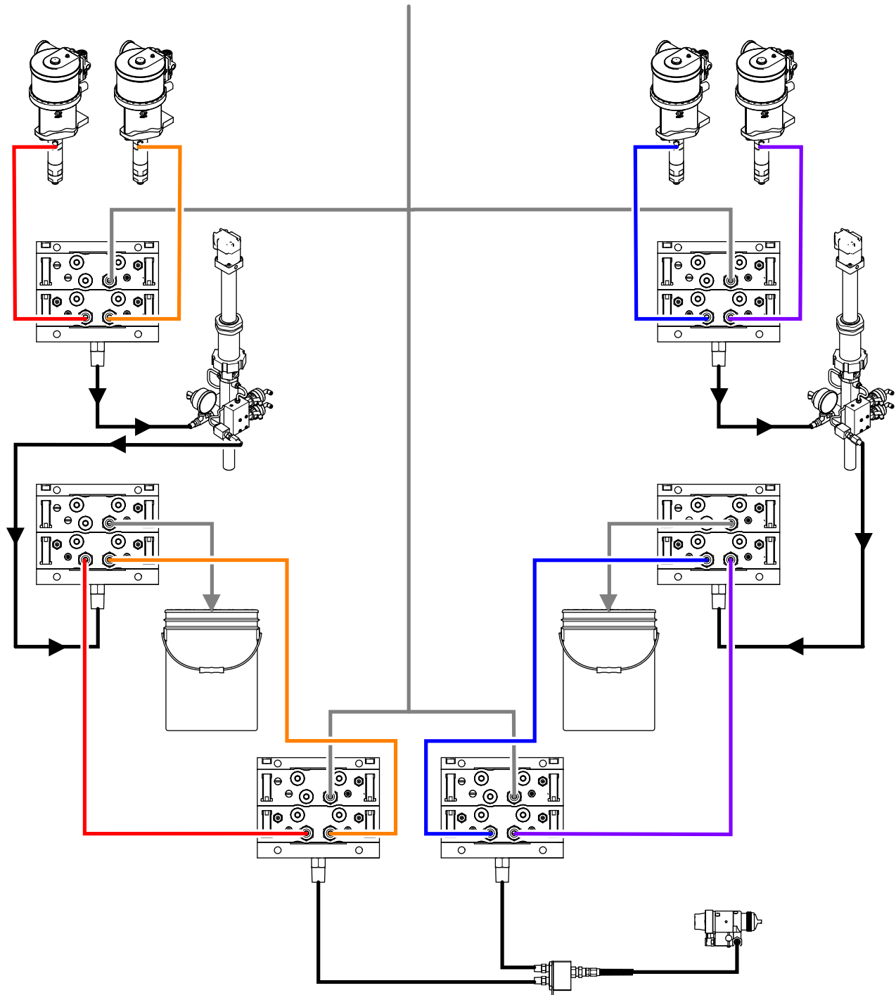
Figure 85 Conduites de produit pour un système PD2K automatique classique.
