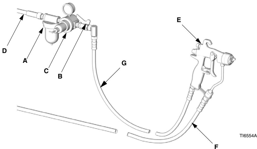
FIG. 1: voorbeeldinstallatie (afgebeeld model: G15)
