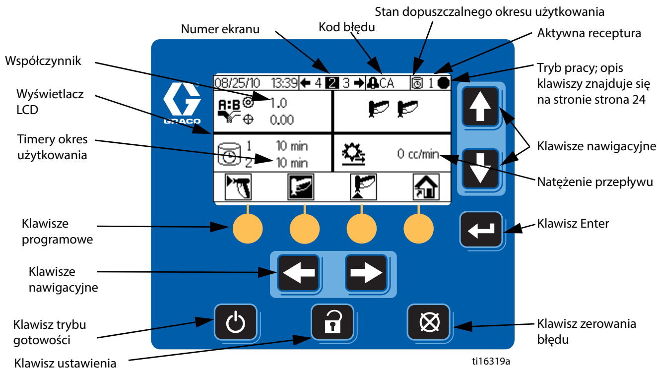
Rys. 10. Moduł wyświetlacza
