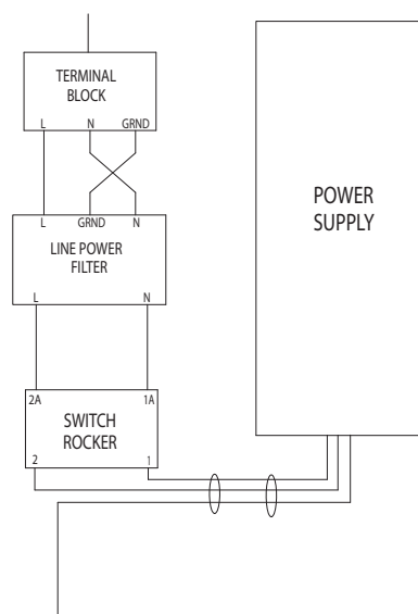
Rys. 7. Schemat elektryczny
