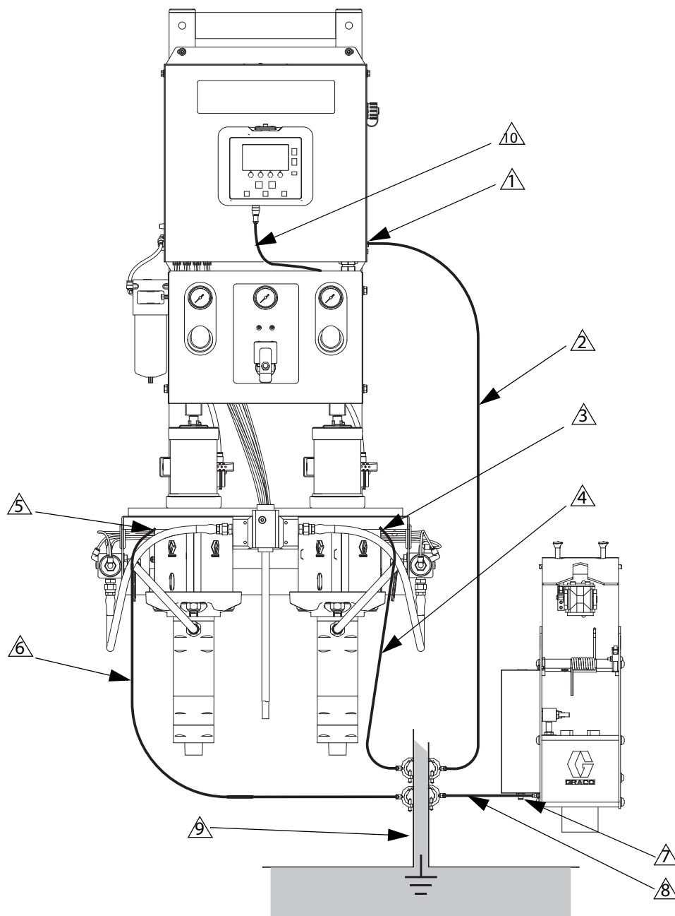
Rys. 9. Uziemienie
