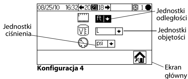
Rys. 39. Ekran Konfiguracja 3 (ekran 20) i Konfiguracja 4 (ekran 21)
