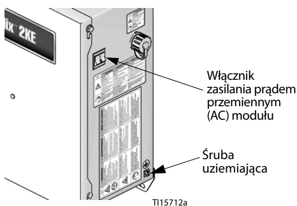
Rys. 8. Śruba uziemiająca i wyłącznik zasilania
