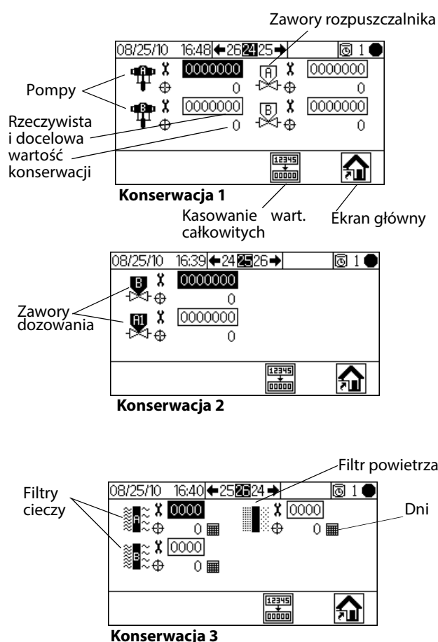
Rys. 42. Konfiguracja ekranu Konserwacja 1-3 (ekrany 24-26)
