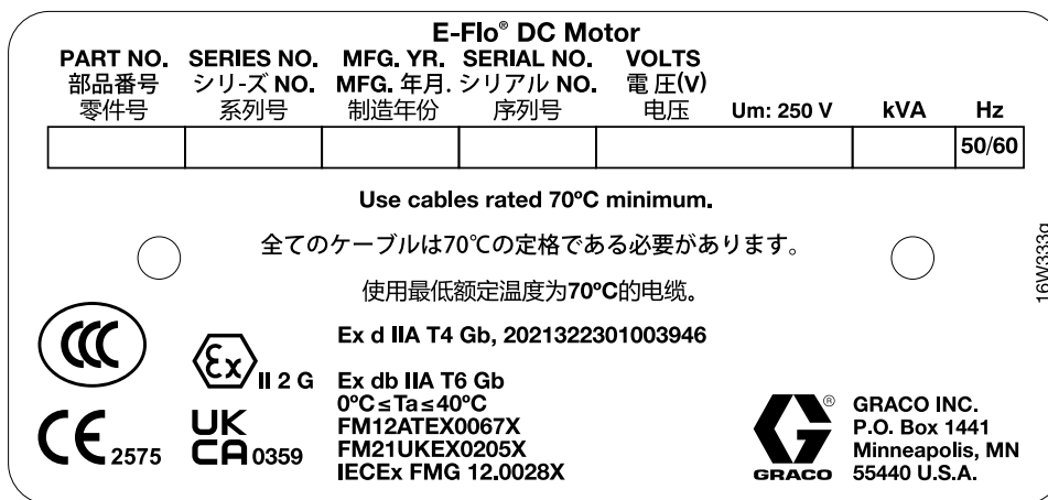
Figure 2 Identificatielabel basismotor met regio-specifieke goedkeuringen
