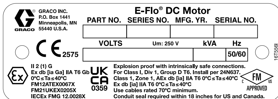
Figure 3 Identificatielabel geavanceerde motor
