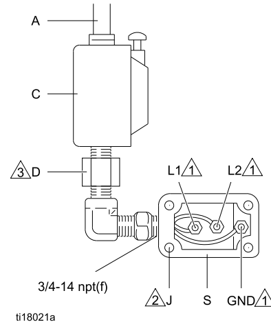
Figure 7 Collegare i fili dell'alimentazione
