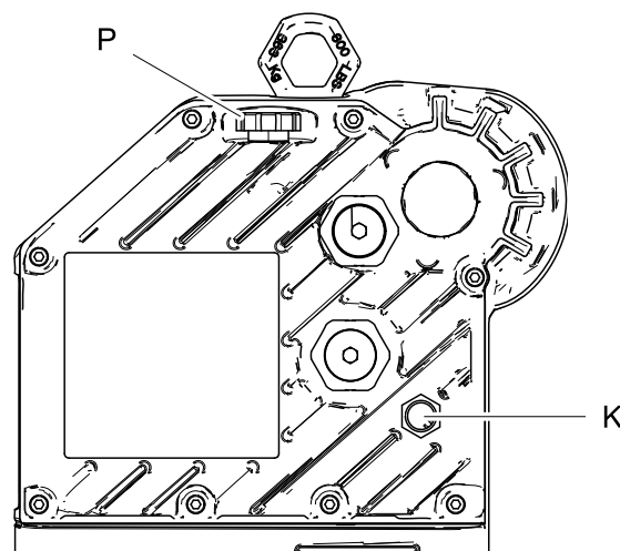
Figure 15 Finestra di ispezione e cappuccio di riempimento dell'olio
