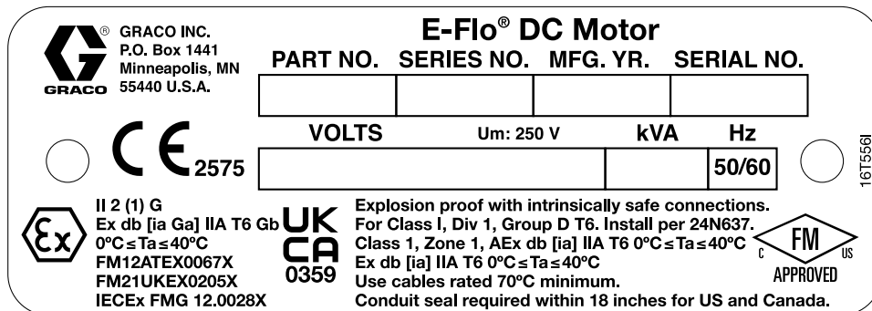
Figure 3 Etichetta identificativa del motore avanzato
