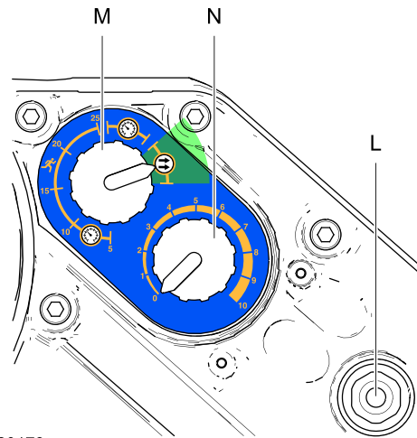
ti20173a Figure 13 Modalità Portata
