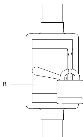
Figure 6 Zablokowany zabezpieczony bezpiecznikiem wyłącznik bezpieczeństwa
