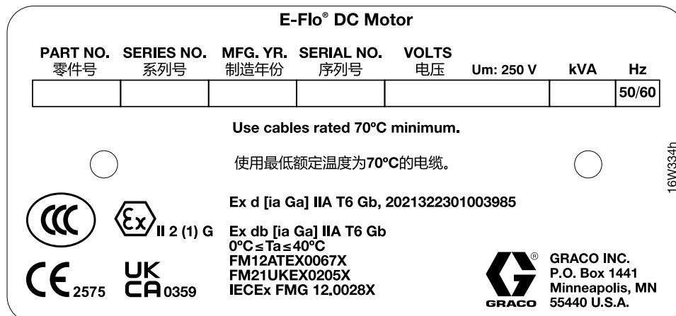
Figure 4 Zaawansowany silnik z naklejką identyfikacyjną zawierającą regionalne aprobaty
