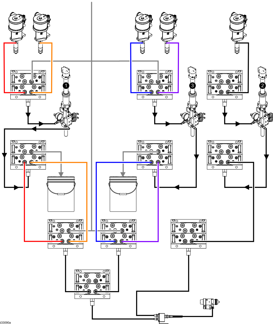
Figure 53 Aplicación de ejemplo de la válvula auxiliar
