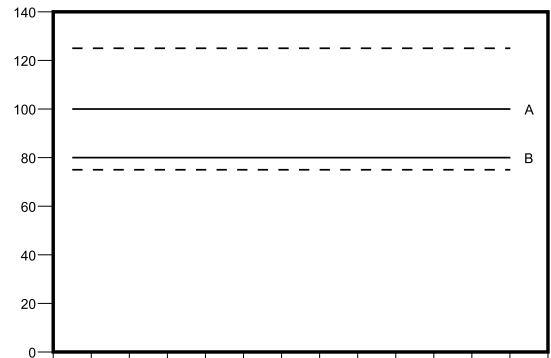
Figure 46 El rango de presión de salida aceptable de la bomba B para un sistema con un objetivo de presión de pulverización (A) de 100 psi y una tolerancia de presión de mezcla del 25 %.
