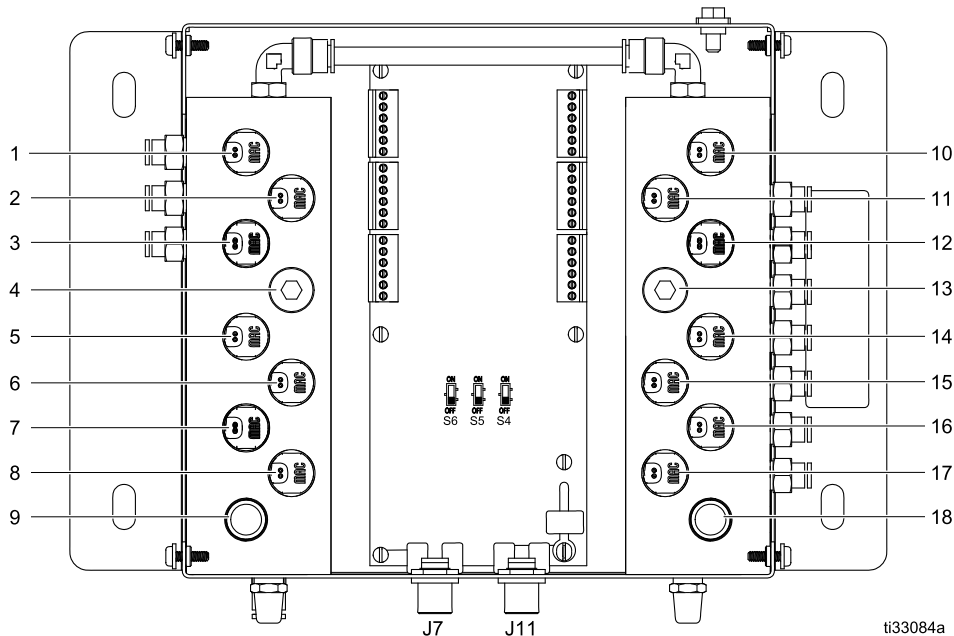
Figure 55 Enumeración de ubicación de solenoides
