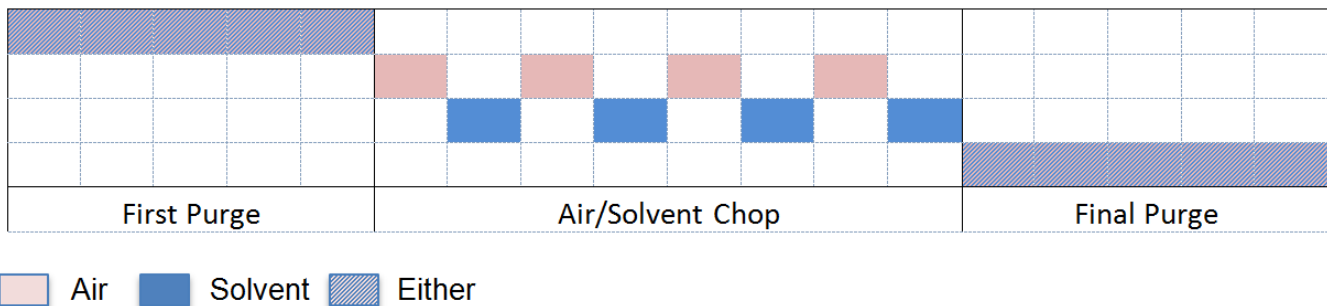
Figure 50 Diagrama de temporización de Corte aire/Solvente
