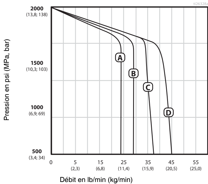
FIG. 78: Performances de la mousse GH-2 et GH-4
