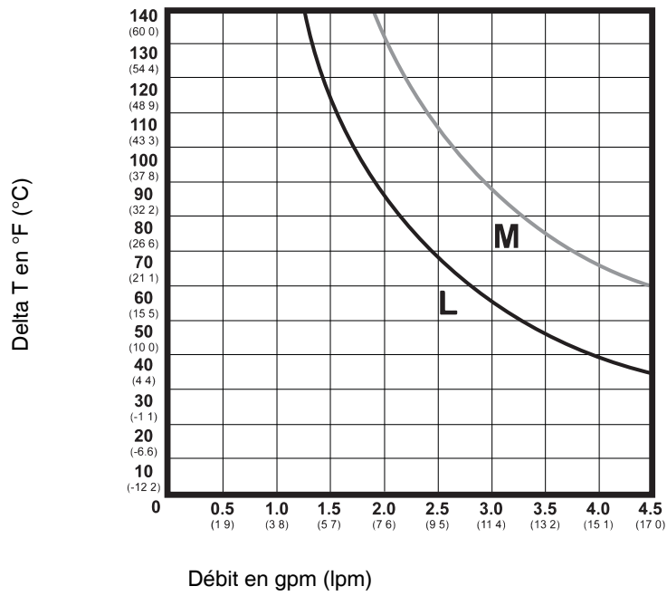
FIG. 79: Performances du réchauffeur
