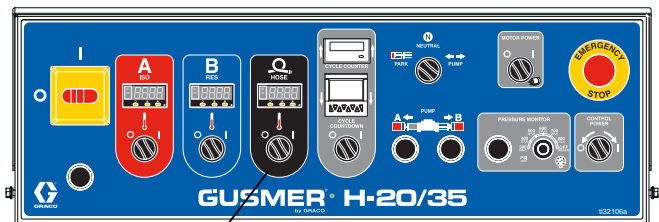
FIG. 24: Interrupteur de zone de chauffage pour flexible
